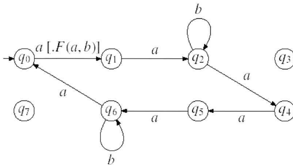
Figura 2.1 –Exemplo de autômato adaptativo que utiliza a notação exposta no tópico 2.1.3 (PISTORI,2003).
