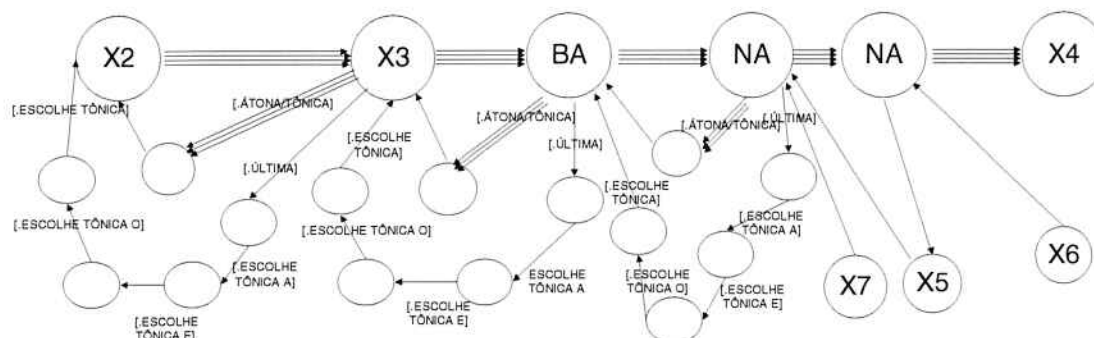
Figura 5.5 – Configuração do Transdutor após o desempenho da segunda sílaba NA da palavra banana .
