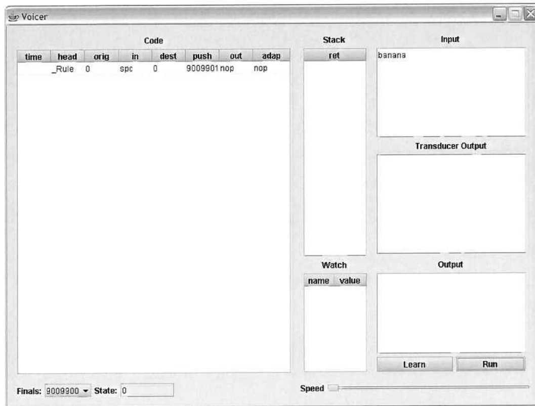
Figura 8.1 – Aparência Inicial do Voicer para a cadeia de entrada banana
