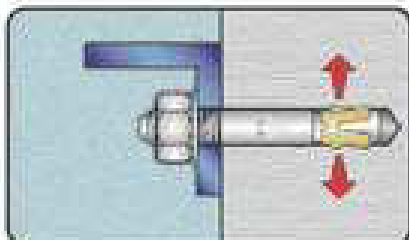
Figura 115: método de aplicação parabolit.
