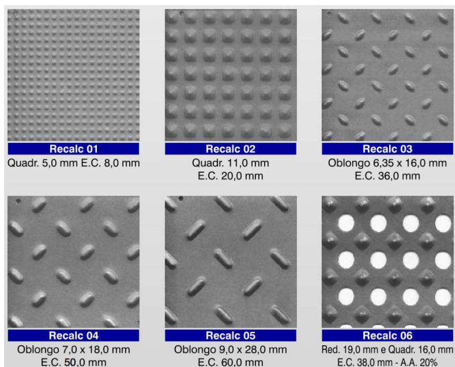
Figura 116: exemplo chapas recalçadas, catálogo Permetal.
