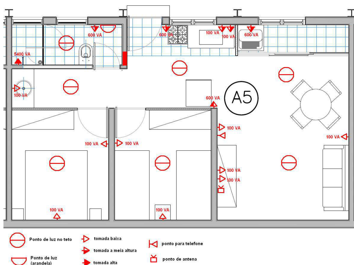
Figura 79 - exemplo de instalação elétrica em um apartamento.
