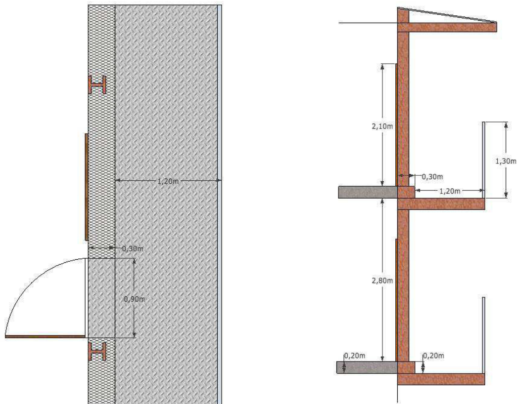
Figura 96: detalhe das passarelas: planta e corte, e degrau/relação com altura da janela do banheiro
