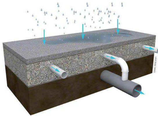
Figura 123 - Esquema do piso poroso. Fonte:
