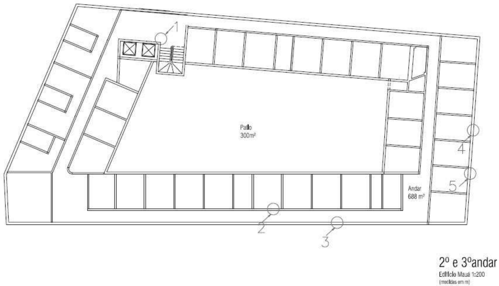
Figura 105: croqui dos pontos analisados pelo ensaio esclerométrico nos pavimentos.
