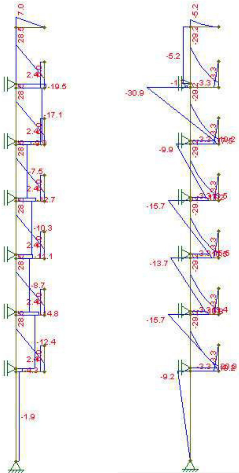
Diagramas da passarelas ( da esq para a dir.): cortante e fletor. Diagramas gerado pelo ftool.
