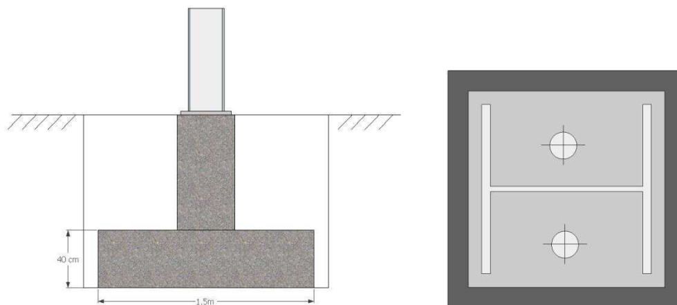
Figura 122: fundação da passarela
