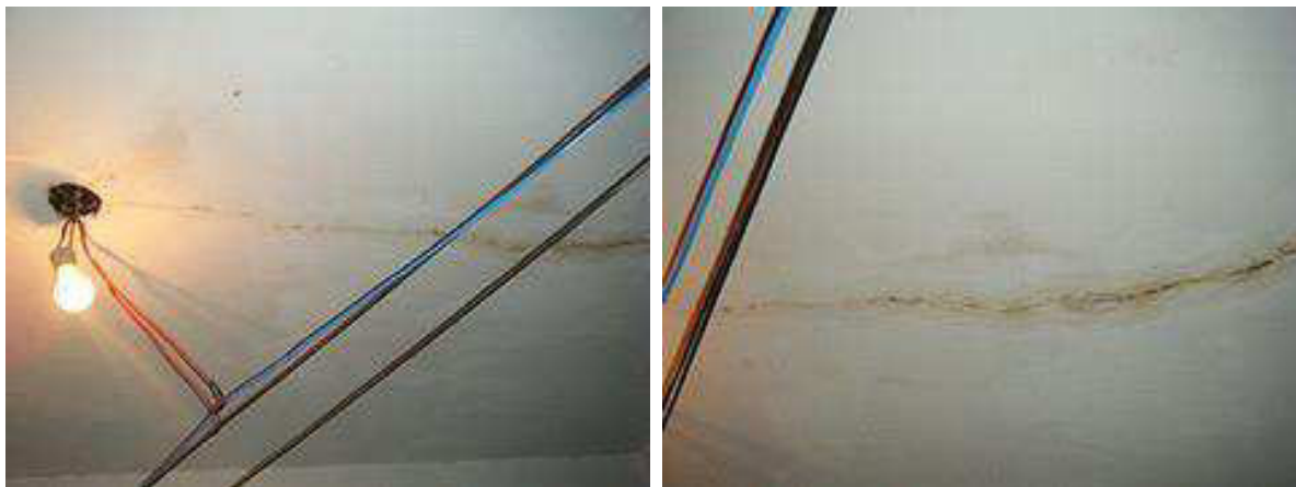
Figura 51: fissuras por corrosão de conduíte nas lajes do 4º andar. Fotos tiradas pelo grupo.
