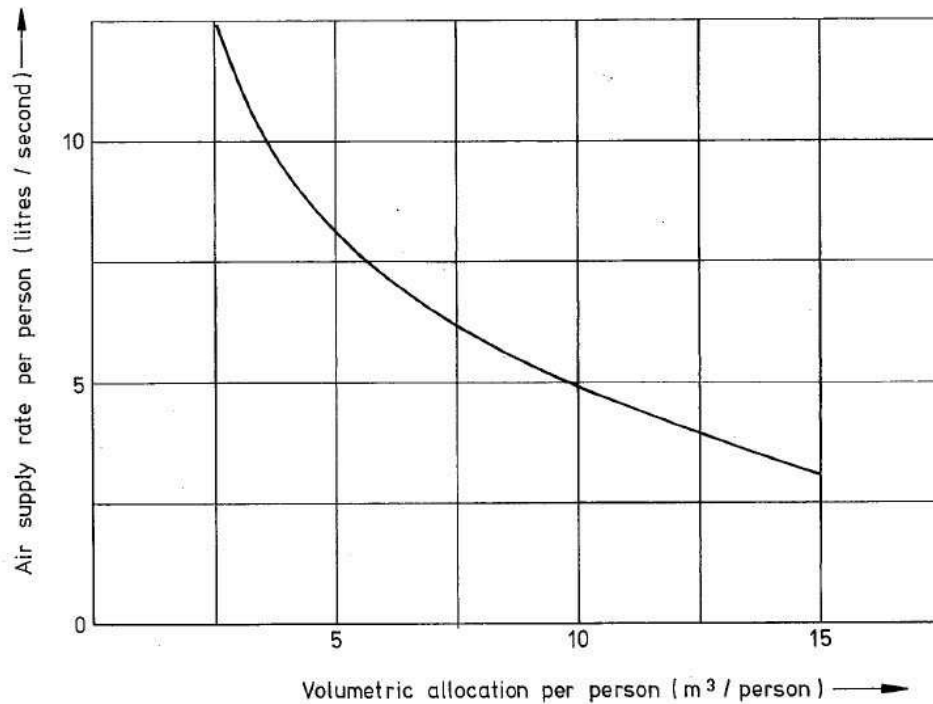
Gráfico 8: taxa de suprimento de ar para remoção de odores internos. Fonte: norma BS5925.
