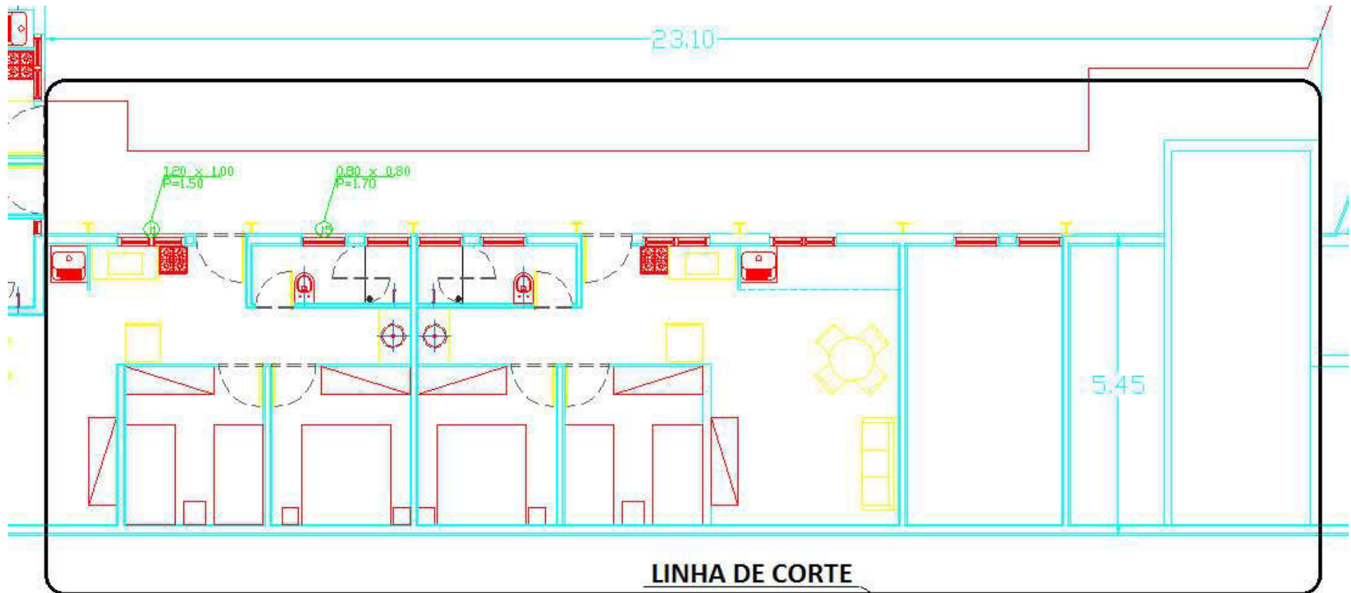
Figura 109: porção do pavimento-tipo do edifício Mauá modificado para o cálculo da ventilação.
