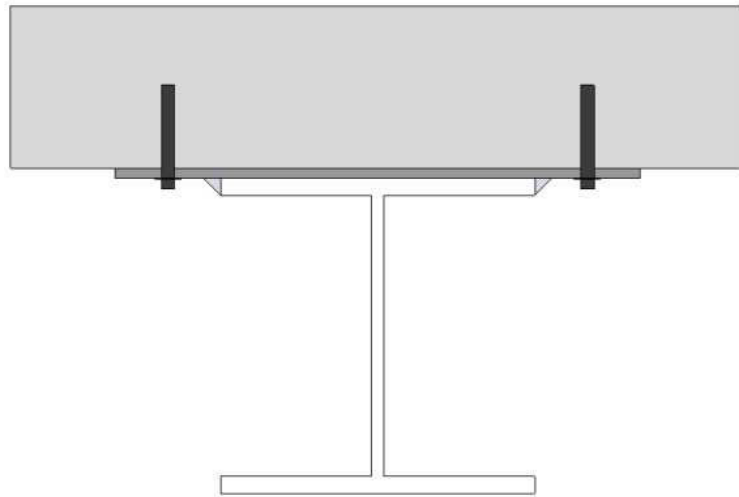
Figura 113: detalhe chumbamento - planta
