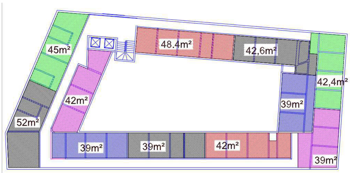
Figura 67: alternativa 1 de projeto para os pavimentos.
