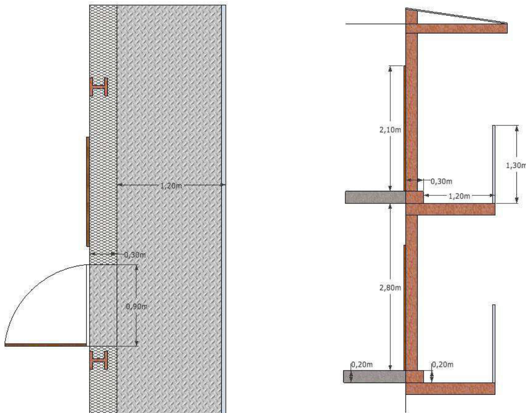
Figura 111: dimensões da passarela.
