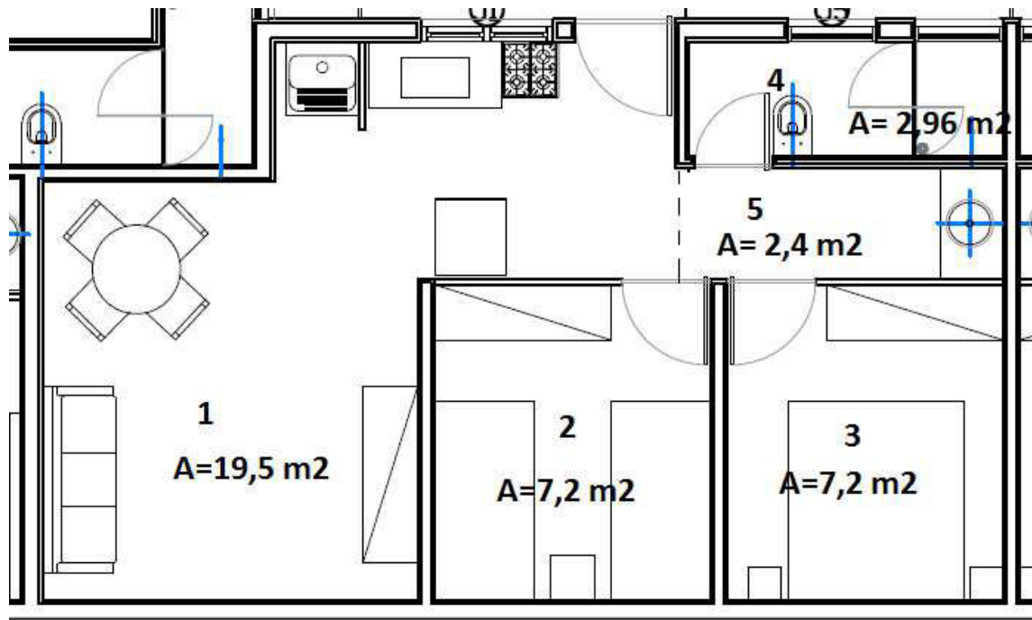
Figura 108: apartamento projetado para a Mauá, separado em cômodos para o cálculo da ventilação.
