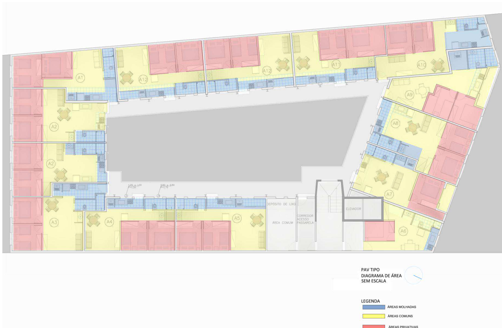
Figura 72: diagrama de área para o pavimento: áreas molhadas, áreas comuns e áreas privativas.
