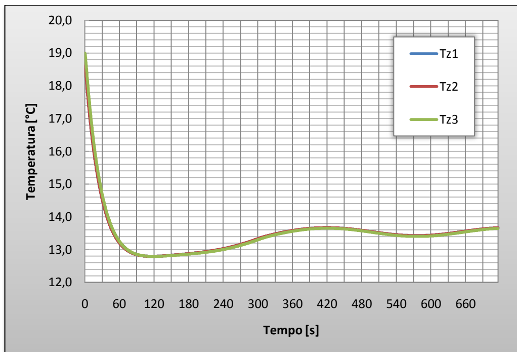
Gráfico 37 - Resposta para uma noite fria no Cenário III.
