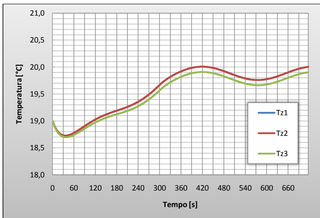
Gráfico 39 - Resposta para uma noite fria no Cenário V.
