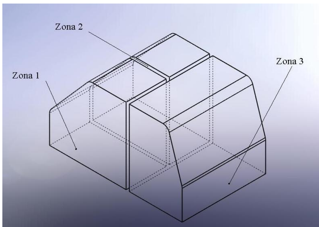
Figura 5 - Modelo 3D com divisão em "zonas" térmicas.
