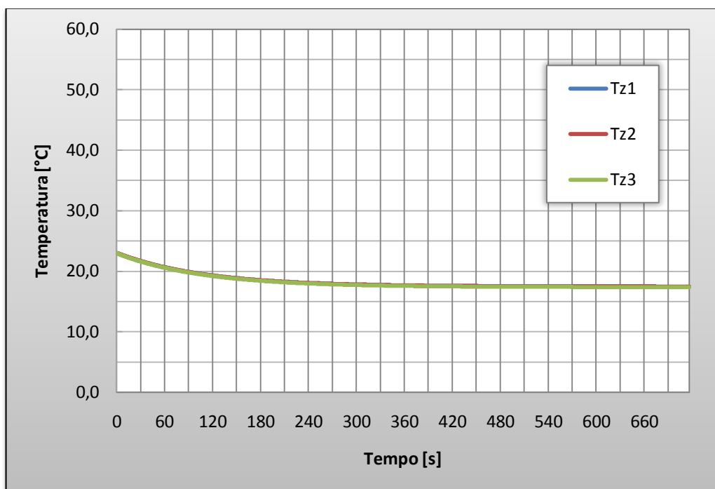
Gráfico 3 - Resultado para T_{ext}=12^{\circ}\text{C} e I_D=0\text{W/m}^2
