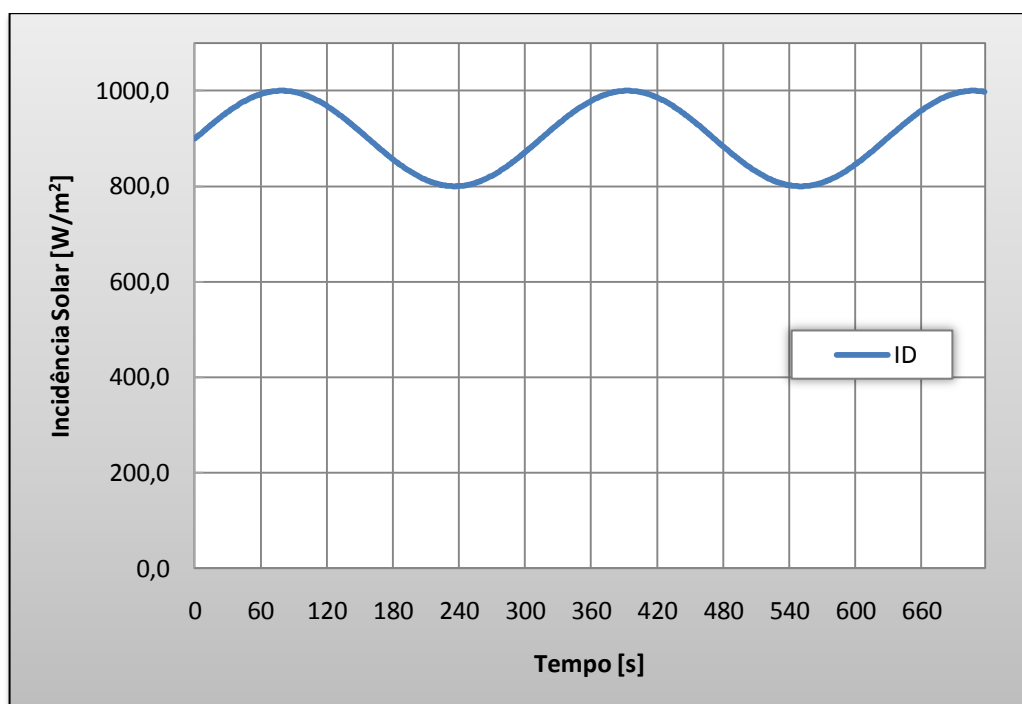
Gráfico 14 - Comportamento de I_D ao longo do tempo.
