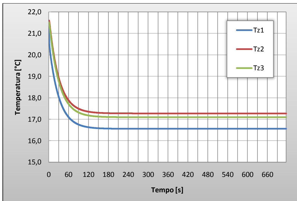
Gráfico 11 - Resultado para T_{ext}=20^{\circ}\text{C} e I_D=500\text{W/m}^2
