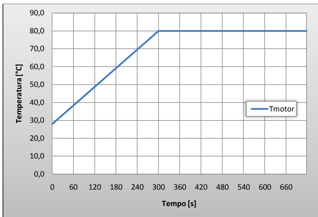
Gráfico 13 - Comportamento de T_{motor} ao longo do tempo.
