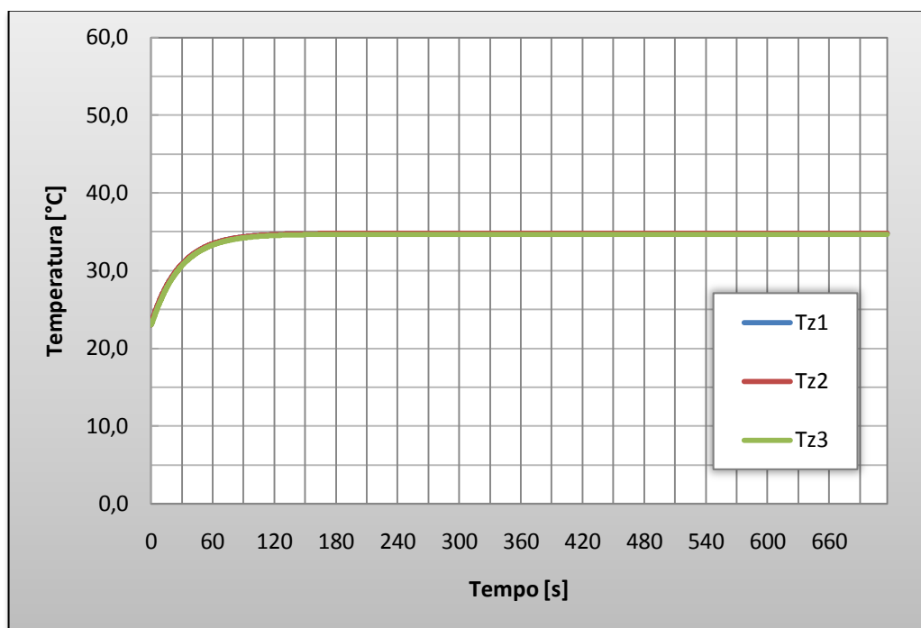
Gráfico 4 - Resultado para T_{ext}=28^{\circ}\text{C} e I_D=1000\text{W/m}^2
