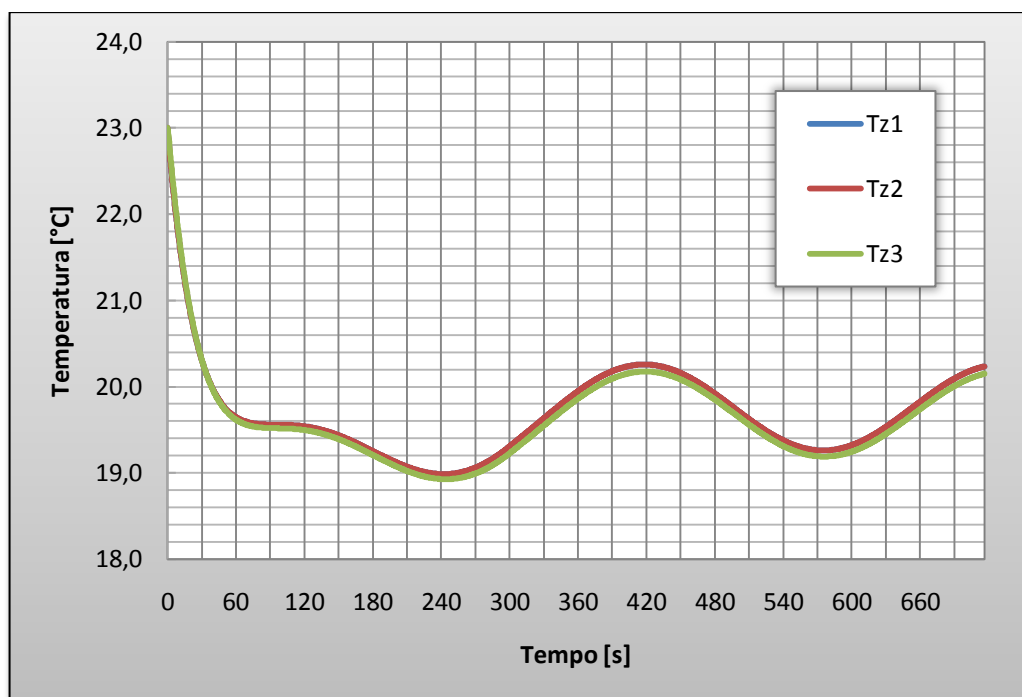
Gráfico 19 - Resposta para um dia típico de verão no Cenário V.
