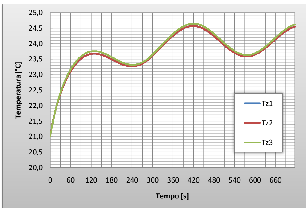
Gráfico 26 - Resposta para um dia encoberto no Cenário II.
