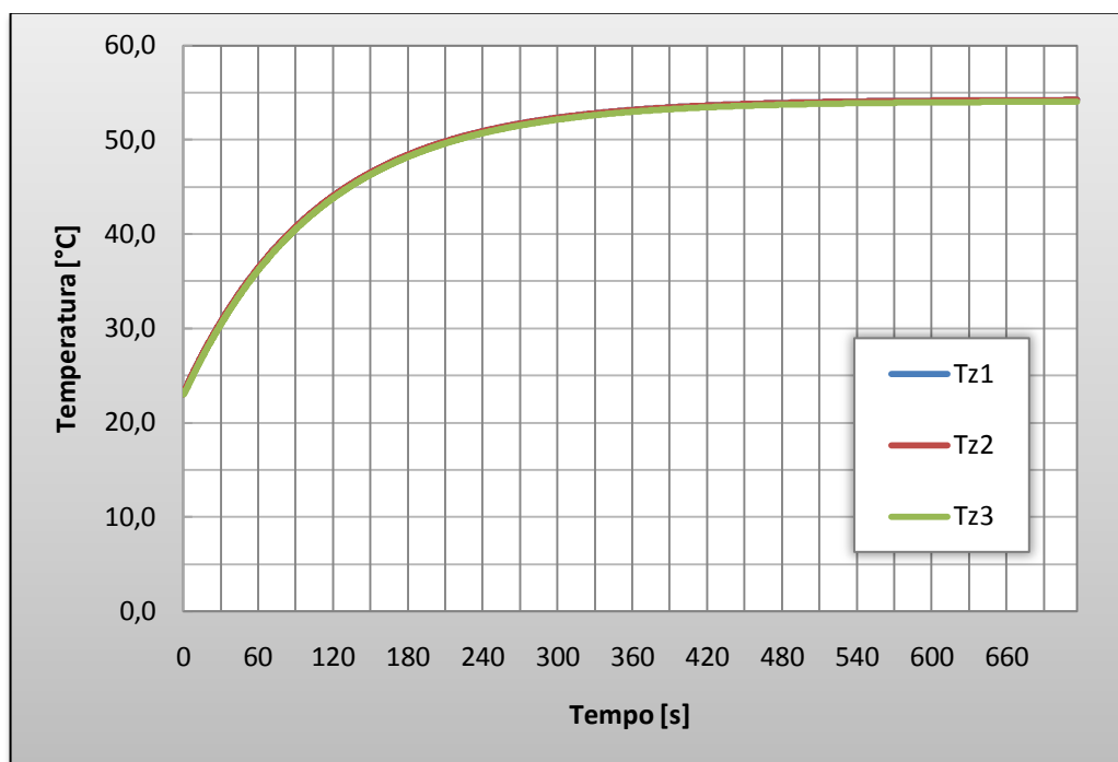
Gráfico 1 - Resultado para T_{ext}=28^{\circ}\text{C} e I_D=1000\text{W/m}^2
