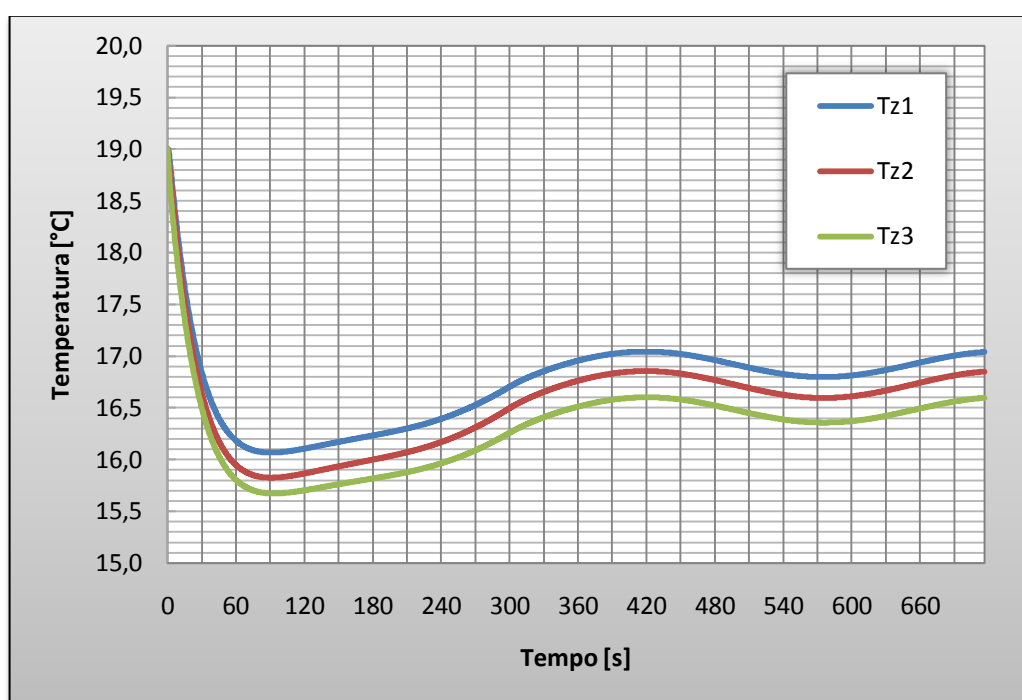
Gráfico 42 - Resposta para uma noite fria no Cenário VIII.
