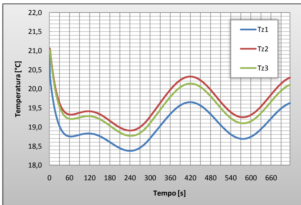
Gráfico 30 - Resposta para um dia encoberto no Cenário VI.
