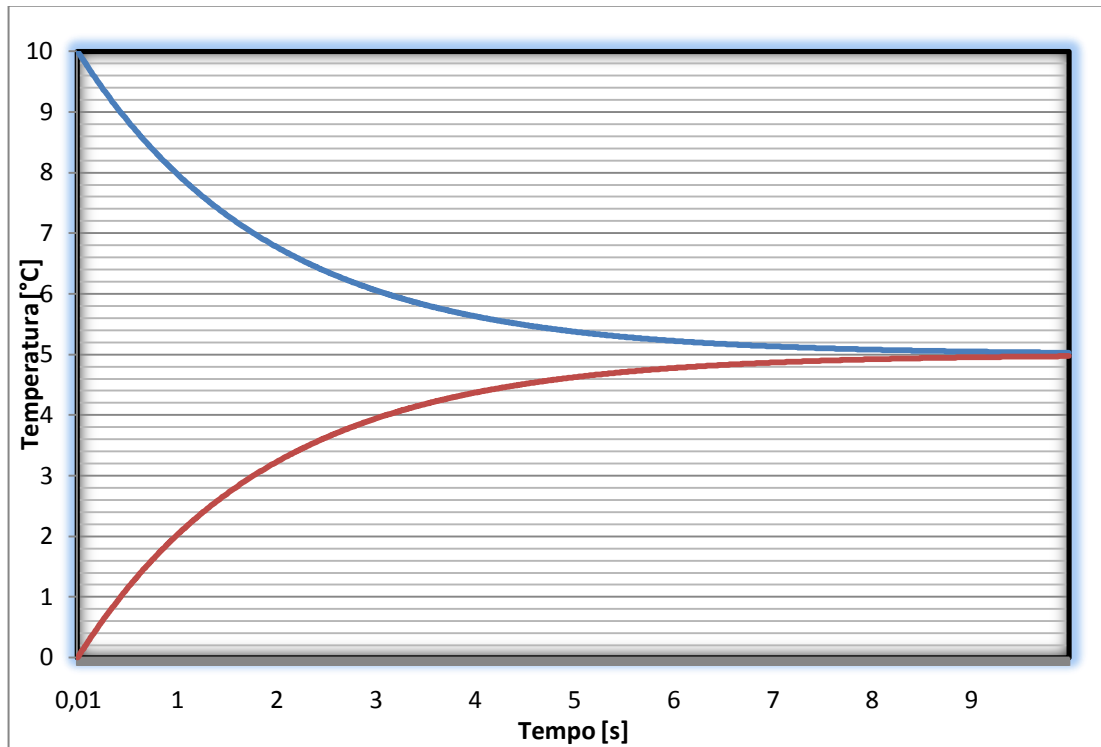
Figura 8 - Análise gráfica para a determinação do valor da resistência térmica do modelo de fluxo de calor entre as zonas 1 e 2.
