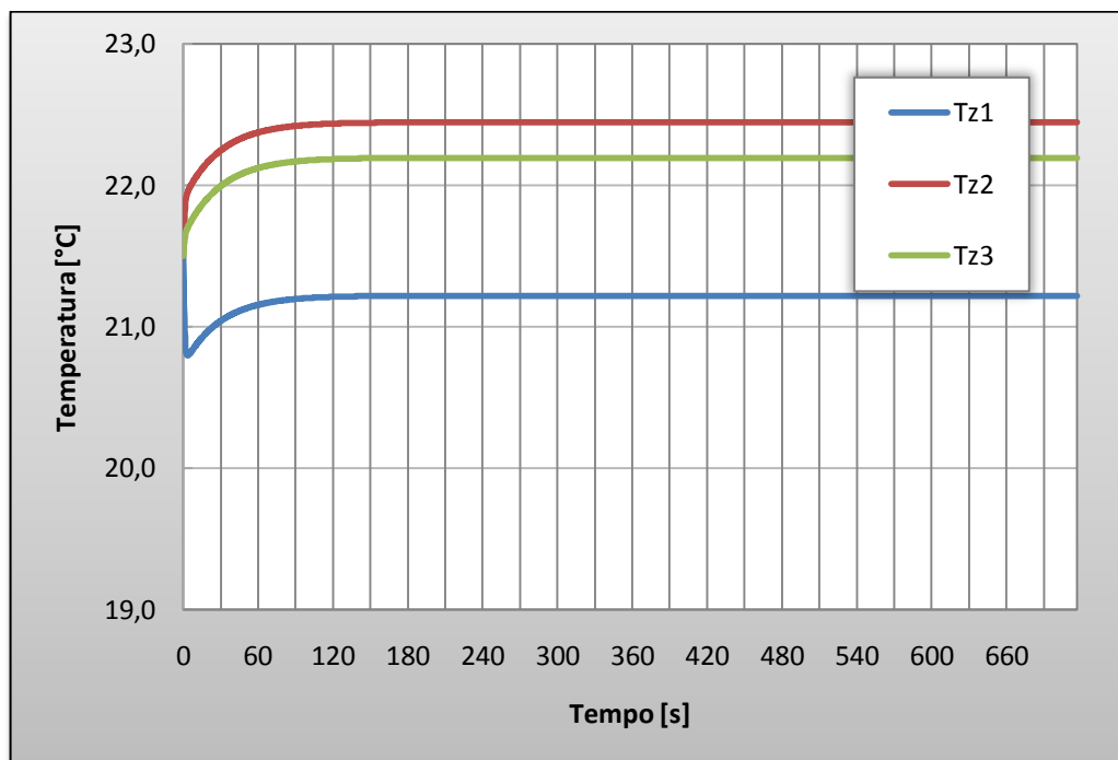
Gráfico 10 - Resultado para T_{ext}=28^{\circ}\text{C} e I_D=1000\text{W/m}^2
