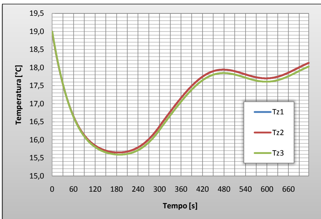
Gráfico 35 - Resposta para uma noite fria no Cenário I.
