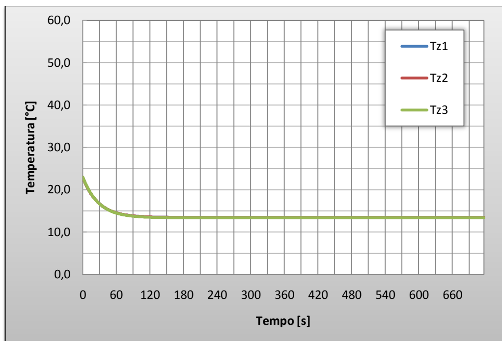
Gráfico 6 - Resultado para T_{ext}=12^{\circ}\text{C} e I_D=0\text{W/m}^2
