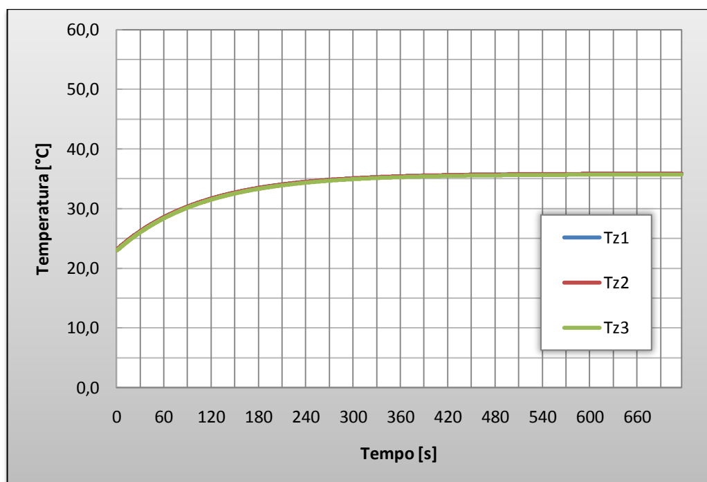
Gráfico 2 - Resultado para T_{ext}=20^{\circ}\text{C} e I_D=500\text{W/m}^2
