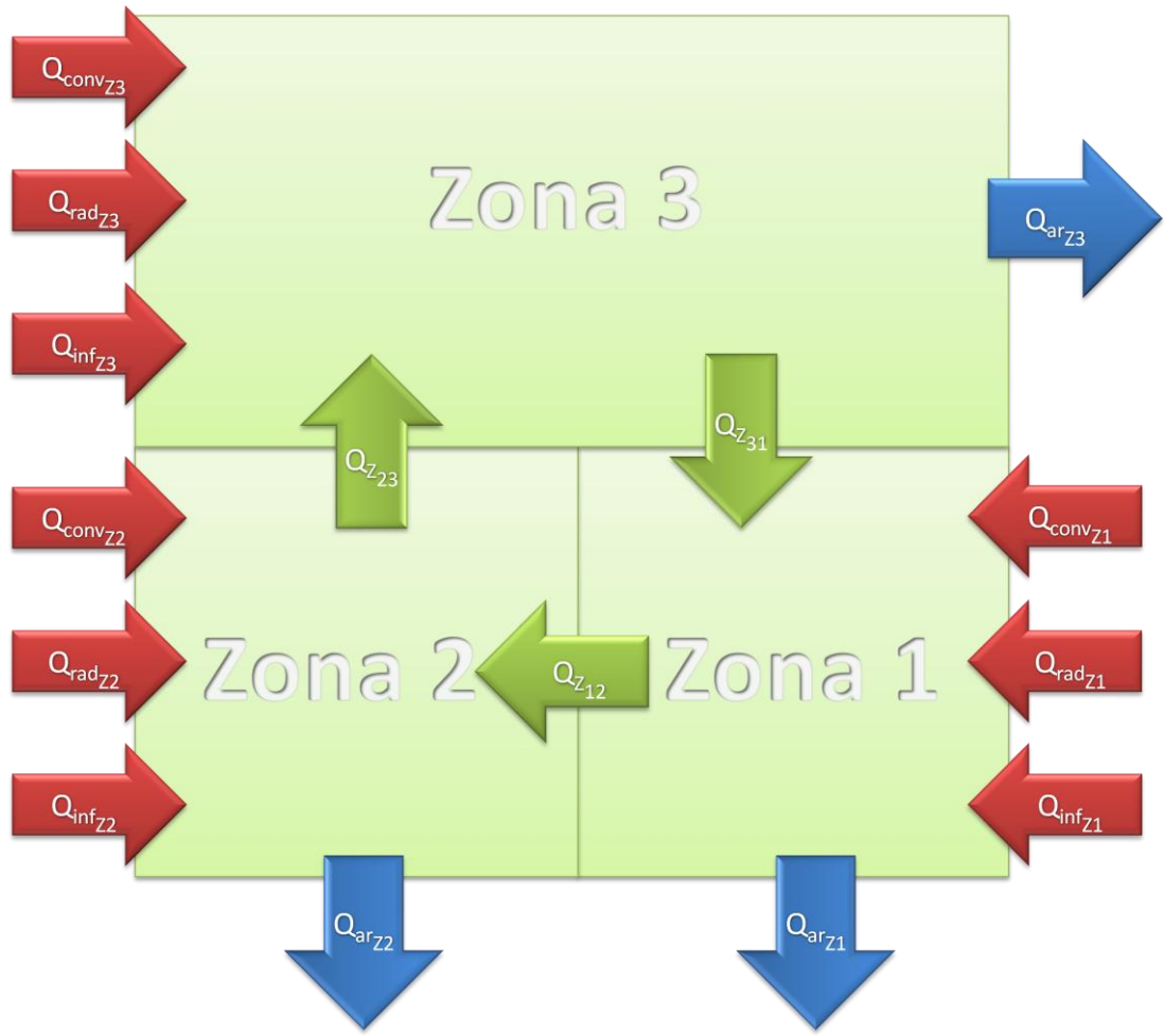
Figura 6 - Diagrama de fluxos de calor no modelo.
