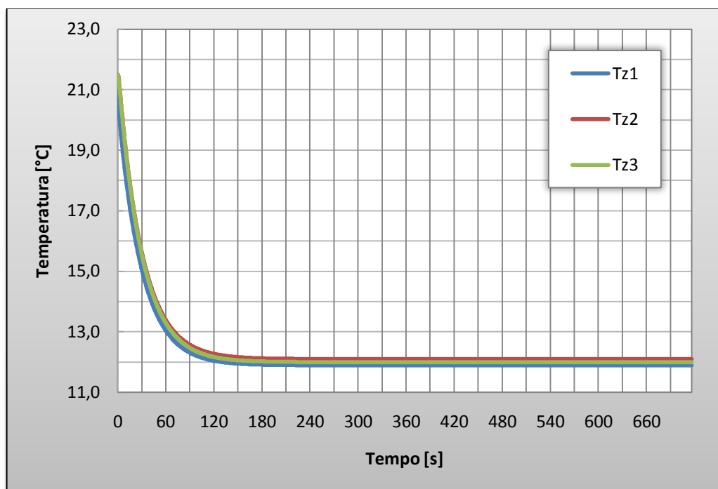
Gráfico 12 - Resultado para T_{ext}=12^{\circ}\text{C} e I_D=0\text{W/m}^2
