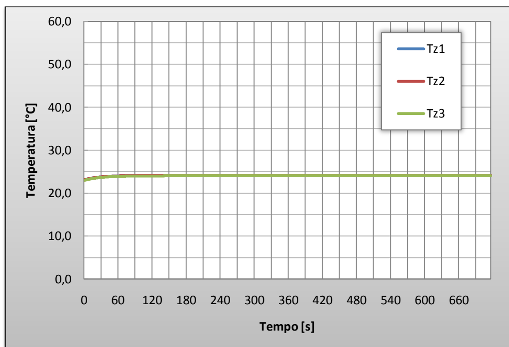
Gráfico 5 - Resultado para T_{ext}=20^{\circ}\text{C} e I_D=500\text{W/m}^2
