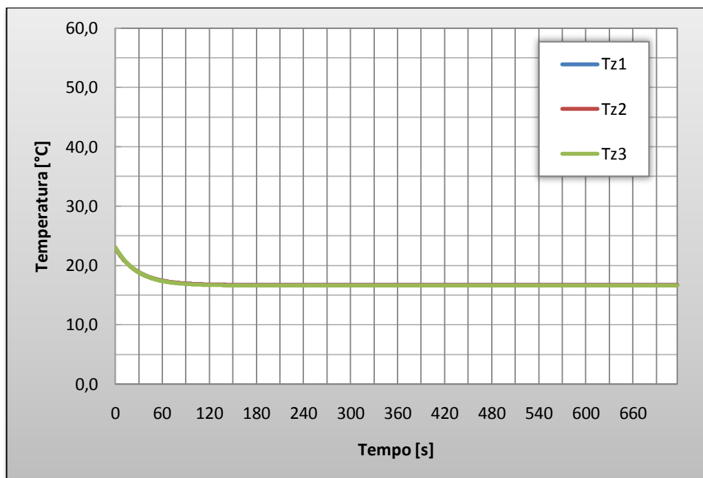
Gráfico 8 - Resultado para T_{ext}=20^{\circ}\text{C} e I_D=500\text{W/m}^2
