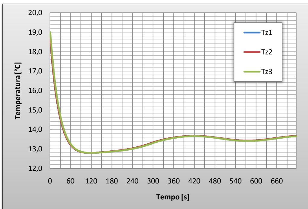
Gráfico 36 - Resposta para uma noite fria no Cenário II.
