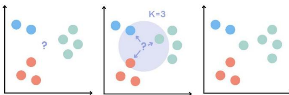
FIGURA 3. Funcionamento do KNN utilizando 3 vizinhos representados no círculo.
