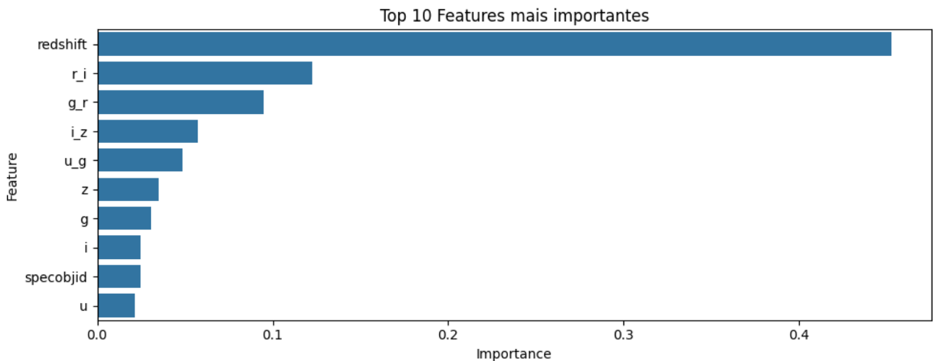
FIGURA 17. Importância das variáveis utilizadas no modelo de classificação de objetos. As features foram ordenadas com base na contribuição relativa para a acurácia do modelo Random Forest: Autoria Própria (2025).
