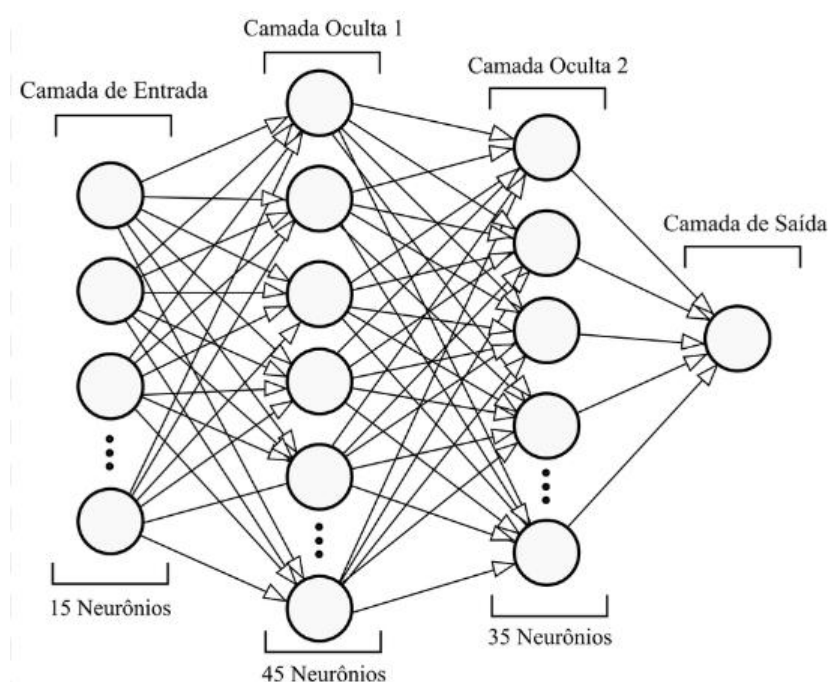
FIGURA 8. Arquitetura de uma MLP com 2 camadas ocultas. Fonte: ResearchGate, 2015
