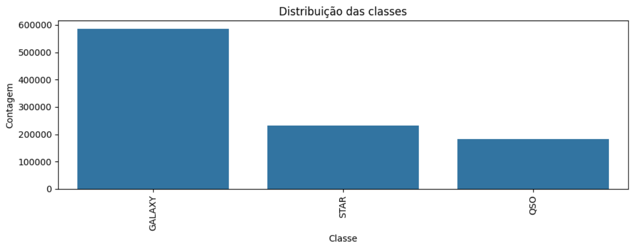
FIGURA 13. Distribuição de classes no conjunto de dados 1: Autoria Própria (2025).
