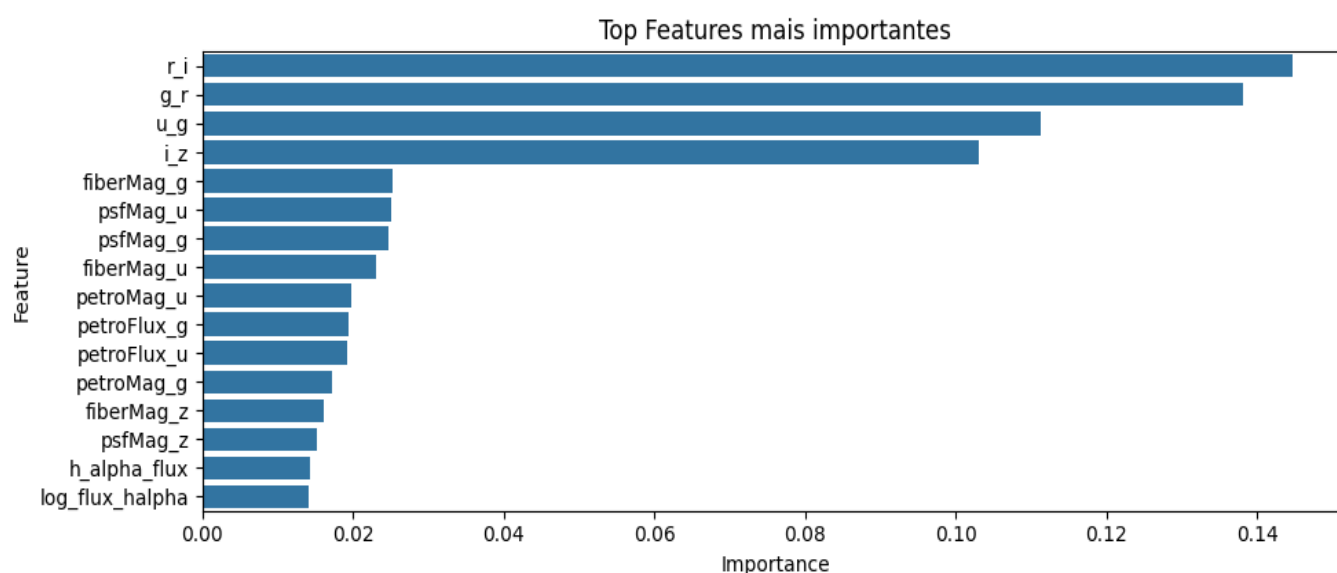
FIGURA 18. Importância das variáveis utilizadas no modelo de classificação espectral estelar. As features foram ordenadas com base na contribuição relativa para a acurácia do modelo Random Forest: Autoria Própria (2025).
