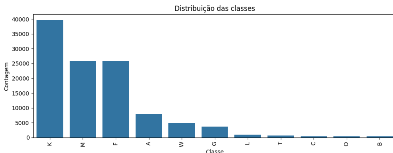
FIGURA 14. Distribuição de classes no conjunto de dados 2: Autoria Própria (2025).
