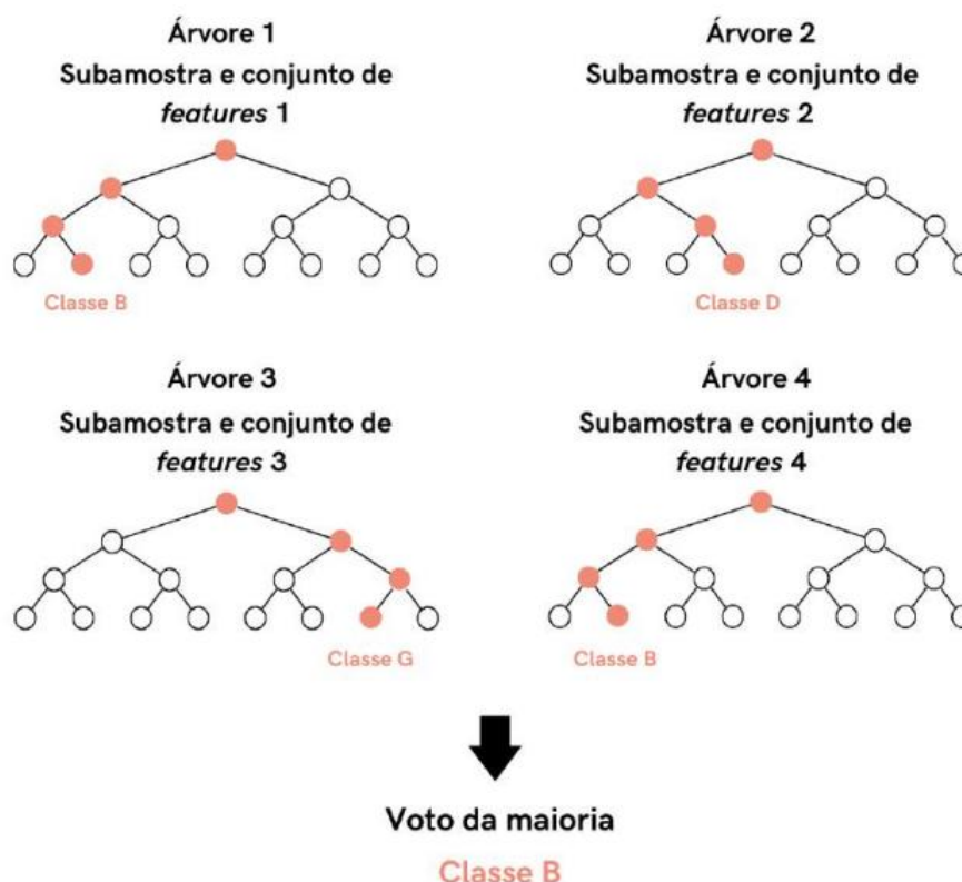
FIGURA 7. Representação de uma classificação com Random forest. Fonte: ALVES, J. C (2022)
