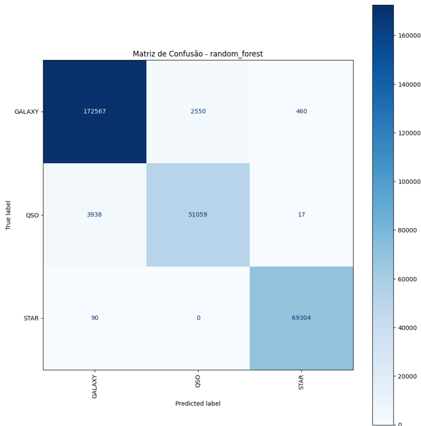
FIGURA 19. Matriz confusão do modelo de classificação de objetos astronômicos: Autoria Própria (2025).
