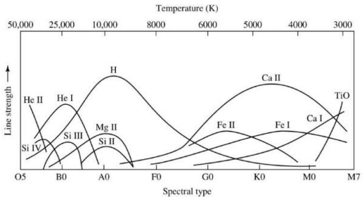
FIGURA 2. A dependência da intensidade das linhas espectrais: CARROLL & OSTLIE (2017).
