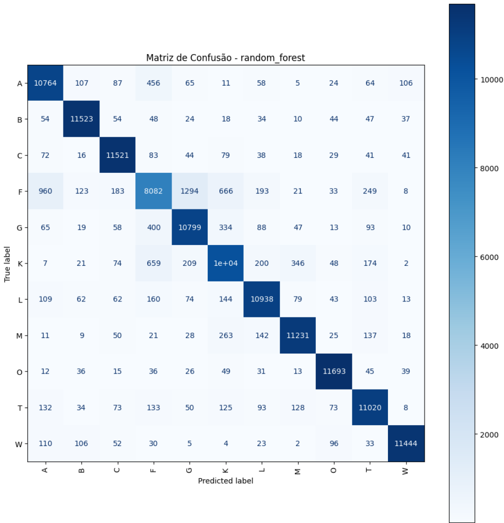
FIGURA 20. Matriz confusão do modelo random forest de classificação de espectros estelares: Autoria Própria (2025).
