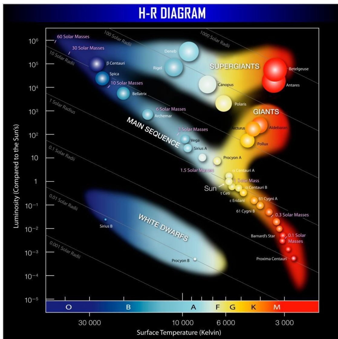
FIGURA 2.1 Diagrama de Hertzsprung-Russell: CARROLL & OSTLIE (2017).
