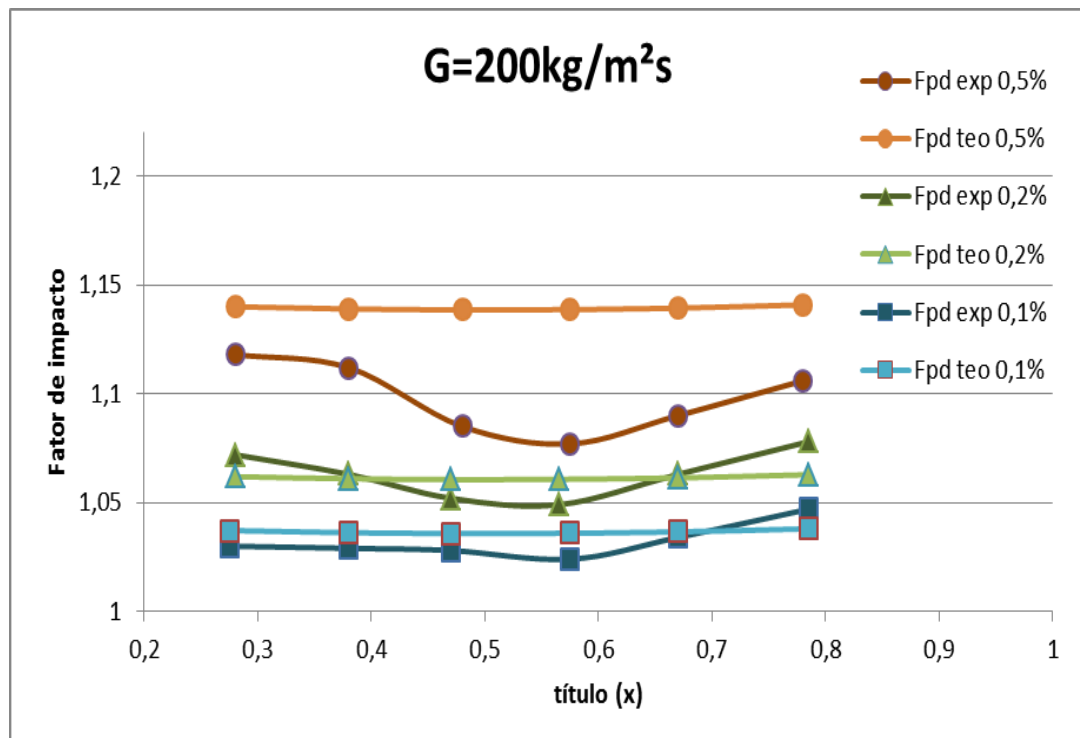
Figura 5.9: Correlação de atrito de Peng em função do título para G=200\text{kg/m}^2\text{s}
