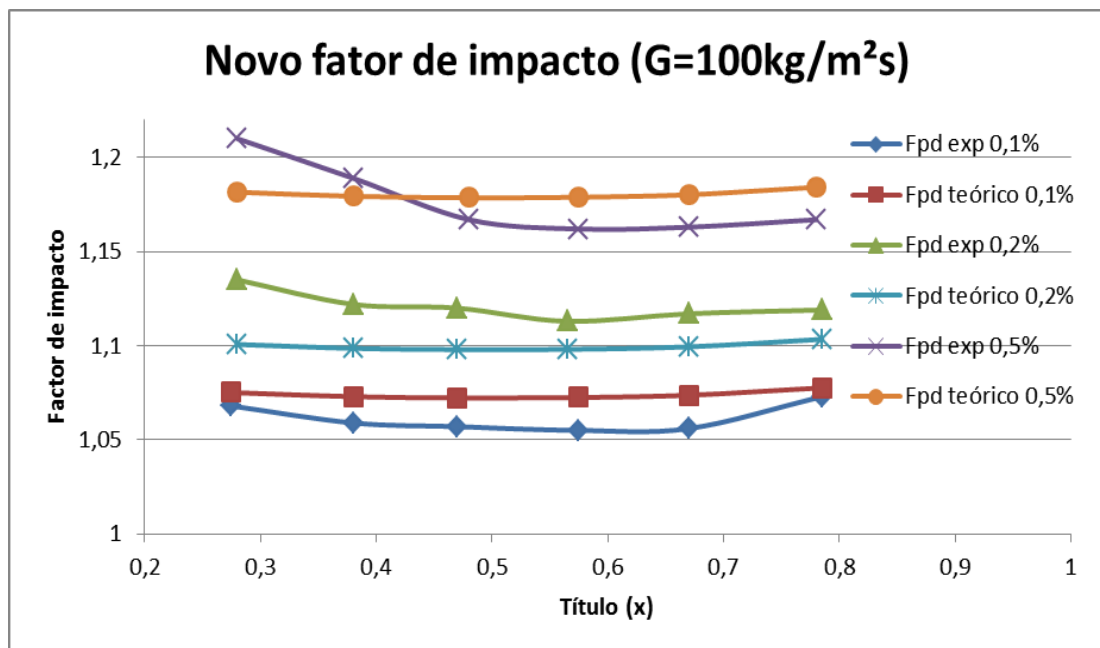
Figura 6.1: Nova correlação de atrito em função do título para G=100\text{kg/m}^2\text{s}
