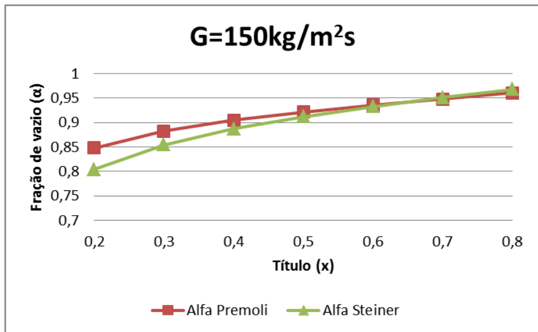
Figura 5.2: Comparativo do cálculo das frações de vazio entre a equação de Premoli e de Steiner para G=150\text{kg/m}^2\text{s}
