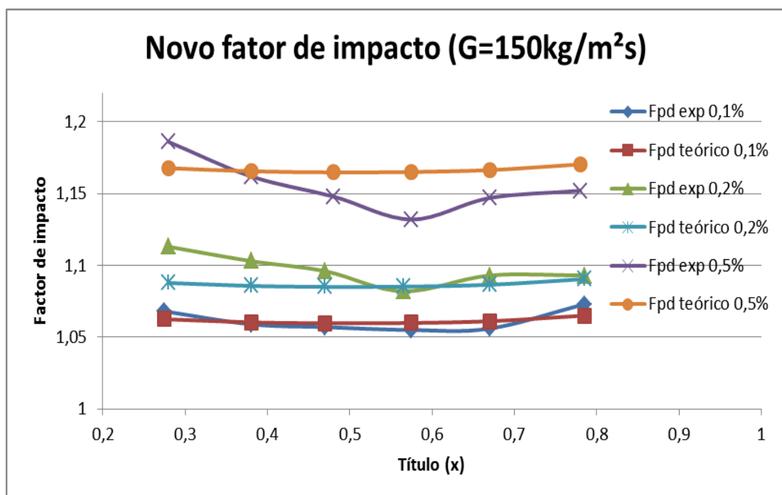
Figura 6.2: Nova correlação de atrito em função do título para G=150\text{kg/m}^2\text{s}
