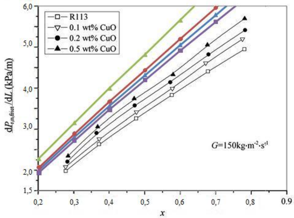
Figura 5.5: Gradiente de pressão em função do título para G=150 \text{ kg} \cdot \text{m}^{-2} \cdot \text{s}^{-1}
