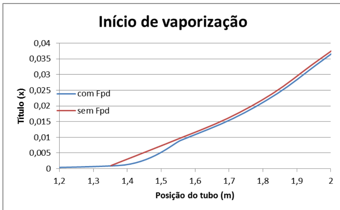
Figura 7.1: Trecho ampliado indicando "atraso" do título em função da posição no tubo capilar quando há nanopartículas (cenários 1 e 2)
