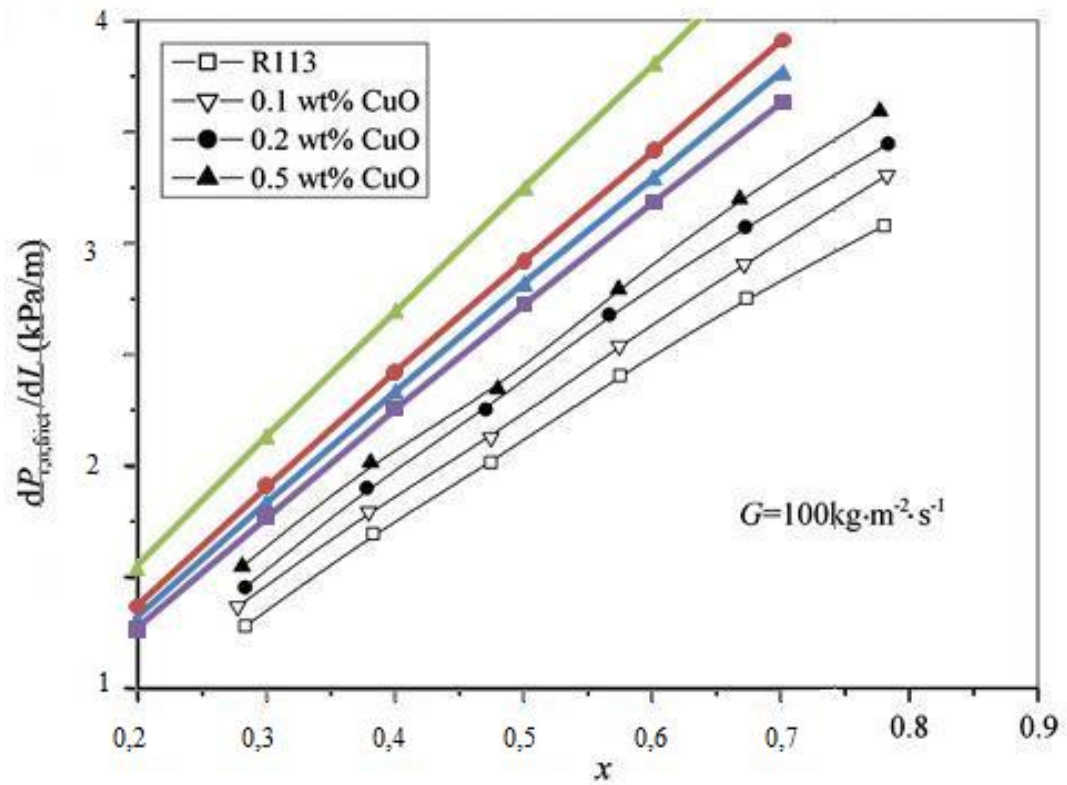
Figura 5.4: Gradiente de pressão em função do título para G=100 \text{ kg/m}^2 \text{s}
