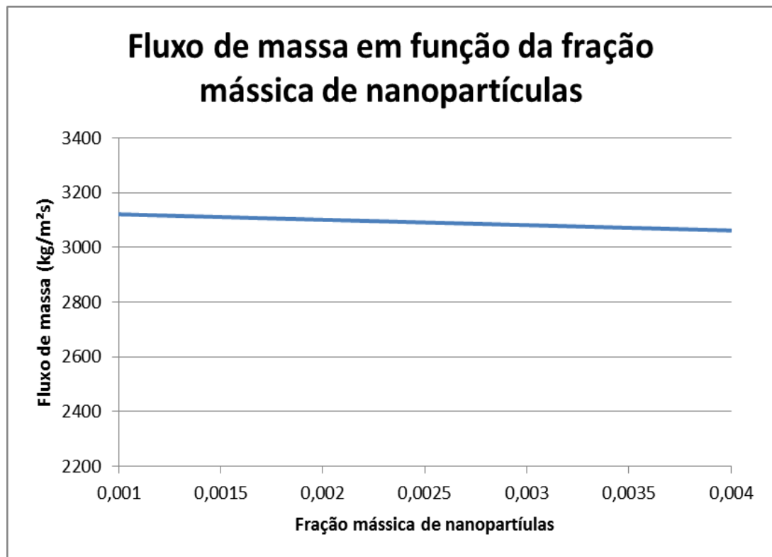
Figura 7.10: Variação do fluxo de massa em função da fração mássica de CuO
