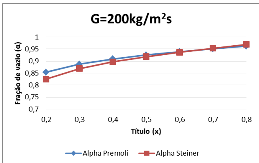
Figura 5.3: Comparativo do cálculo das frações de vazio entre a equação de Premoli e de Steiner para G=200\text{kg/m}^2\text{s}
