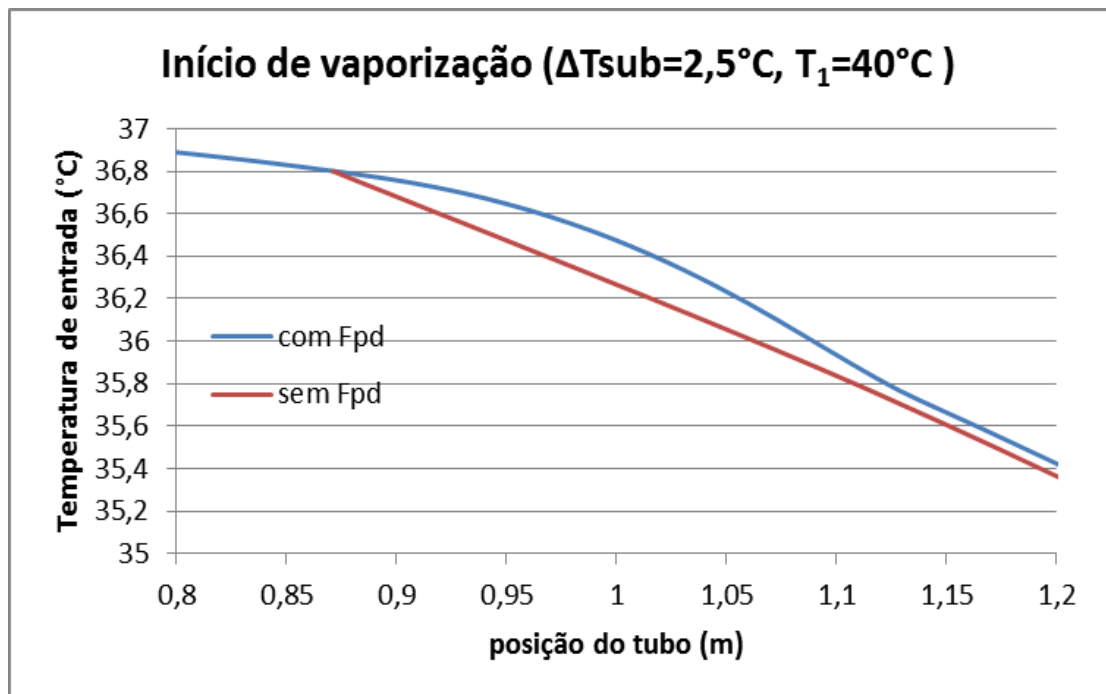
Figura 7.5: Início de vaporização no trecho ampliado do gráfico de temperatura em função da posição do tubo capilar para T_1=40^{\circ}\text{C} e \Delta T_{\text{sub}}=2,5^{\circ}\text{C}
