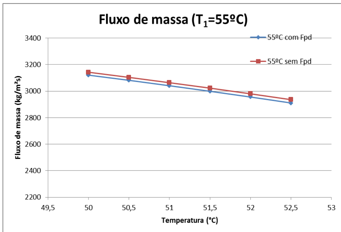
Figura 7.4: Variação do fluxo de massa em função do grau de subresfriamento para T_1=55^\circ\text{C}
