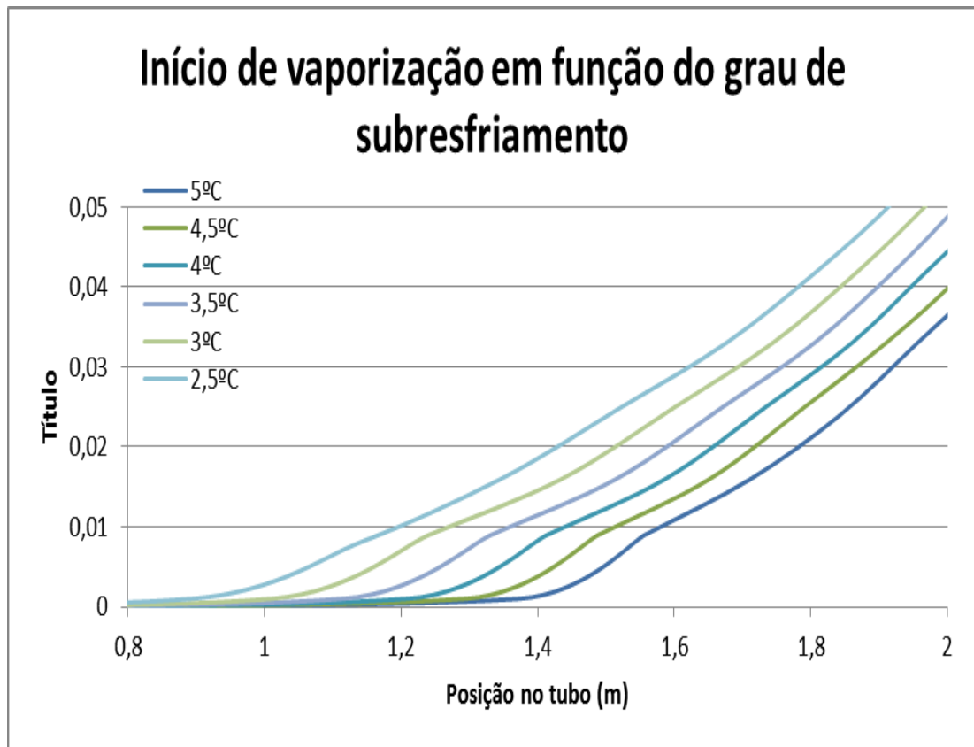
Figura 7.2: Trecho ampliado indicando "atraso" do título em função da posição no tubo capilar quando há nanopartículas (cenários 1 e 2)
