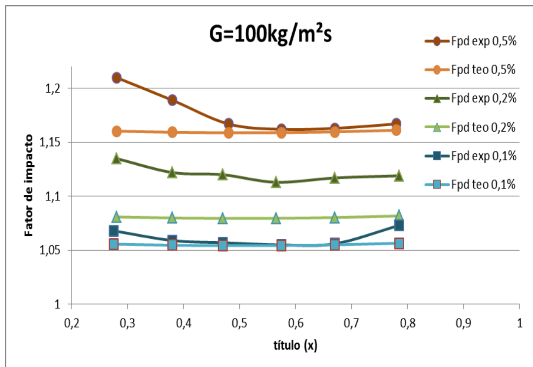
Figura 5.7: Correlação de atrito de Peng em função do título para G=100kg/m 2 s
