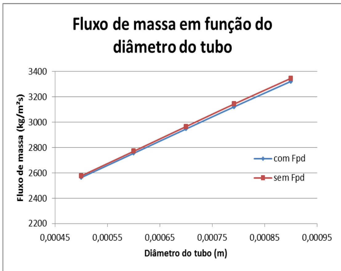
Figura 7.8: Fluxo de massa em função do diâmetro do tubo capilar
