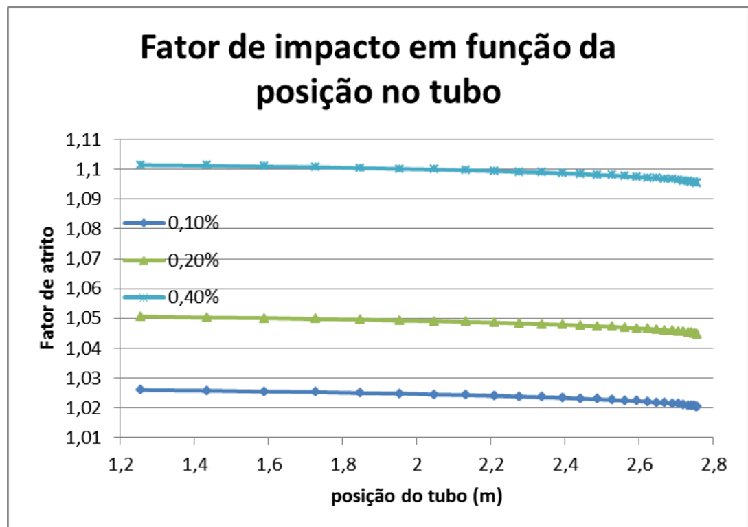
Figura 7.11: Fator de impacto em função da posição do tubo para diferentes frações mássicas de CuO
