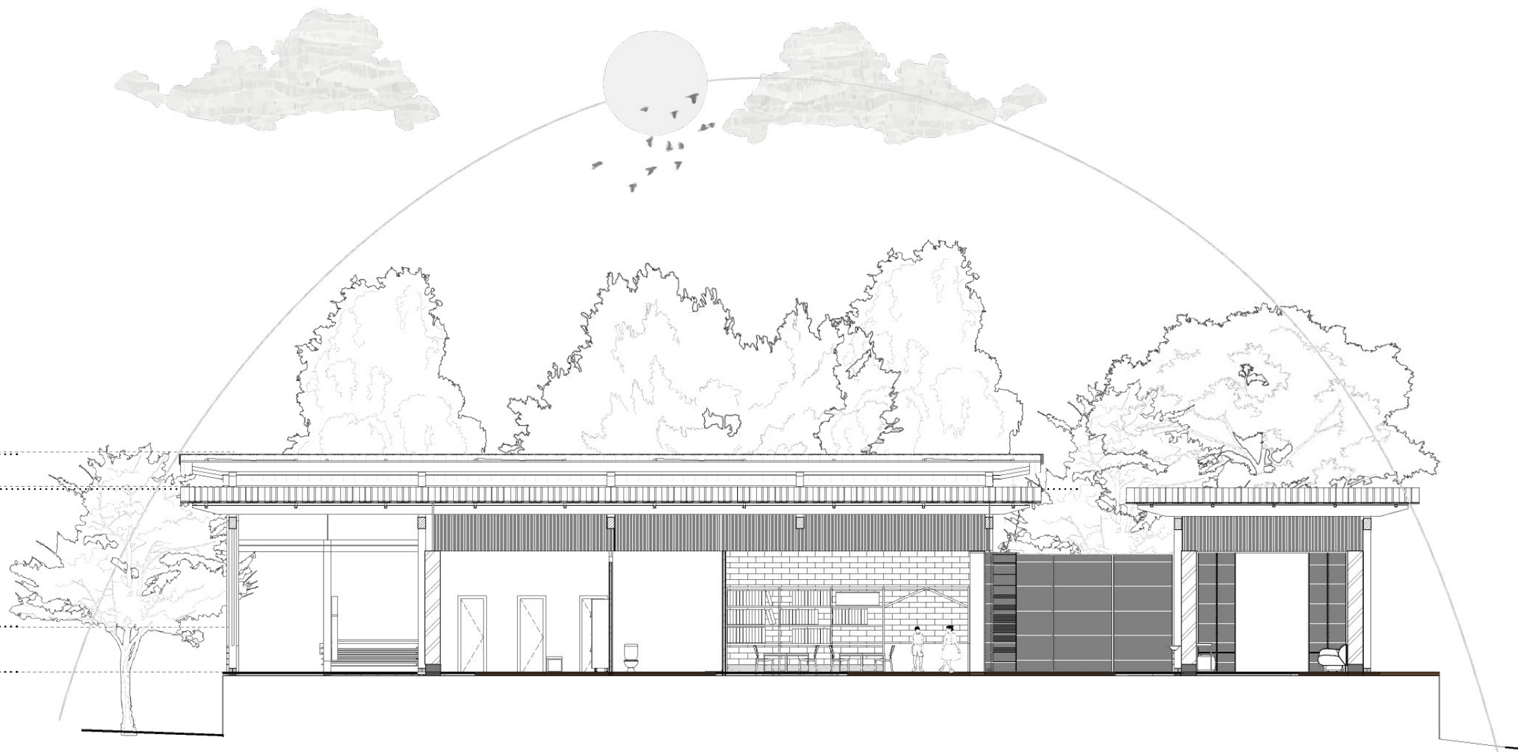
corte A3 | casa das mulheres
