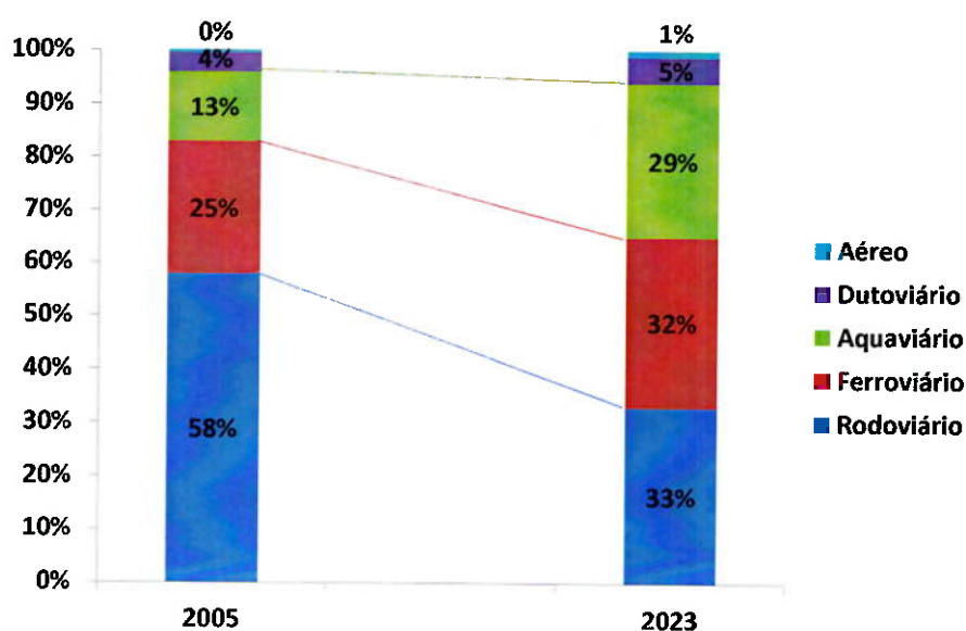
Gráfico 10: Previsão da matriz de transportes brasileira
