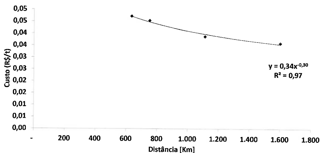
Gráfico 18: Curva de frete hidroviário
