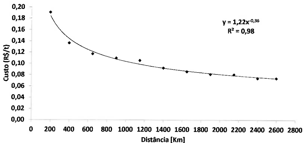
Gráfico 16: Curva de frete rodoviário
