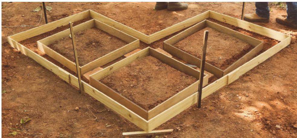
Figura 22 - Montagem das fôrmas para fundação do módulo cubos. Fonte: Caetés, 2017
