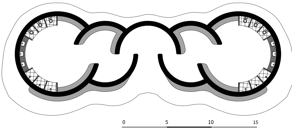
Figura 34 - Planta de proposta para o vestiário em hiperadobe; escala gráfica aima. Fonte: Caetés, 2017
