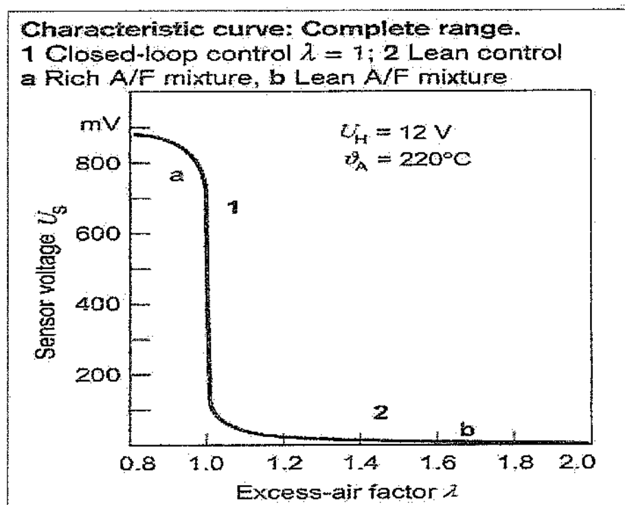
Figura 21 – Curva característica da sonda lambda
