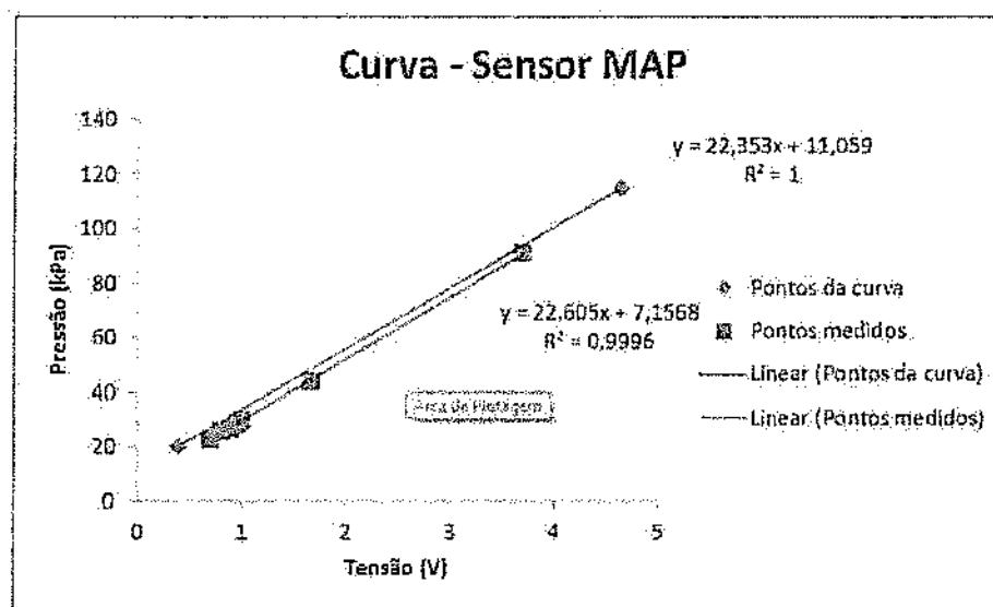
Figura 26 – Interpolação da curva característica do sensor MAP
