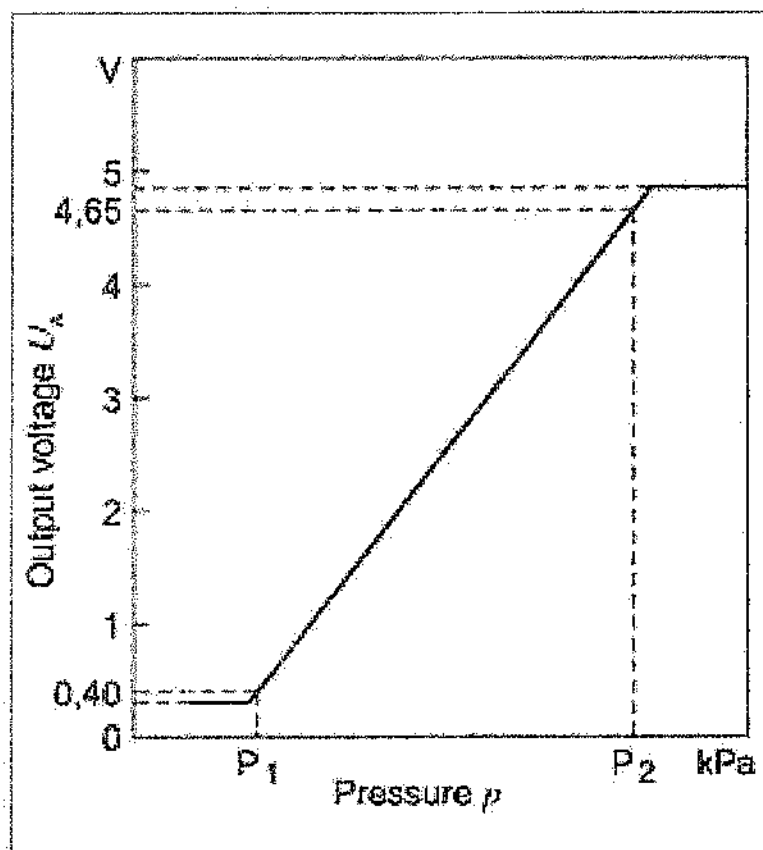
Figura 25 – Curva característica do sensor MAP
