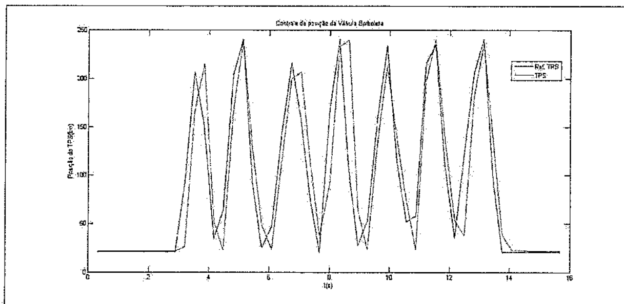
Figura 71 – Gráfico do controle de posição da válvula borboleta com variações bruscas na referência
