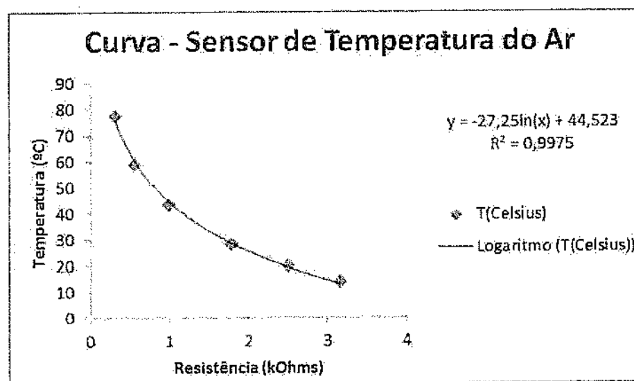
Figura 28 – Interpolação da curva característica do sensor de temperatura do ar
