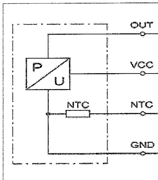
Figura 20 – Diagrama do MAP com o sensor de temperatura integrado
