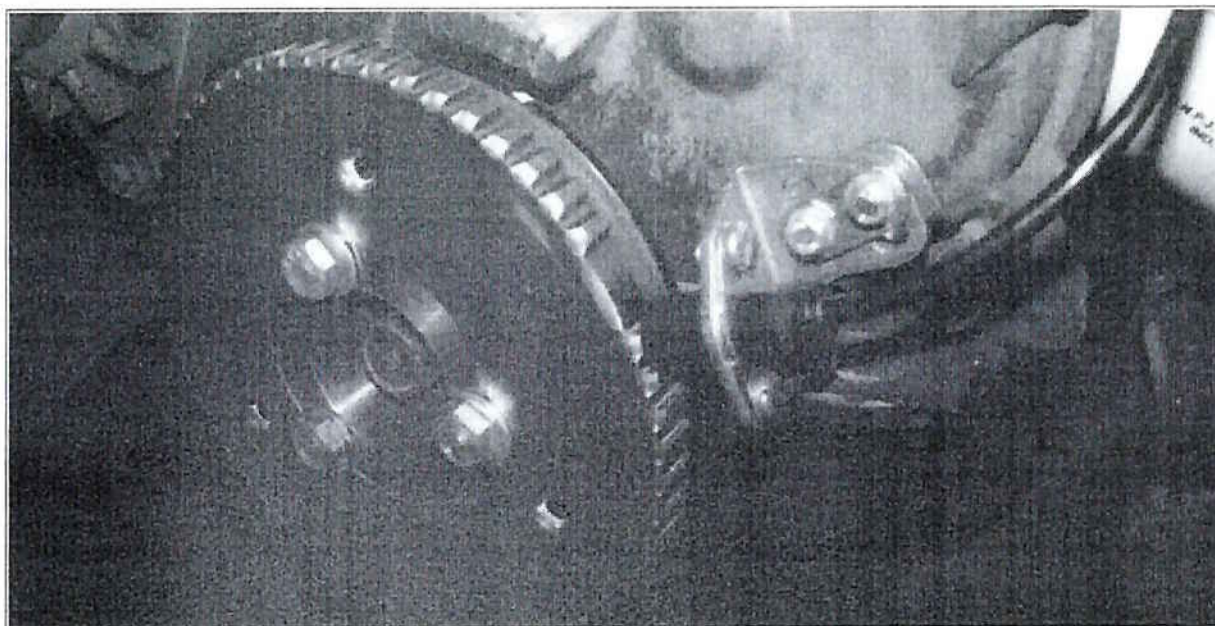
Figura 35 – Roda Fônica equipada com o sensor de rotação
