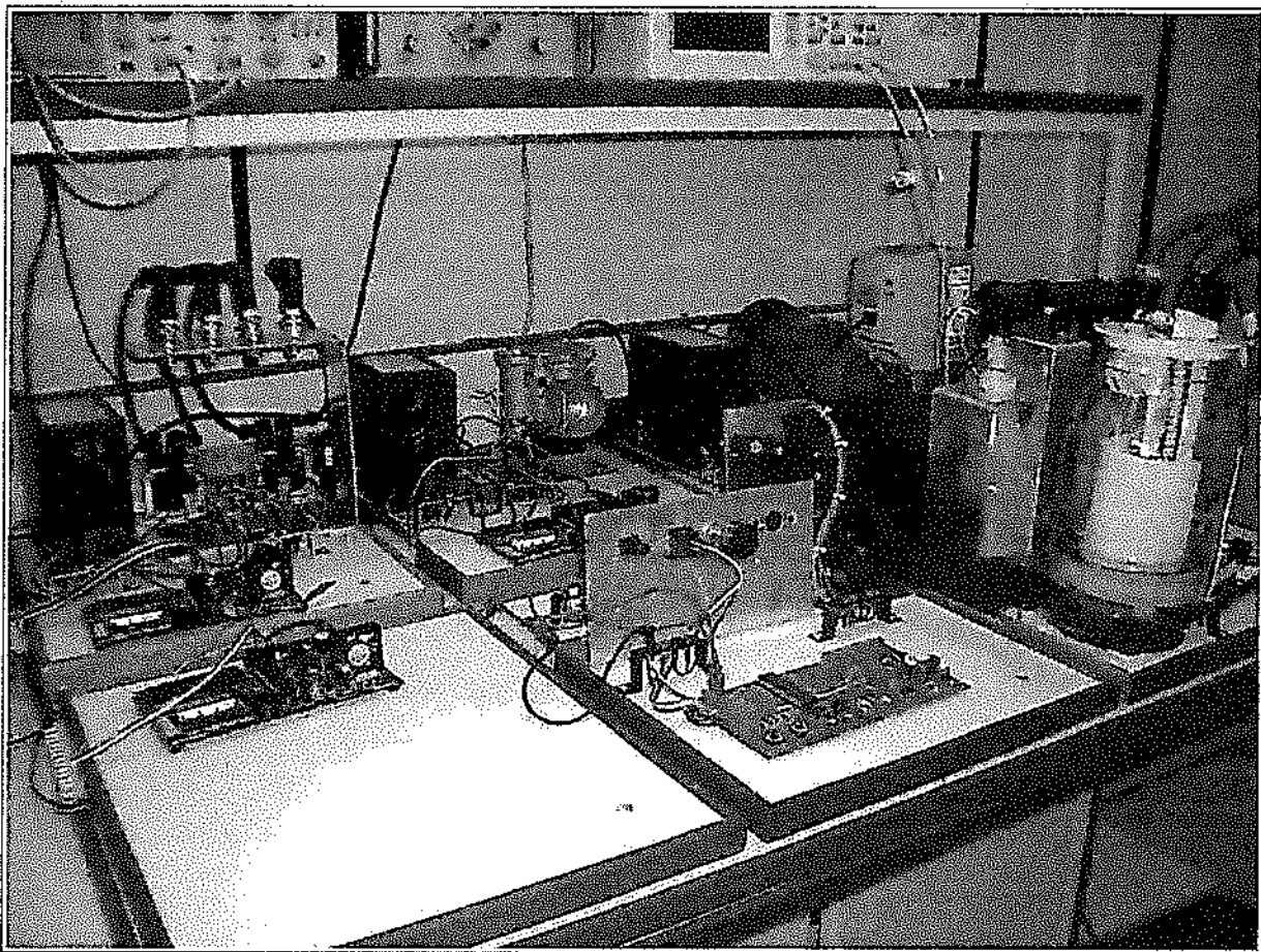
Figura.67 – Bancadas com kits de simulação
