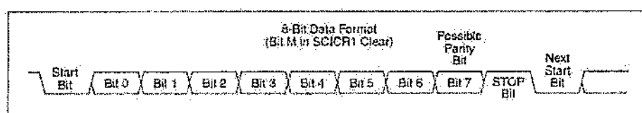
Figura 16 – Formato do protocolo de comunicação UART
