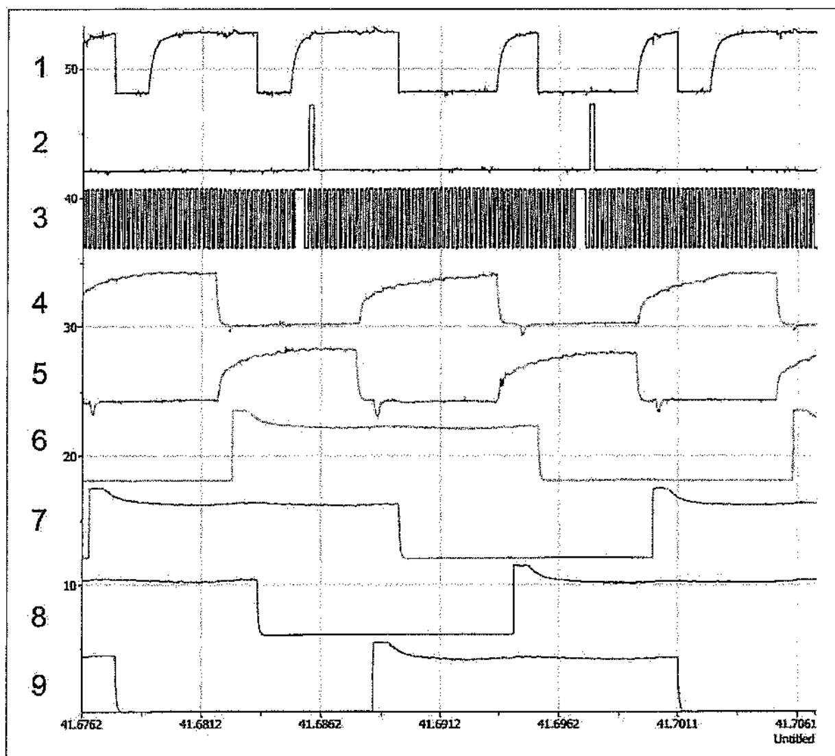
Figura 83 – Sinais de acionamento – Aceleração brusca com carga
