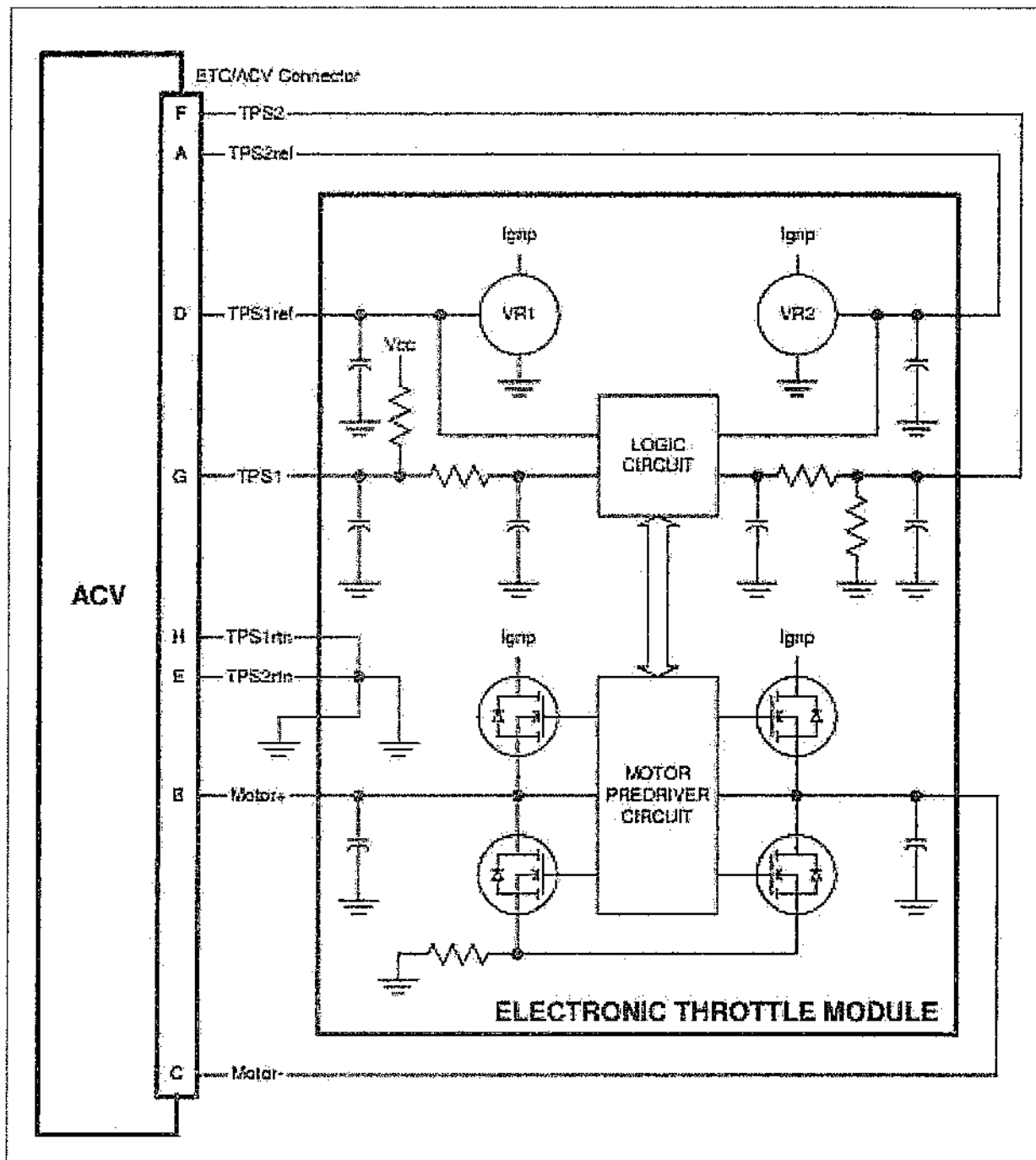
Figura 38 - Diagrama de bloques da válvula borboleta eletrônica
