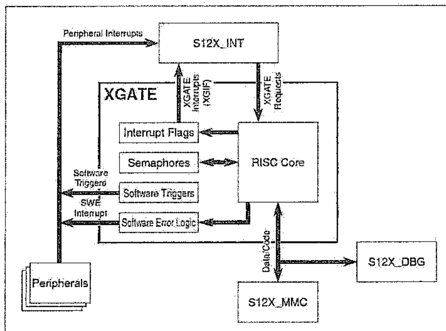
Figura 7 – Diagrama de blocos do coprocessador XGate
