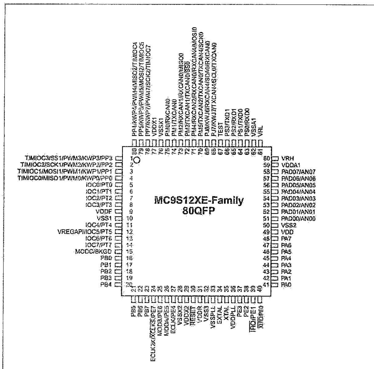
Figura 47 - S12XE com encapsulamento de 80 pinos
