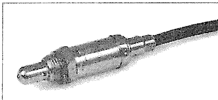
Figura 20 - Sonda Lambda tipo LSM 11
