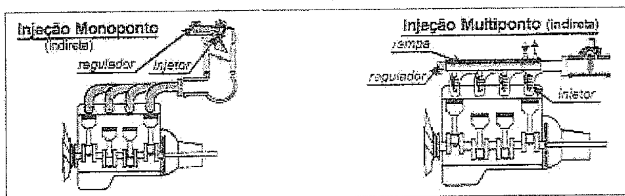
Figura 4 - Injeção Monoponto e Multiponto
