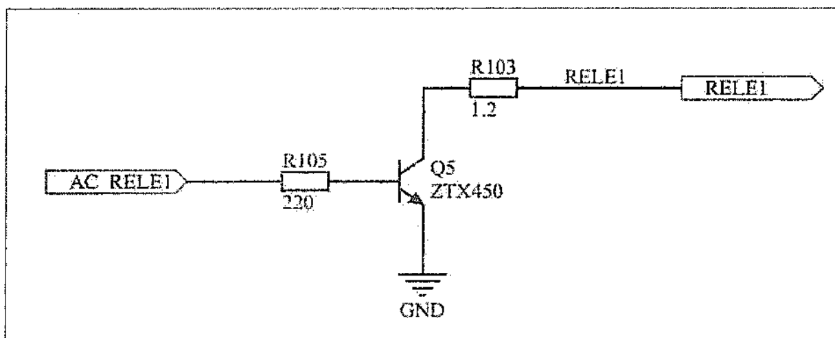
Figura 58 – Esquema elétrico do acionamento de relé
