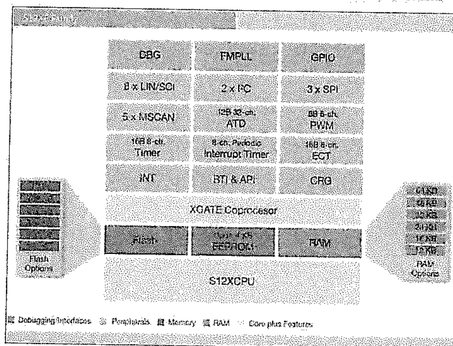
Figura 6 – Diagrama de blocos da família de microcontroladores S12XE
