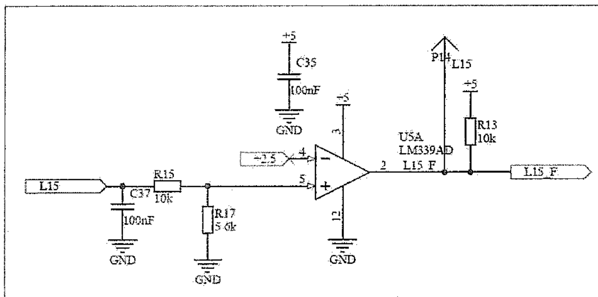
Figura 51 – Esquema elétrico do comparador de tensão
