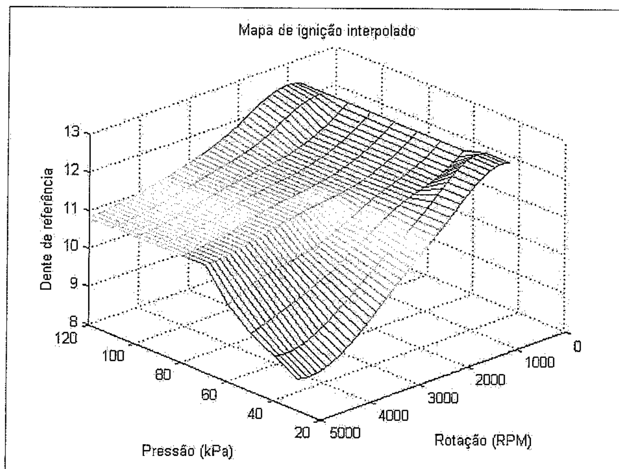
Figura 62 – Gráfico 3D do mapa de ignição final
