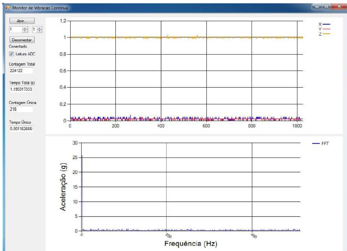
Figura 4.9: Espectro do eixo X para o patamar de ruído retirado sobre a bancada.
