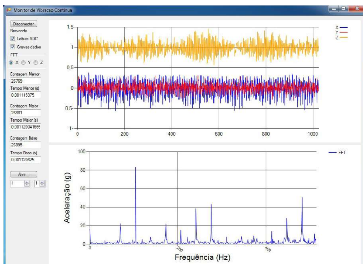
Figura 4.36: Espectro do eixo X do motor de indução à 1798rpm (1 carga).
