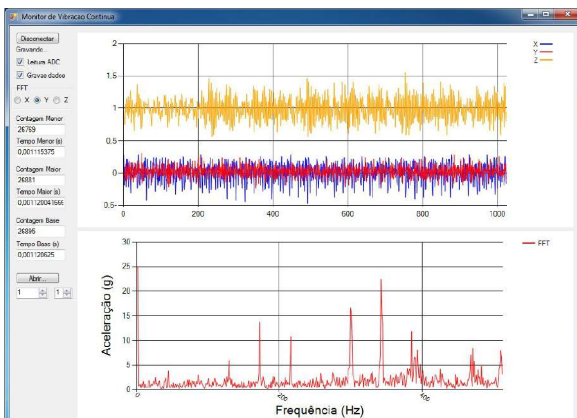
Figura 4.47: Espectro do eixo Y do motor de indução à 2240rpm (em 75,0Hz com blindagem).
