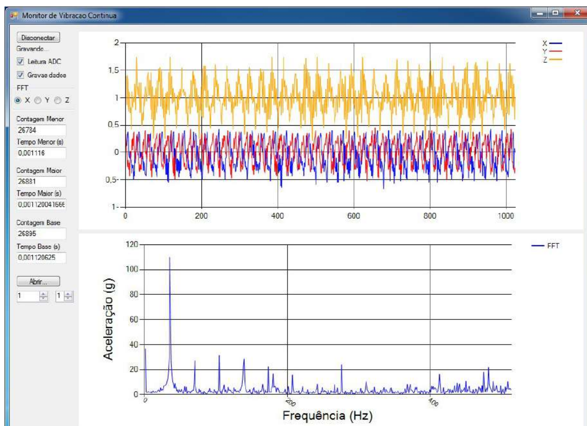
Figura 4.14: Espectro do eixo X para o motor DC de 1700W com carga de 600W.
