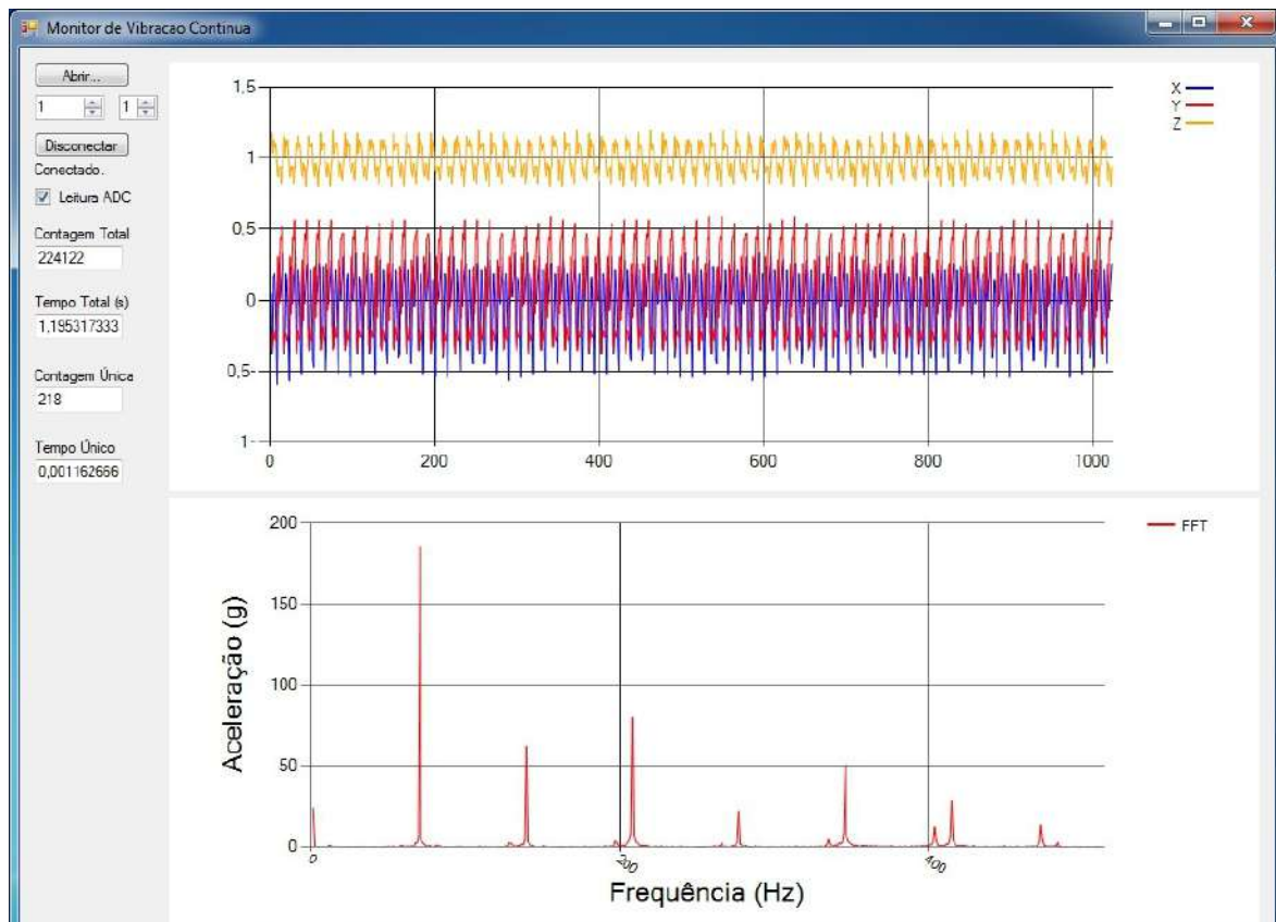
Figura 4.6: Espectro do eixo Y para o motor DC de 12V à velocidade de 3460rpm.
