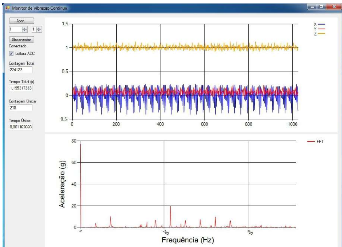
Figura 4.33: Espectro do eixo Y do motor de indução à 1790rpm (sem blindagem).
