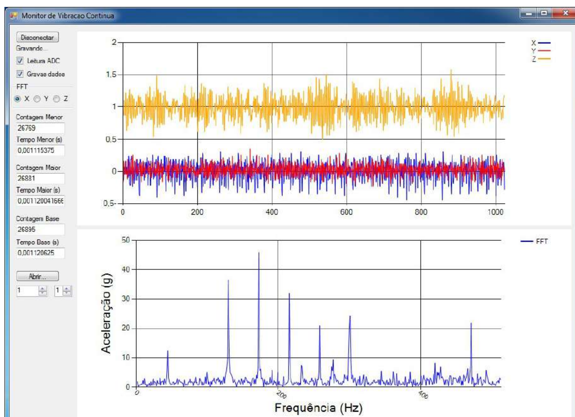
Figura 4.46: Espectro do eixo X do motor de indução à 2240rpm (em 75,0Hz com blindagem).
