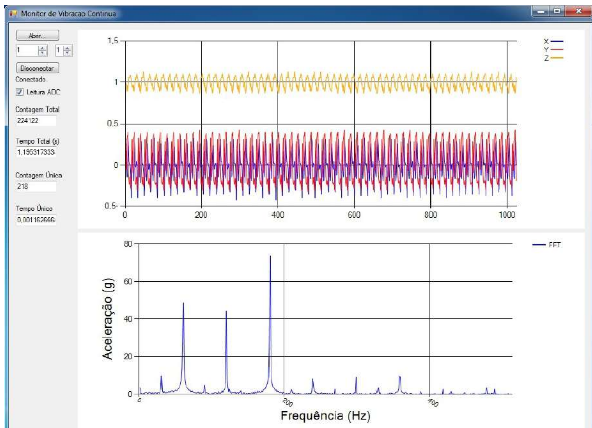
Figura 4.3: Espectro do eixo X para o motor DC de 12V à velocidade de 2995rpm.
