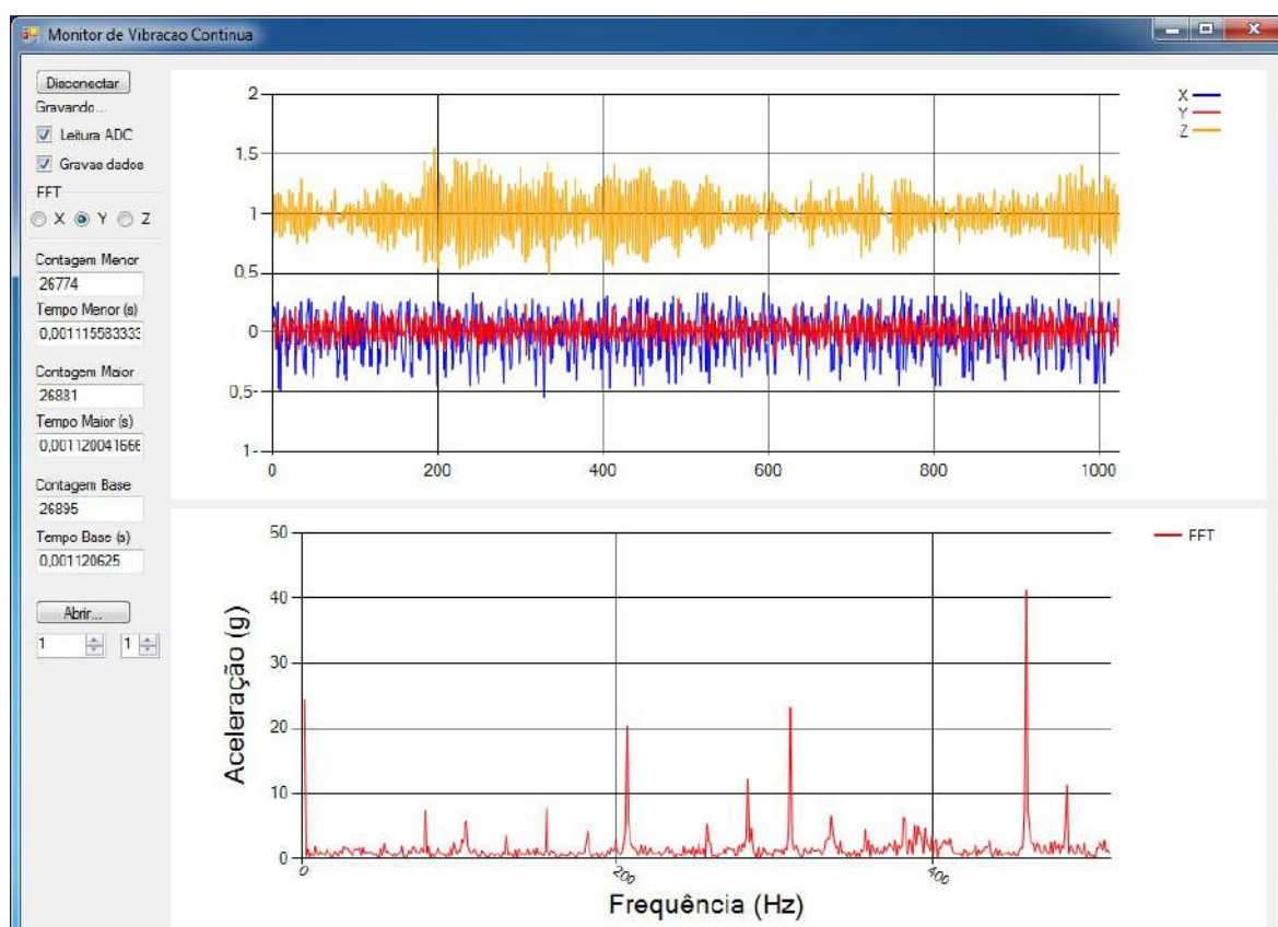
Figura 4.45: Espectro do eixo Y do motor de indução à 1343rpm (em 44,9Hz com blindagem).
