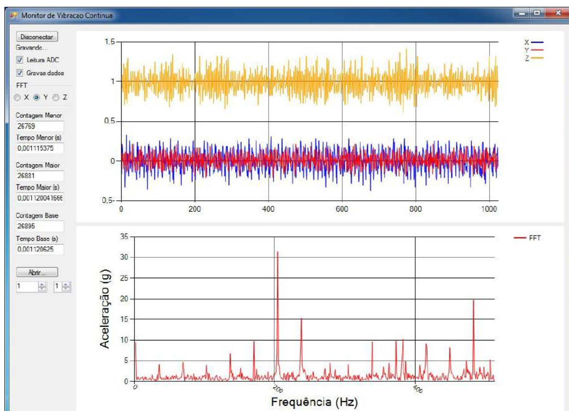
Figura 4.41: Espectro do eixo Y do motor de indução à 1770rpm (3 cargas em paralelo).
