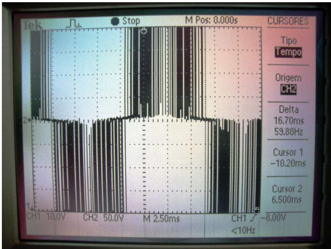
Figura 3.20: Forma de onda da saída do inversor de frequência em 60,2Hz.
