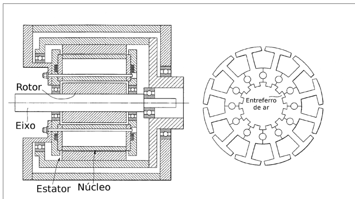
Figura 2.4: Modelo de máquina elétrica rotativa.
