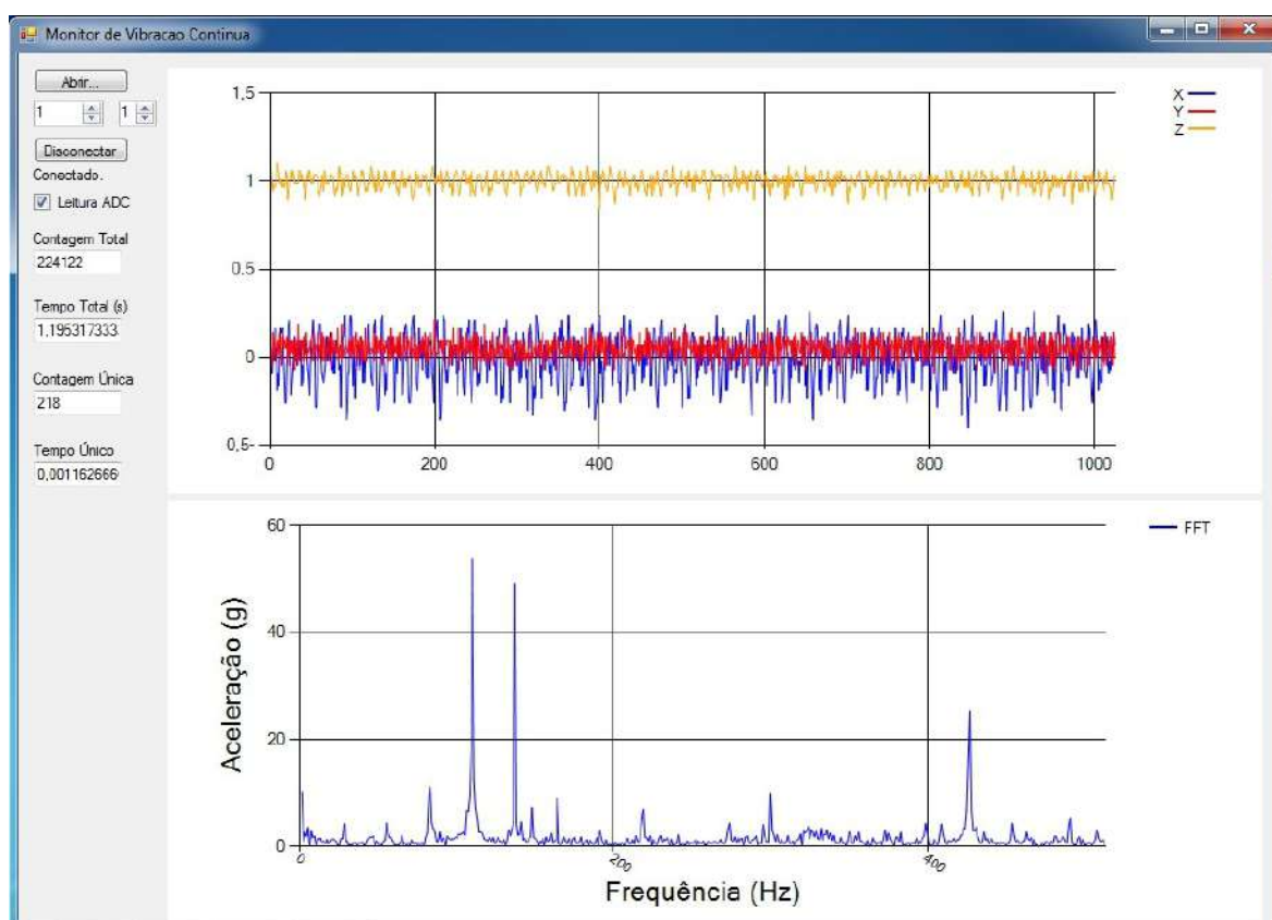
Figura 4.48: Espectro do eixo X do motor de indução à 1366rpm (em 45,6Hz sem blindagem).
