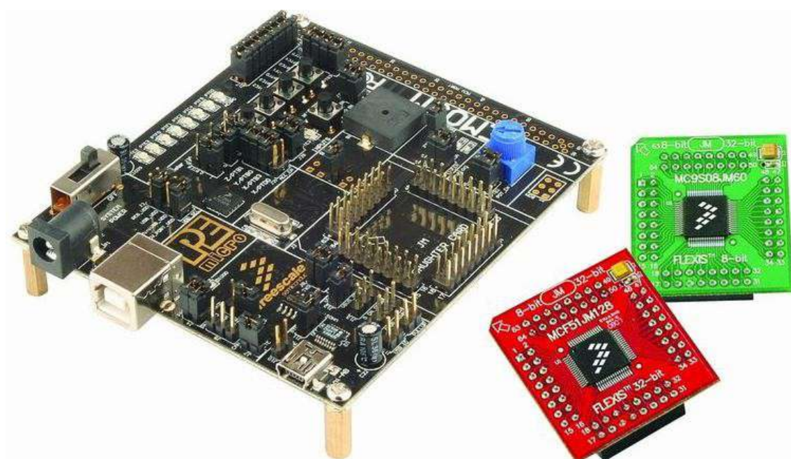
Figura 1: Kit de desenvolvimento DEMOJM.
