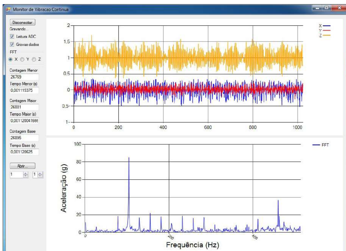
Figura 4.44: Espectro do eixo X do motor de indução à 1343rpm (em 44,9Hz com blindagem).
