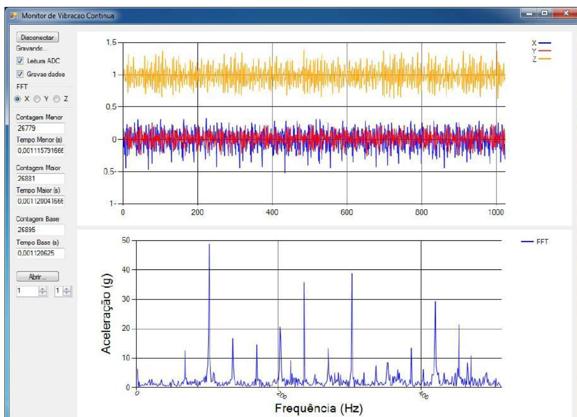
Figura 4.42: Espectro do eixo X do motor de indução à 1758rpm (4 cargas em paralelo).
