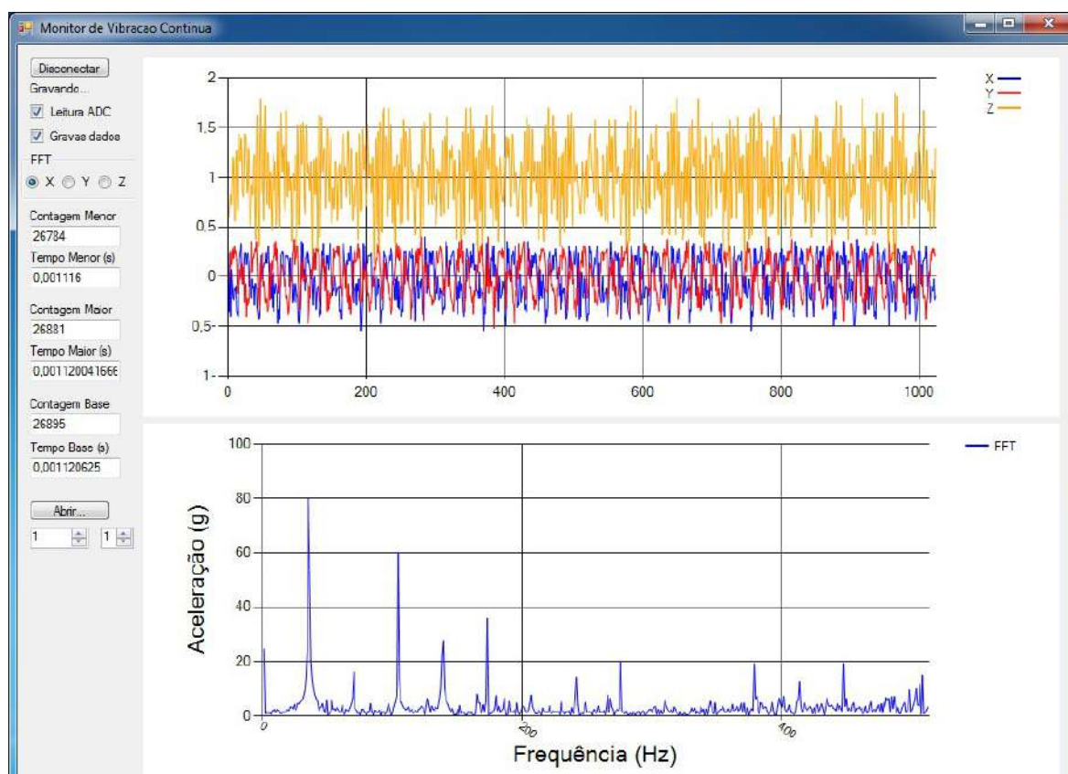
Figura 4.11: Espectro do eixo X para o motor DC de 1700W com carga de 300W.
