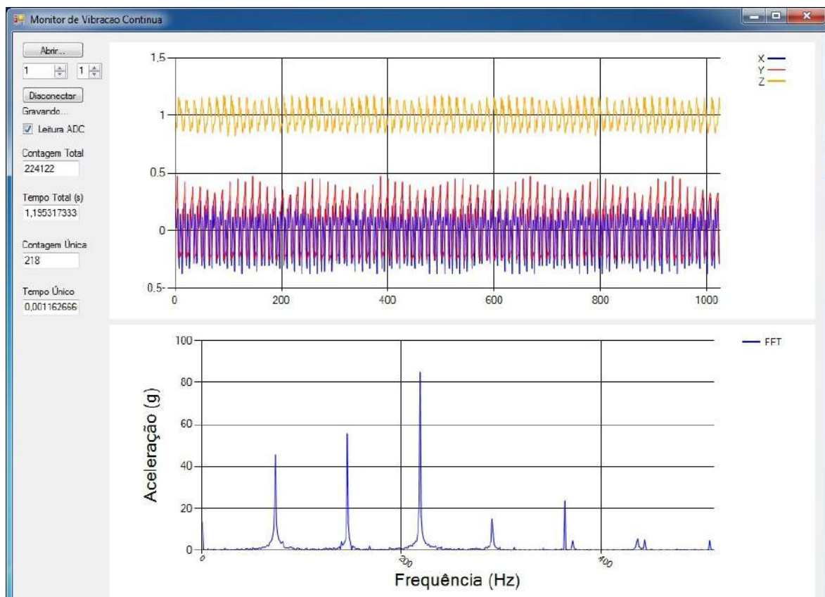
Figura 4.7: Espectro do eixo X para o motor DC de 12V à velocidade de 3641rpm.
