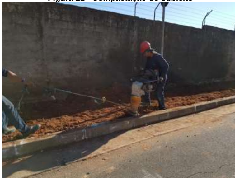
Figura 21 - Compactação do subleito
