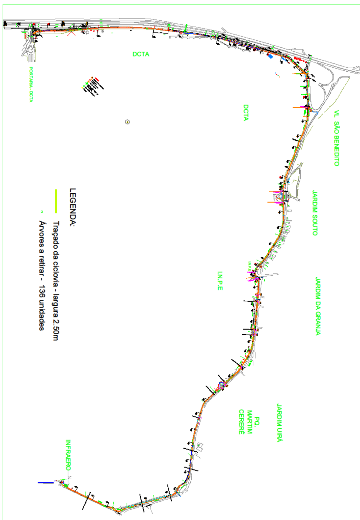
Figura 8 - Implantação da ciclovia
