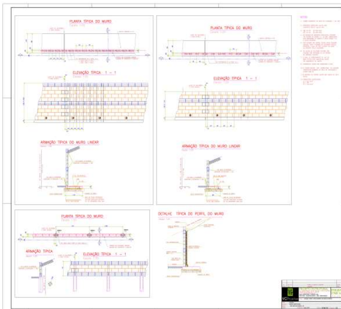
Figura 37 - Projeto referente aos muros de arrimo contratado com as obras iniciadas
