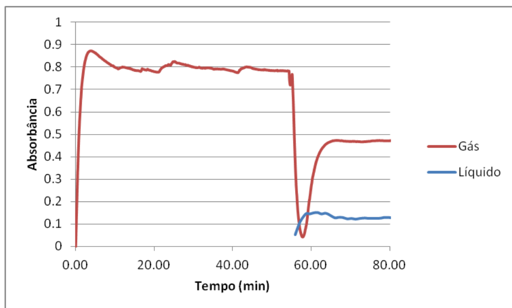
Figura 27 - Gráfico das medidas de absorbância a 254 nm para o experimento F.
