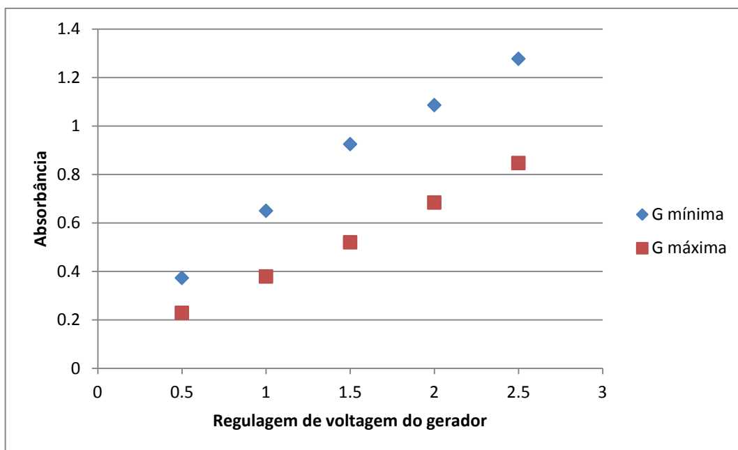
Figura 13 - Verificação da absorbância em relação à vazão do gás e voltagem do gerador.
