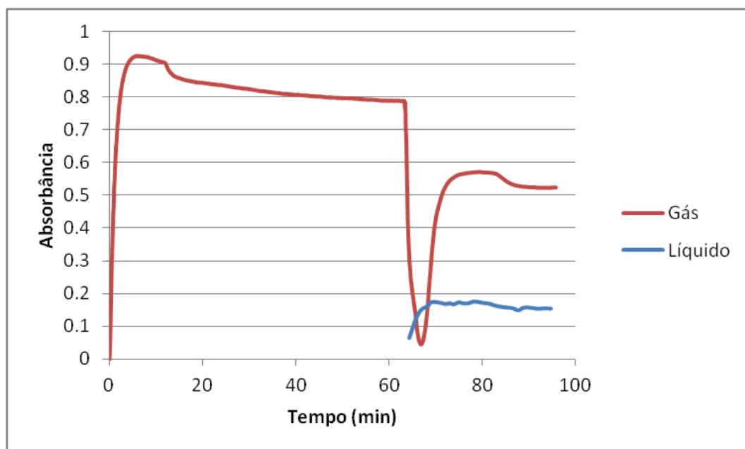
Figura 23 - Gráfico das medidas de absorbância a 254 nm para o experimento B.
