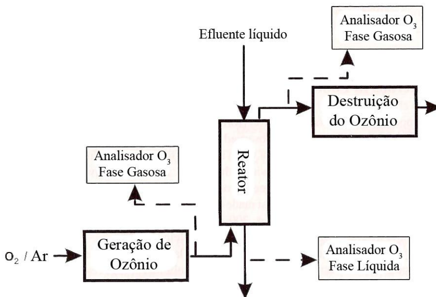
Figura 2 - Arranjo experimental básico. (Fonte: adaptado da referência 1)
