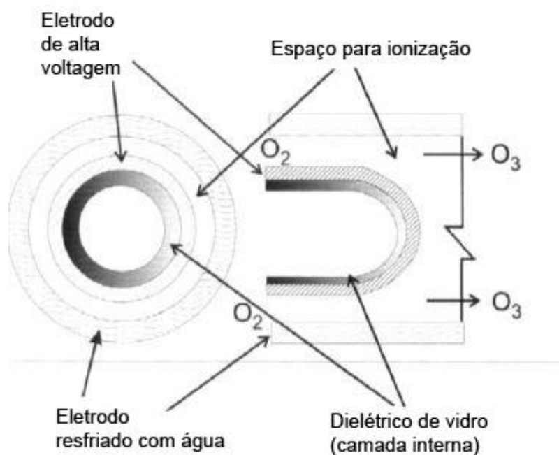
Figura 9 - Exemplo de gerador de ozônio por descarga elétrica tubular. (Fonte: adaptado da referência 1)
