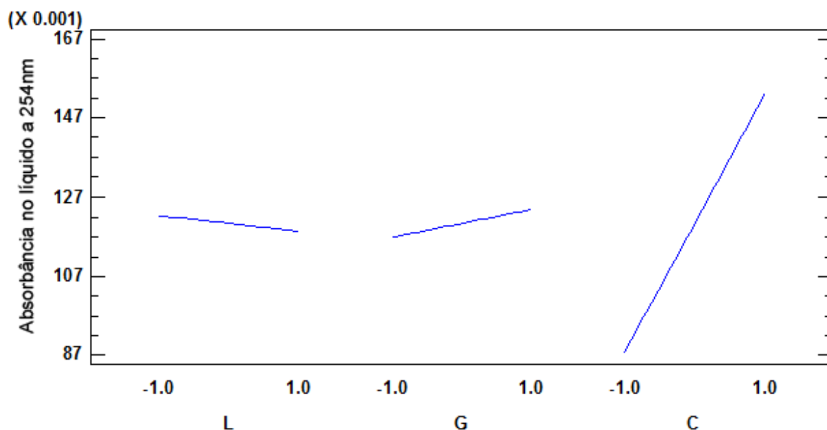
Figura 14 - Efeito das variáveis sobre a absorbância no líquido.
