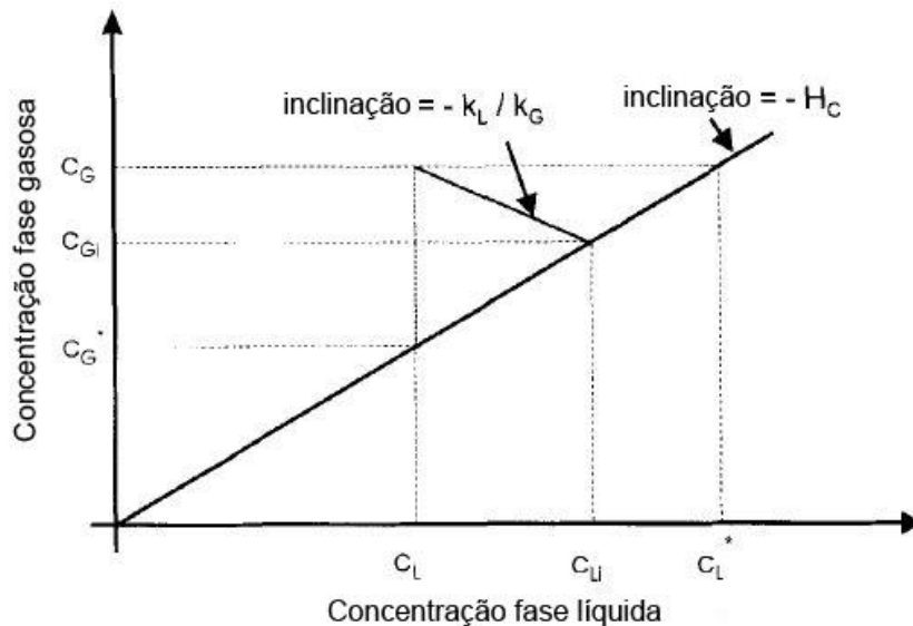
Figura 4 - Relação de equilíbrio entre fases. (Fonte: adaptado da referência 1)
