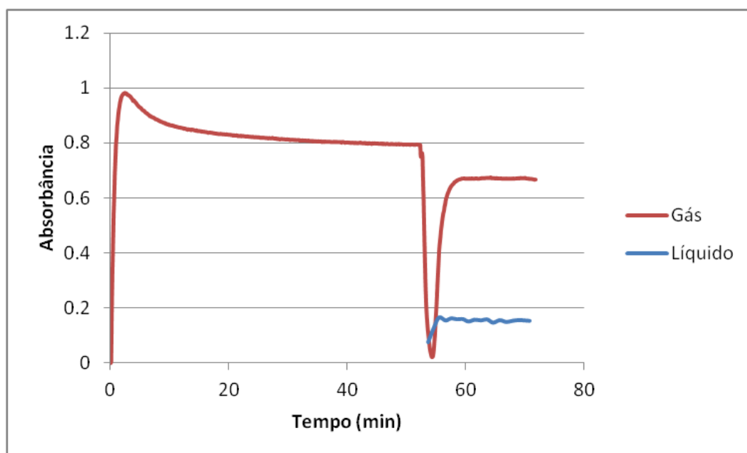
Figura 25 - Gráfico das medidas de absorvância a 254 nm para o experimento D.
