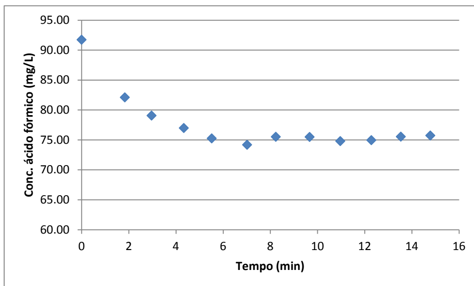
Figura 20 - Variação da concentração do ácido fórmico com o tempo para experimento N.
