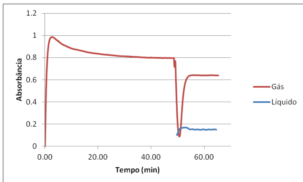
Figura 29 - Gráfico das medidas de absorvância a 254 nm para o experimento H.
