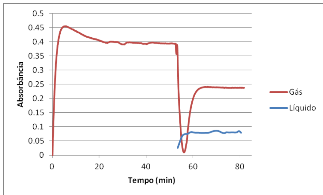
Figura 26 - Gráfico das medidas de absorbância a 254 nm para o experimento E.
