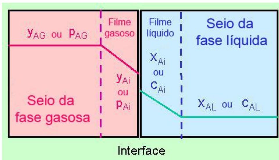
Figura 3 - Teoria do filme com gradiente linear de concentração. (Fonte: adaptado da referência 12)
