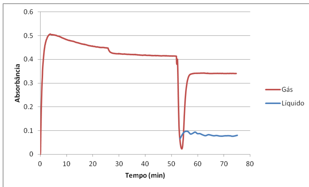
Figura 24 - Gráfico das medidas de absorvância a 254 nm para o experimento C.
