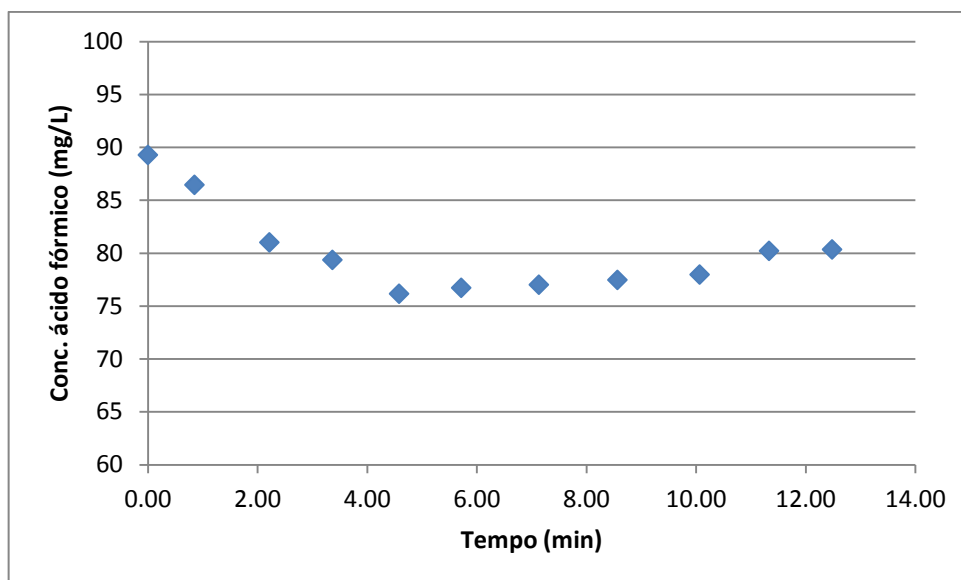
Figura 19 - Variação da concentração do ácido fórmico com o tempo para o experimento M.
