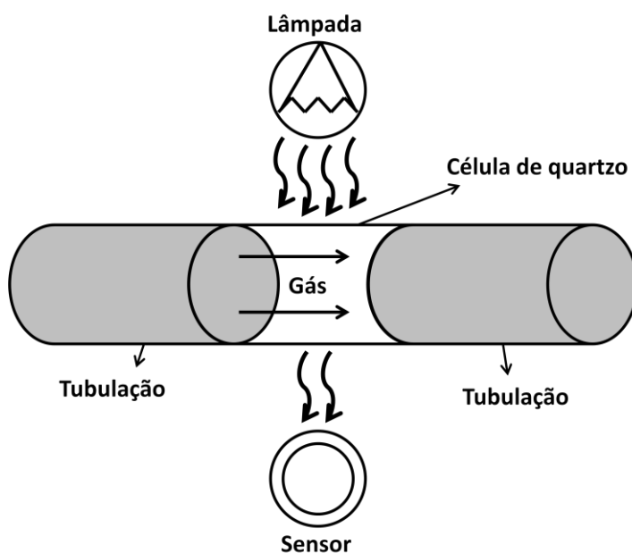
Figura 10 - Esquema simplificado da célula espectrofotométrica para gás.
