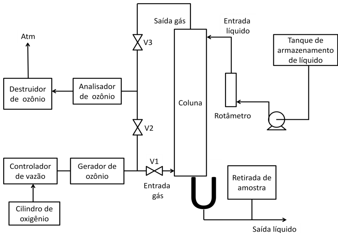
Figura 7 - Esquema simplificado do sistema.
