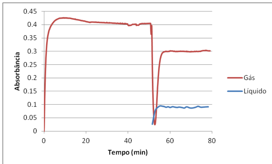
Figura 28 - Gráfico das medidas de absorvância a 254 nm para o experimento G.
