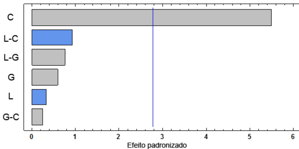
Figura 15 - Gráfico de pareto padronizado para os resultados experimentais.
