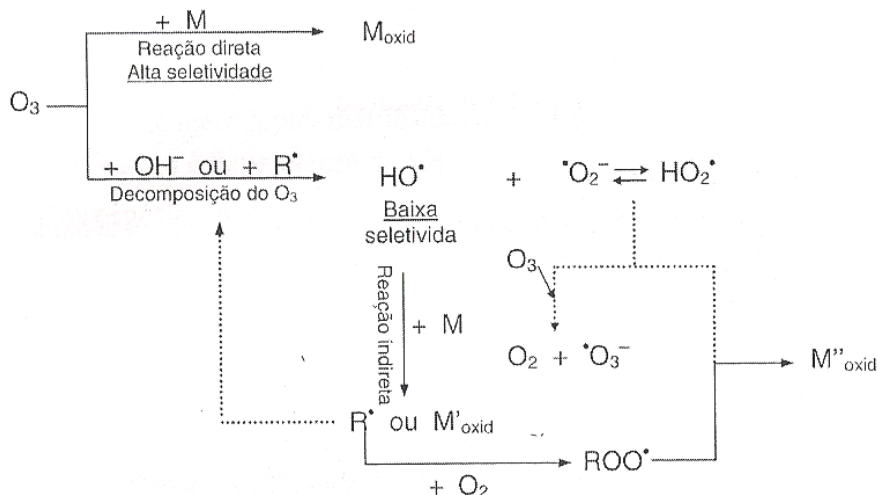
Figura 1 – Esquema de via de reações do ozônio. (Fonte: referência 8)
