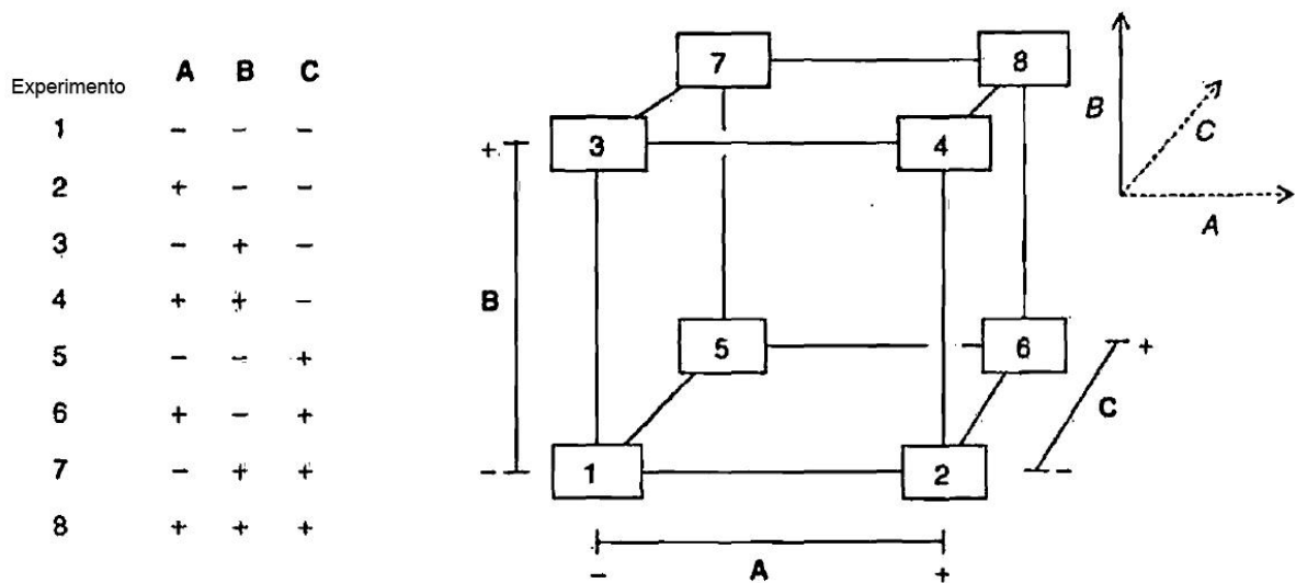
Figura 12 - Exemplo de experimentos fatoriais com 3 fatores. (Fonte: adaptado da referência 9)
