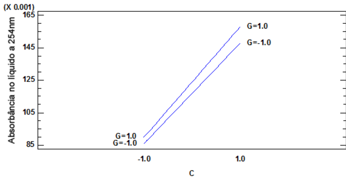
Figura 17 - Influência da interação entre G e C na absorbância do líquido.
