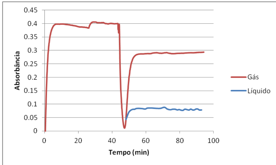
Figura 22 – Gráfico das medidas de absorbância a 254 nm para o experimento A.
