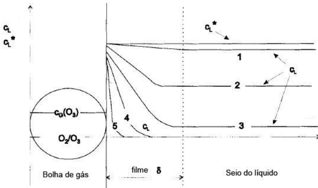
Figura 5 - Regimes cinéticos de transferência de massa com reação. (Fonte: adaptado da referência 1)
