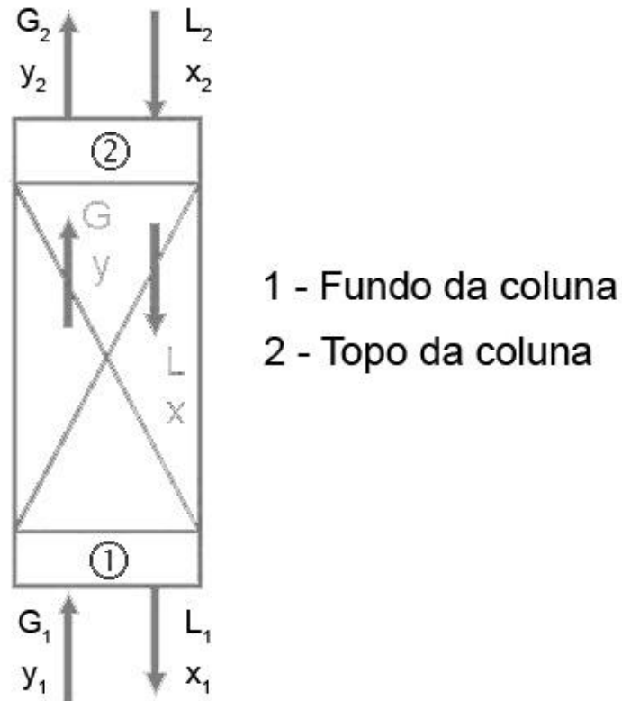
Figura 6 - Esquema de uma coluna de enchimento. (Fonte: adaptado da referência 12)
