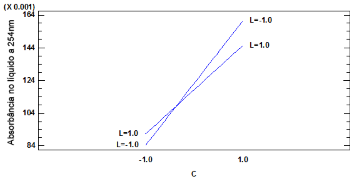
Figura 16 - Influência da interação entre L e C na absorbância do líquido.
