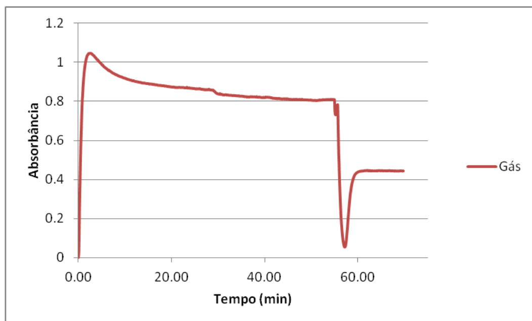
Figura 33 - Gráfico das medidas de absorvância a 254 nm para o experimento M.
