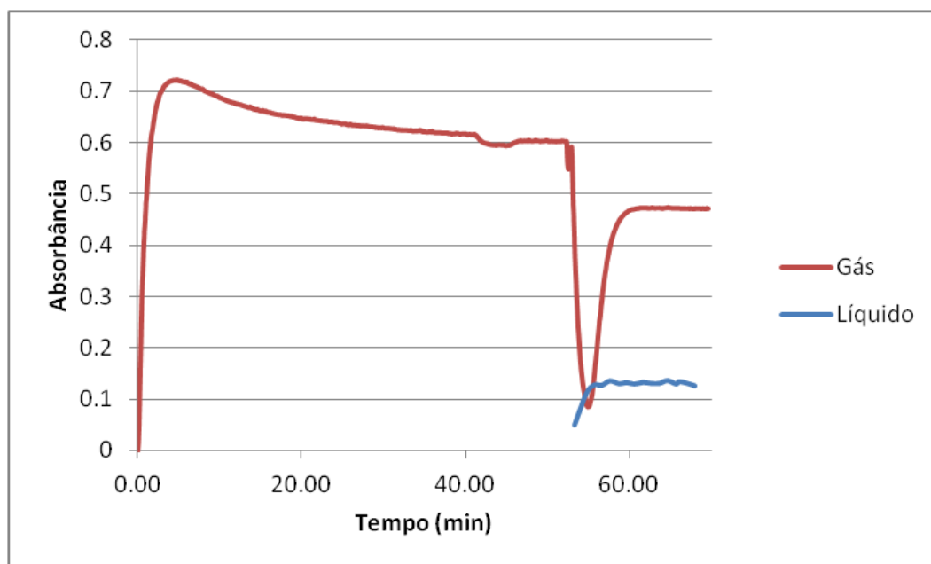
Figura 30 - Gráfico das medidas de absorvância a 254 nm para o experimento I.
