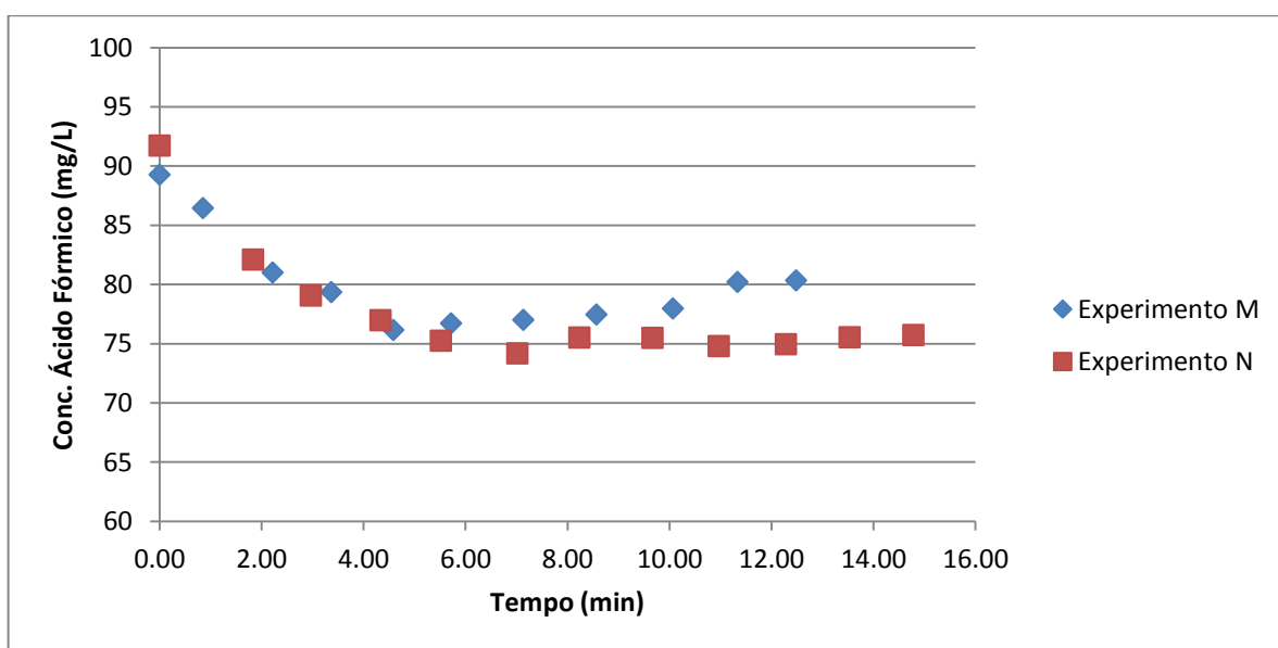
Figura 21 - Comparação entre os experimentos de degradação de ácido fórmico.
