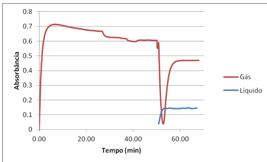
Figura 31 - Gráfico das medidas de absorvância a 254 nm para o experimento J.
