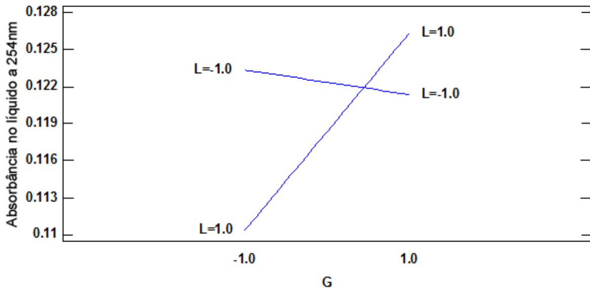
Figura 18 - Influência da interação entre L e G na absorbância do líquido.
