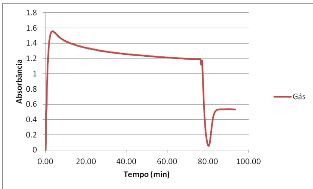
Figura 34 - Gráfico das medidas de absorbância a 254 nm para o experimento N.
