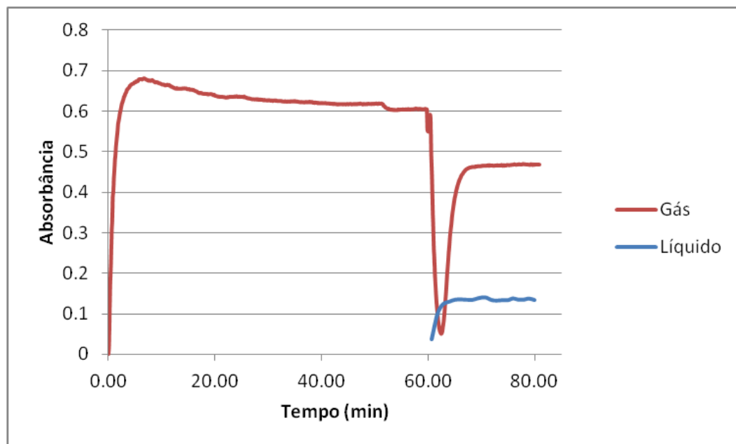
Figura 32 - Gráfico das medidas de absorvância a 254 nm para o experimento L.
