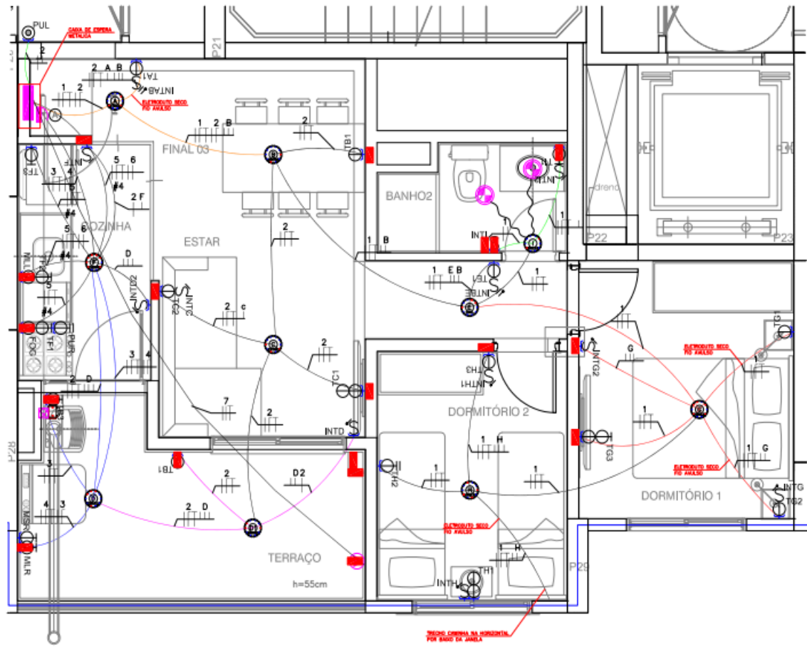
Figura 3 - Planta elétrica do apartamento de 55m 2
