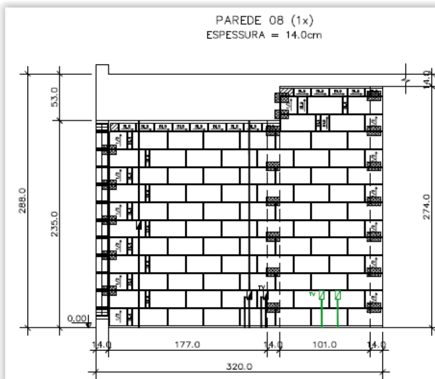
Figura 13 – Elevação com a disposição das caixas elétricas
