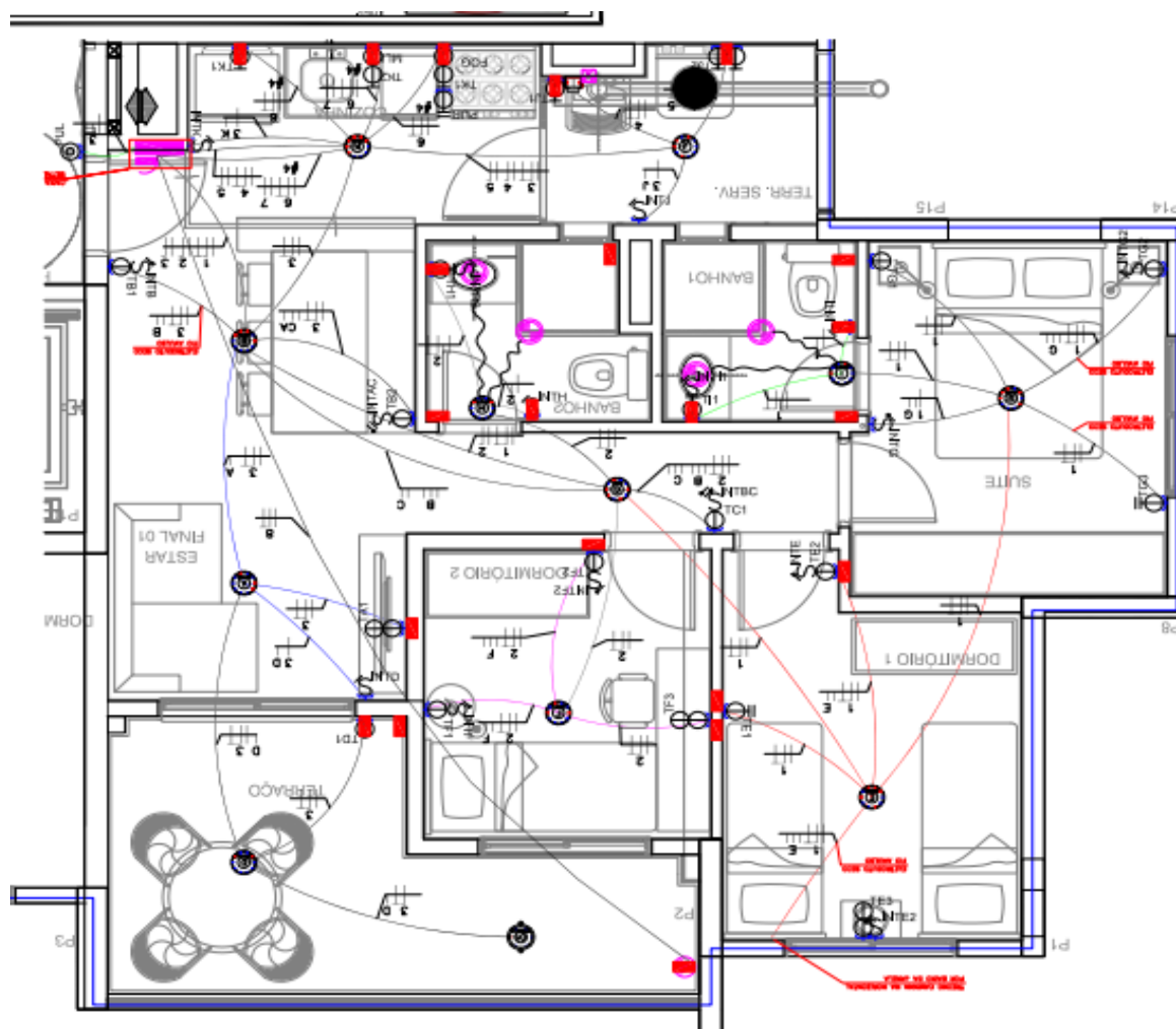
Figura 4 - Planta elétrica do apartamento de 70m 2
