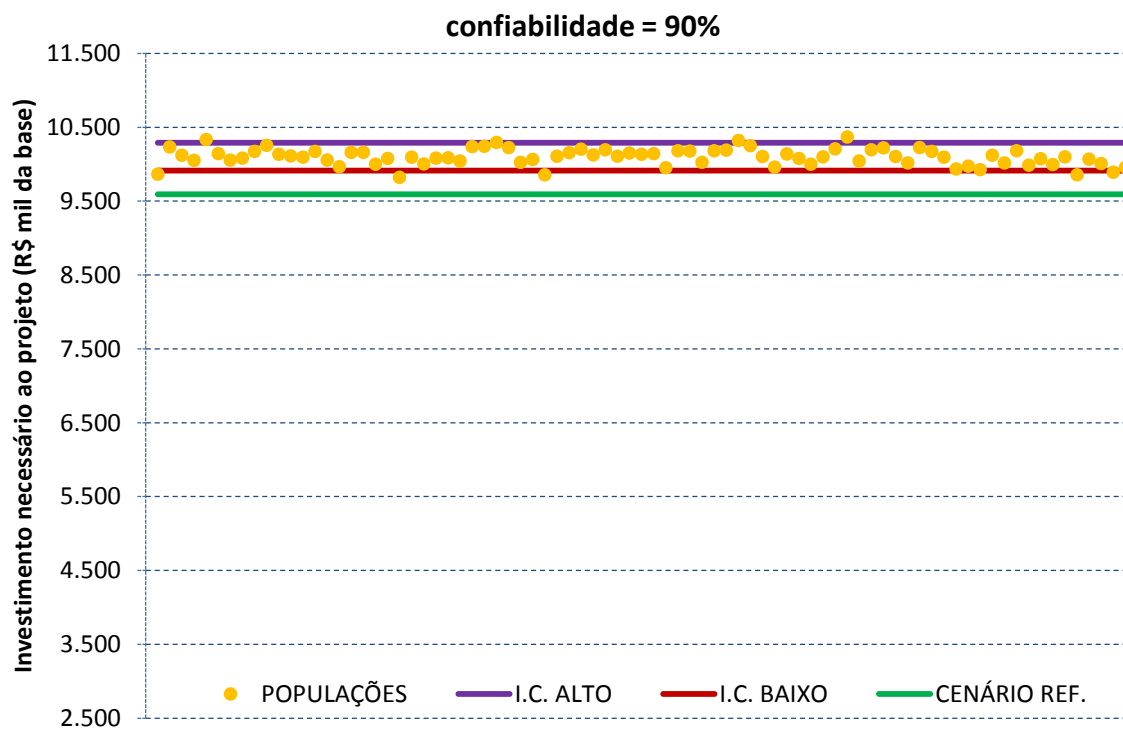
Gráfico 24: Efeitos no Investimento com a flutuação das variáveis preço e custo - caso [ii]
