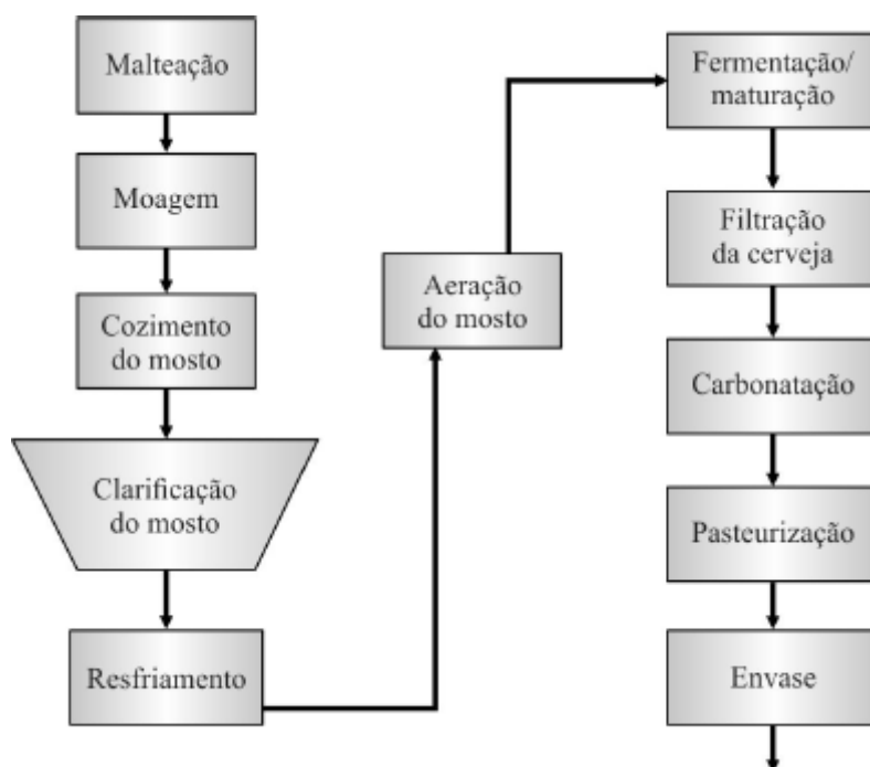
Figura 2 – Diagrama de blocos do processo de produção de cerveja.
