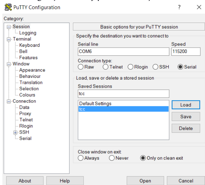
Figura 8 – Configuração do PuTTY para comunicação serial com a Edison.
