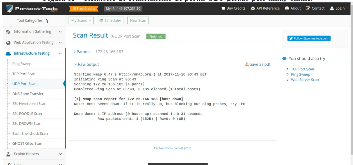
Figura 15 – Relatório de scaneamento de portas UDP gerado pelo nmap online.
