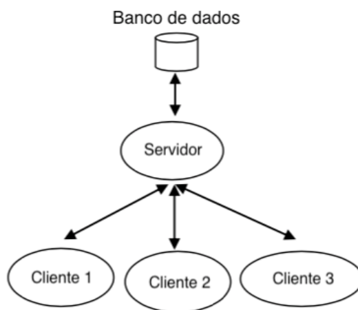
Figura 6 - Arquitetura cliente-servidor.
