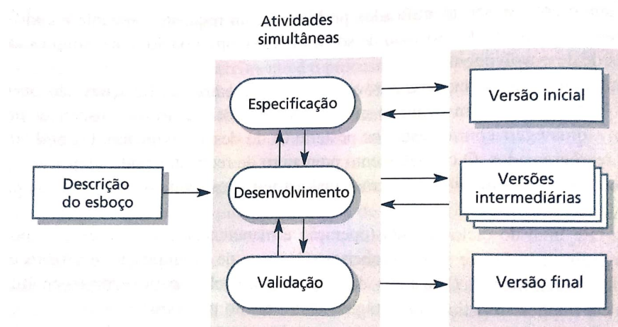
Figura 2 - Modelo Evolucionário.
