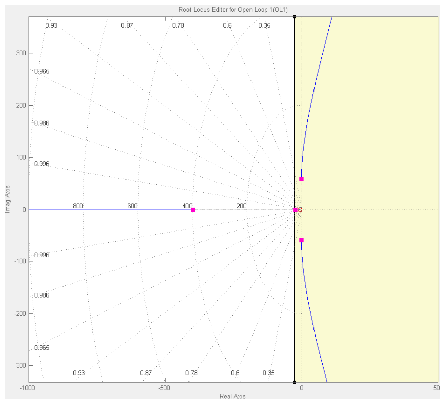
Figura 9: Lugar das Raízes - Sistema C(s)*G(s)
