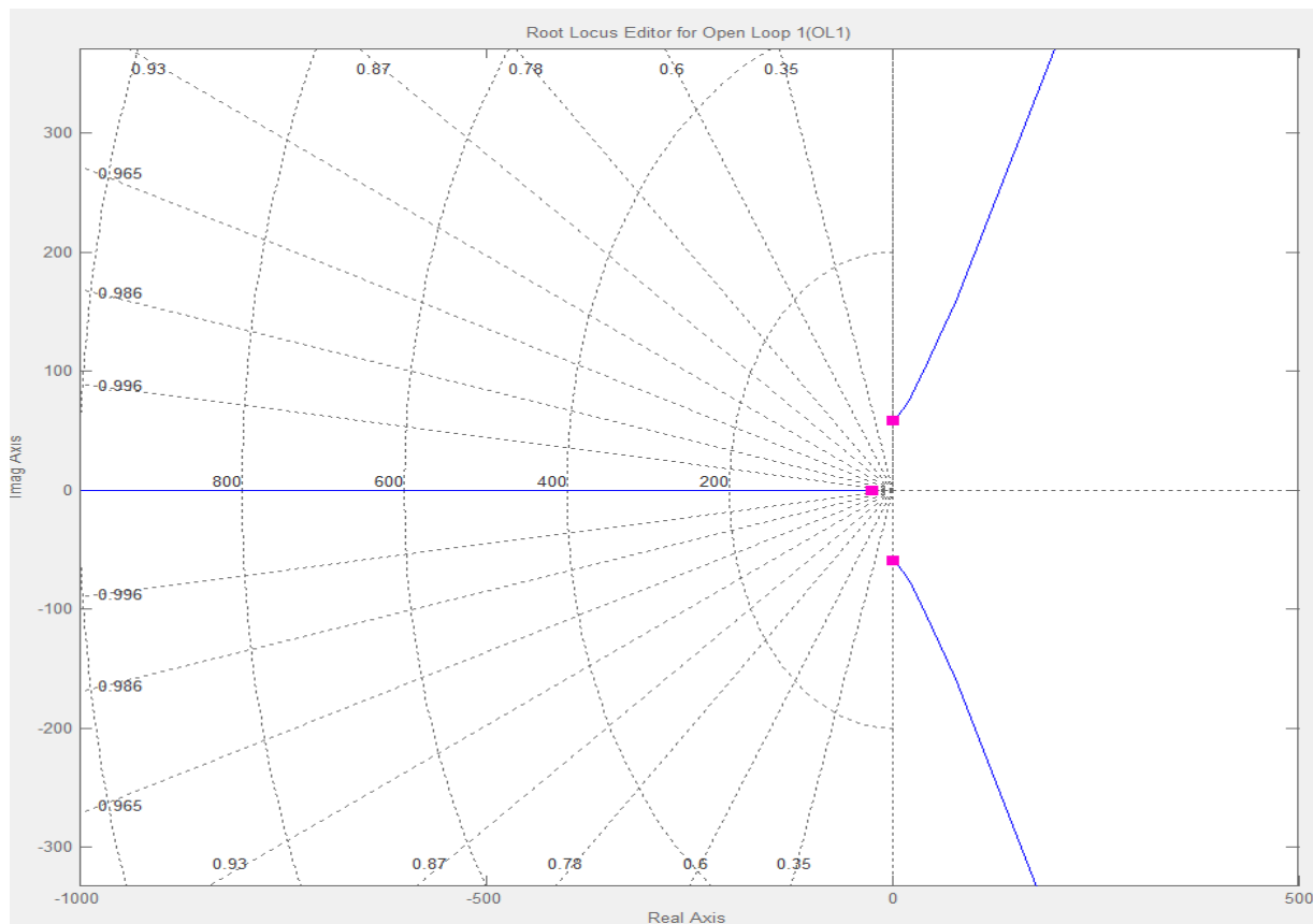
Figura 7: Lugar das Raízes do sistema não compensado
