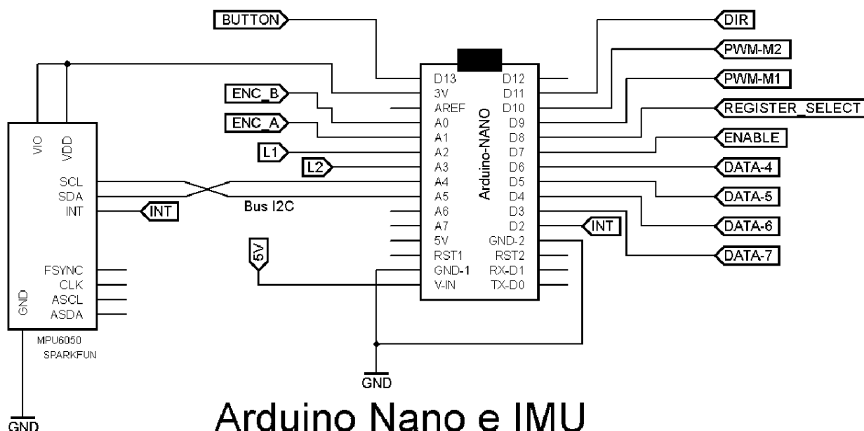
Figura 30 - Esquemático do circuito do microprocessador, com sinais listados.
