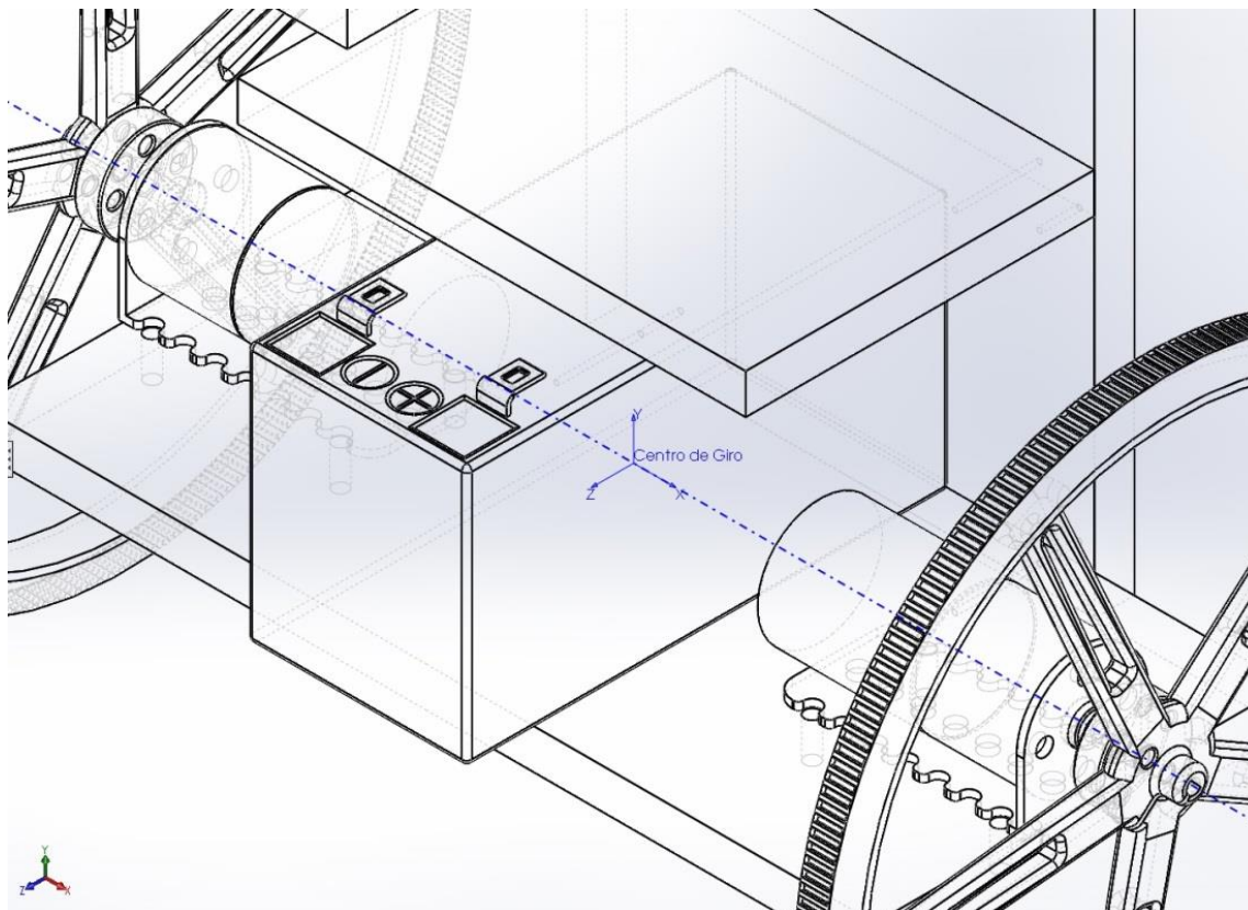
Figura 2: Sistema de coordenadas adotado para o cálculo da posição espacial do CG da planta
