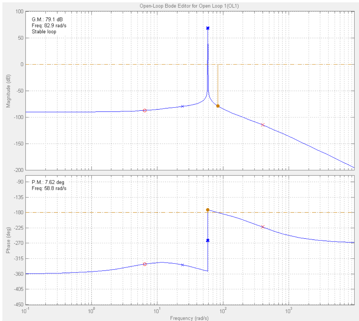
Figura 10: Diagrama de Bode - Sistema C(s)*G(s)
