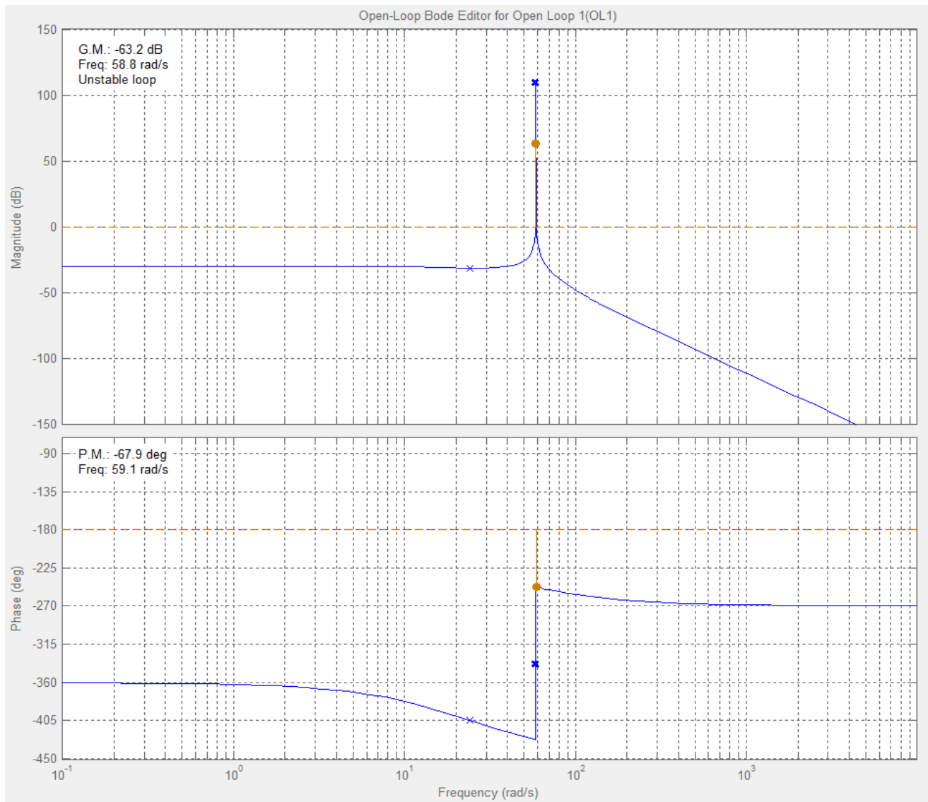
Figura 8: Diagrama de Bode do sistema não compensado
