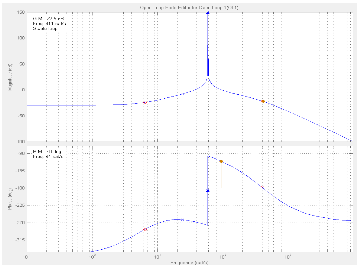
Figura 15: Diagrama de Bode do Sistema C(s)*C2(s)*G(s)
