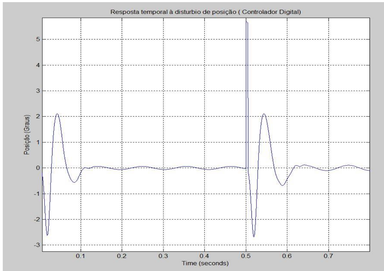
Figura 21 - Resposta temporal do sistema com Controlador digital
