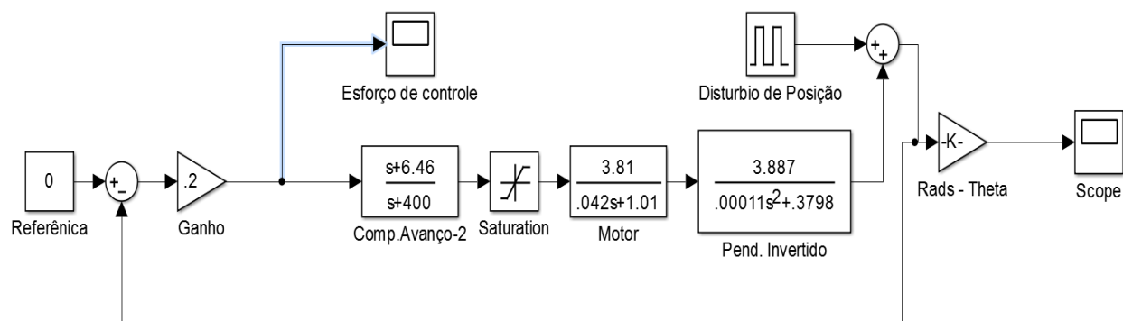
Figura 11: Malha de Controle em Simulink para Simulação
