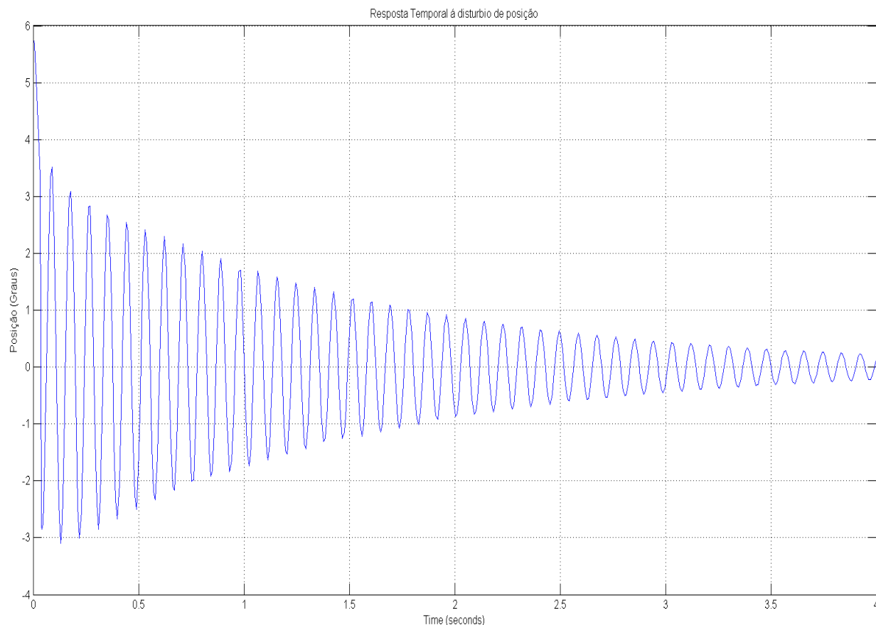
Figura 12: Resposta temporal do sistema C(s)G(s) à distúrbio de posição
