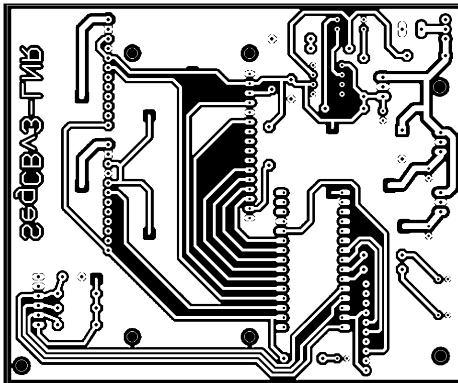
Figura 39 - Roteamento de trilhas na placa de circuito impresso
