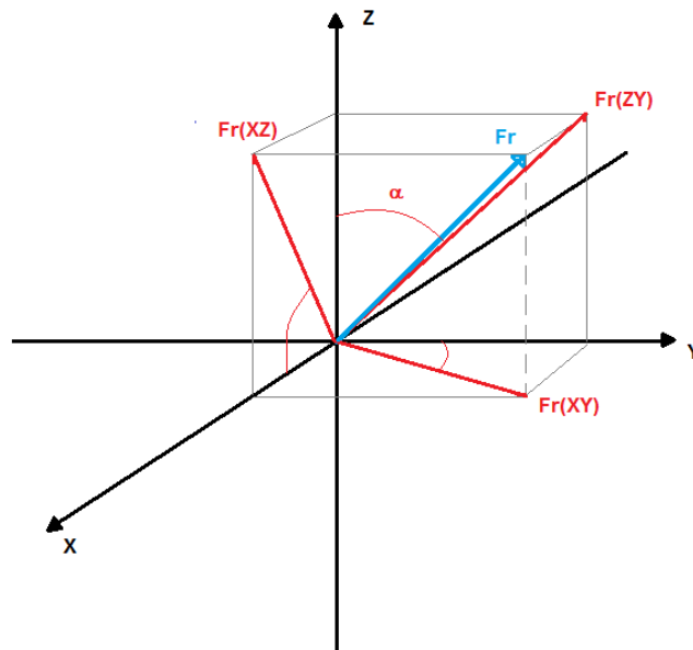
Figura 22 - Força arbitrária aplicada sobre um acelerômetro de três eixos e suas componentes nos planos coordenados
