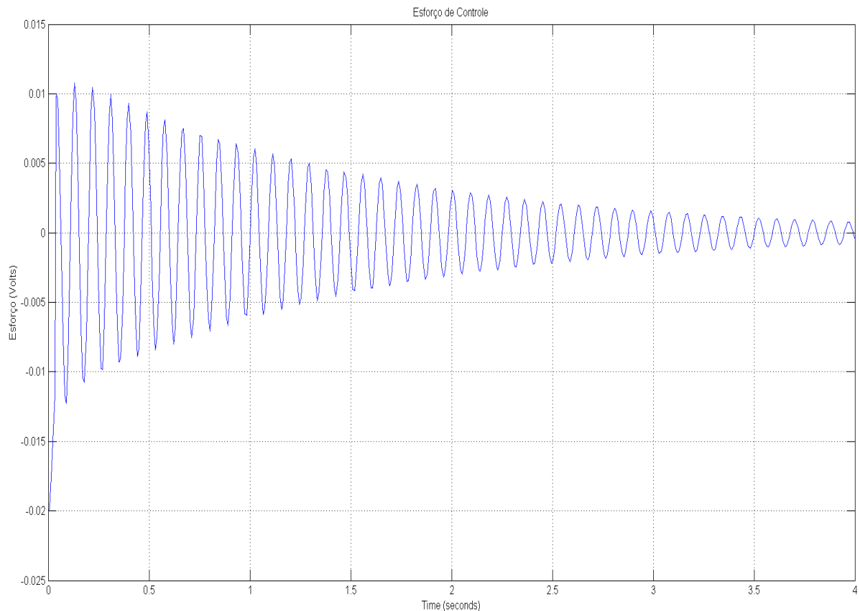
Figura 13: Esforço de Controle do Sistema C(s) \cdot G(s)
