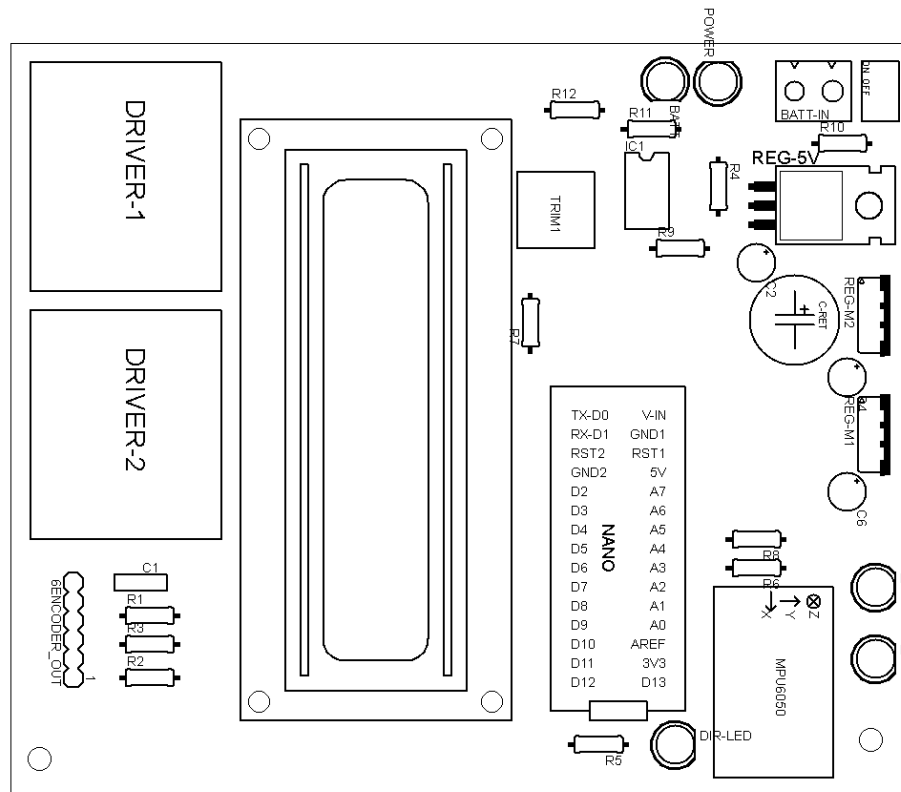
Figura 38 - Disposição de componentes na placa de circuito impresso
