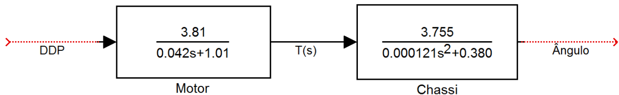
Figura 6: Diagrama de blocos em malha aberta do sistema Motor-Chassi
