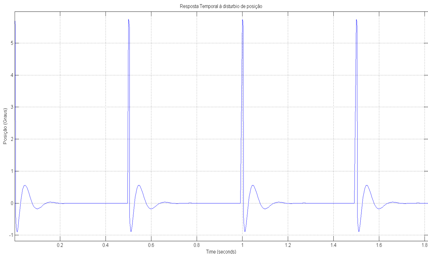
Figura 17: Resposta temporal à distúrbio de posição do sistema C(s)*C2(s)*G(s)
