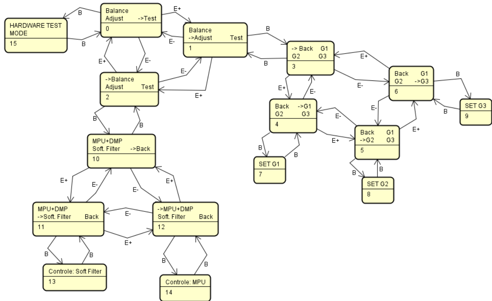
Figura 29 - Máquina de estados e sistema de menus.
