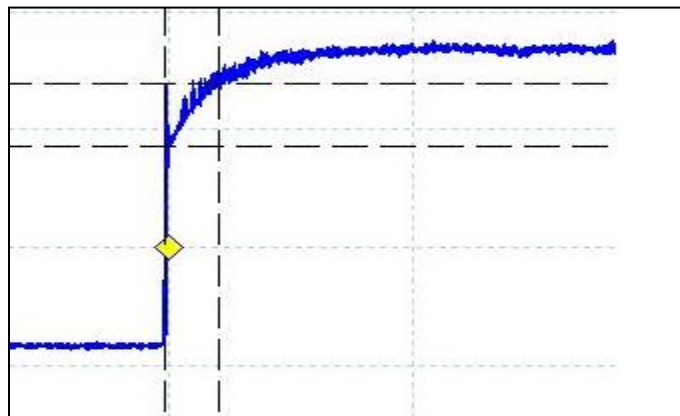
Figura 5: Resposta temporal transitória de voltagem nos terminais do motor, 200ms por divisão, T = 42ms.
