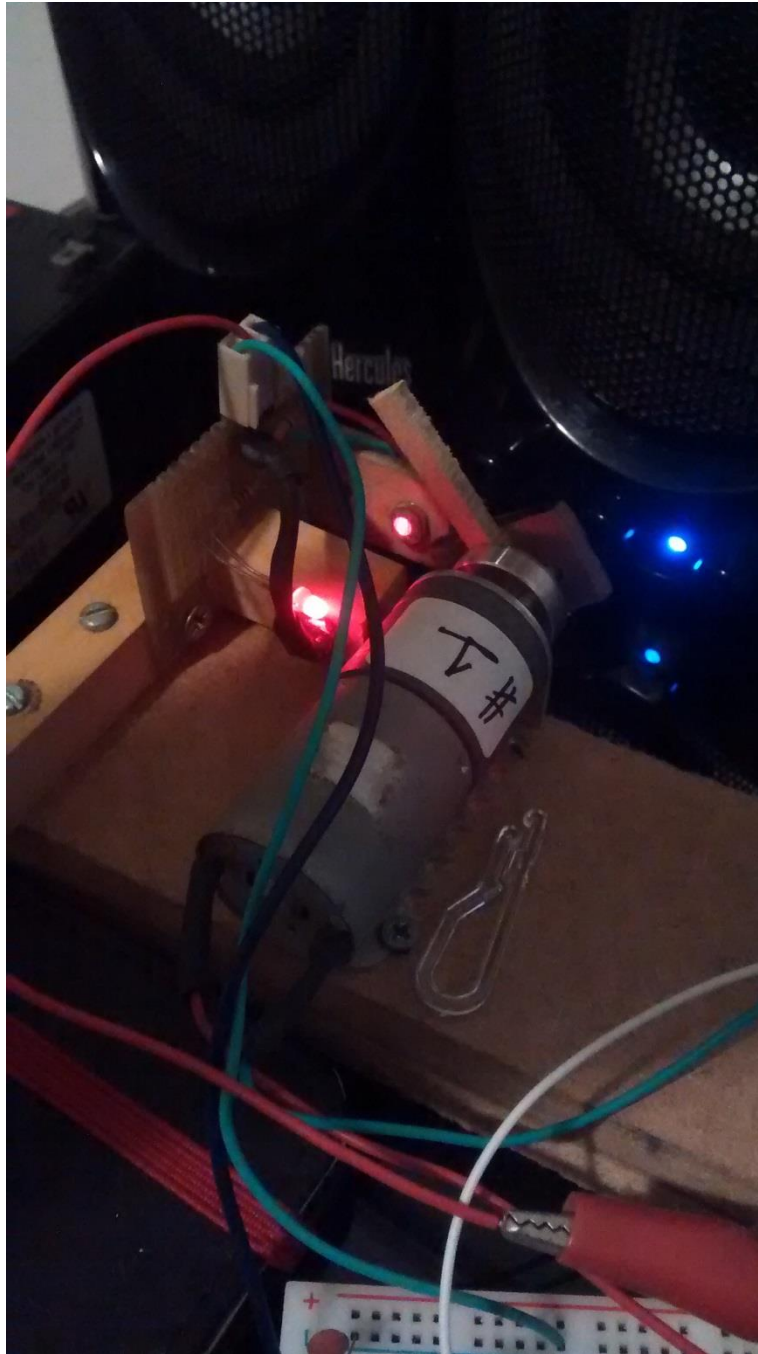
Figura 41: Tacômetro improvisado para medição da velocidade angular do motor em regime. Um diodo Laser e um divisor de tensão usando um LDR geram pulsos de tensão a cada vez que o Laser é interrompido (Maio de 2015)
