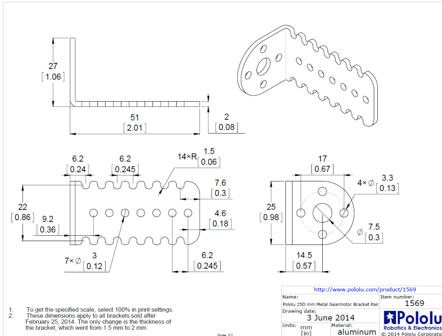
Figura 26: Bracket utilizado na fixação do motor ao chassi
