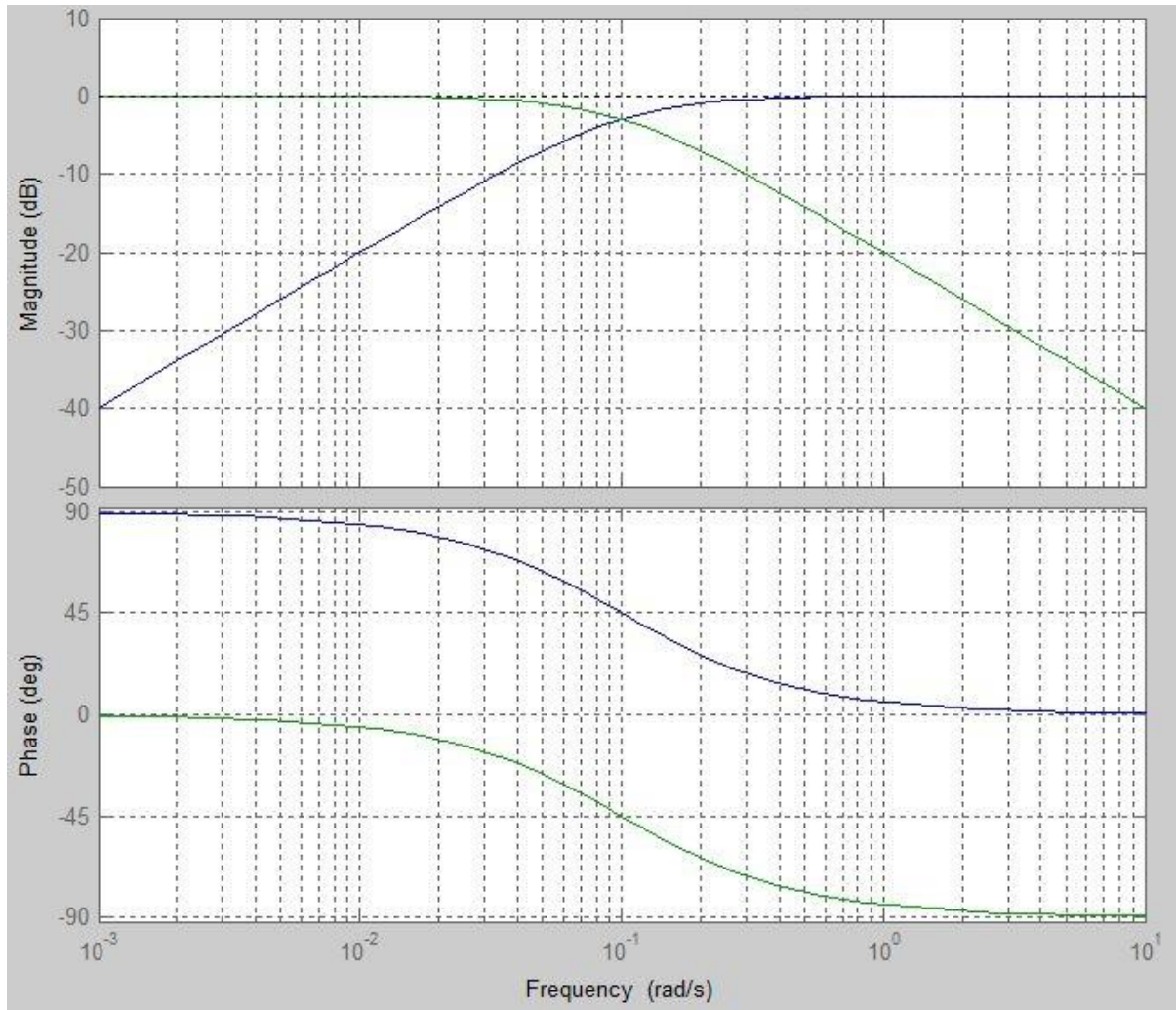
Figura 23 - Resposta em frequência de um filtro complementar típico
