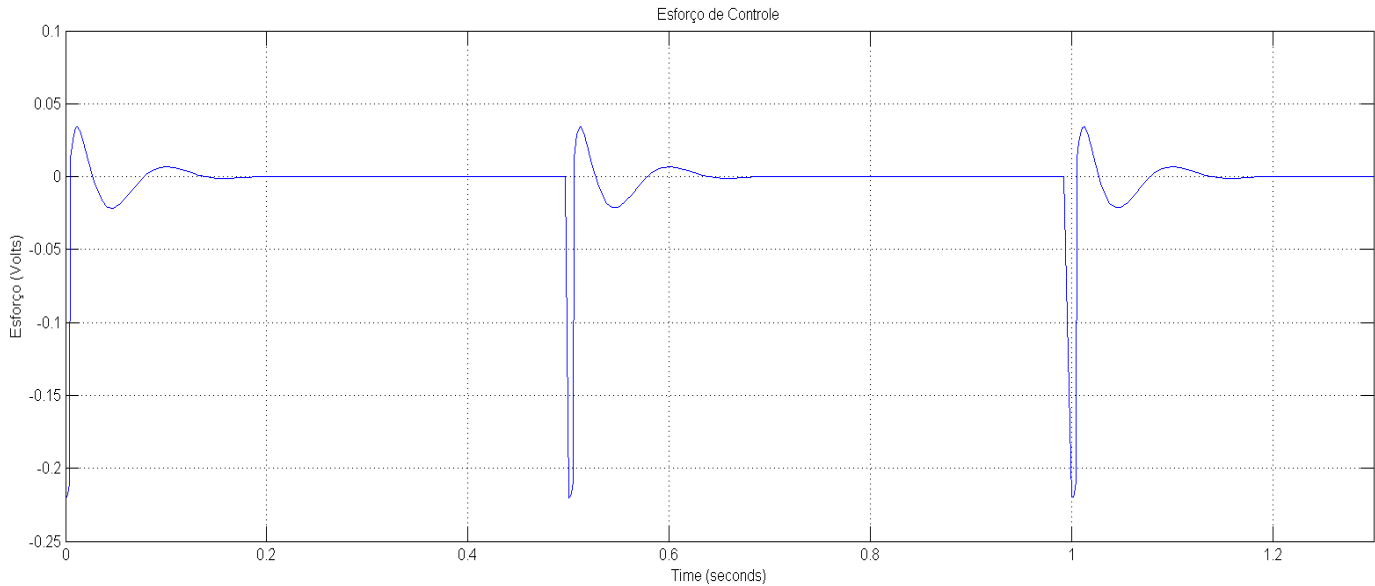
Figura 19: Esforço de controle para o sistema C(s)*C2(s)*G(s)
