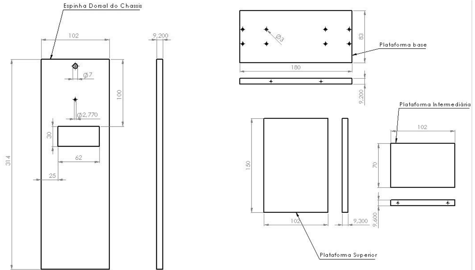
Figura 28: Estrutura em Tauari do chassi e dimensões
