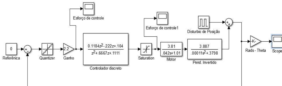
Figura 20: Malha de controle para Controlador discreto C(z)
