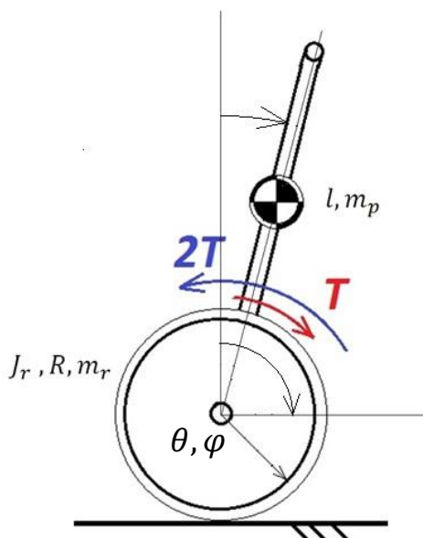
Figura 4 - Planta dinâmica usada para modelar o sistema
