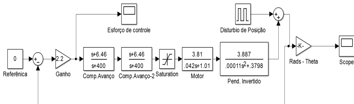
Figura 16: Malha de controle em Simulink para simulação do sistema C(s)*C2(s)*G(s)
