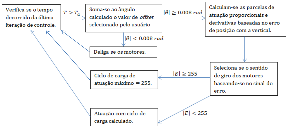
Figura 25 - Fluxograma de cálculo de esforço de controle E baseado no ângulo instantâneo com a vertical \theta
