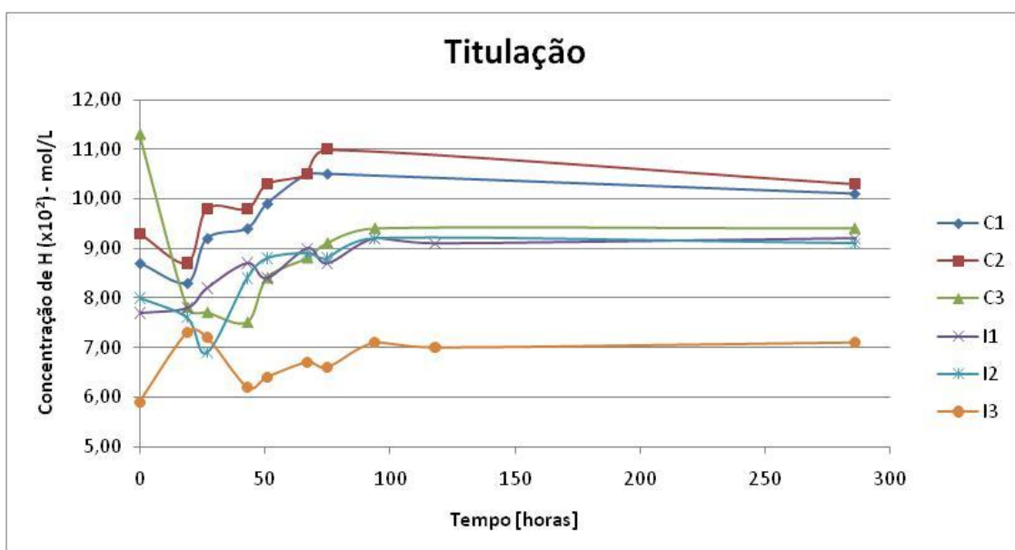
Gráfico 19 – Curvas de acidez total dos vinhos
