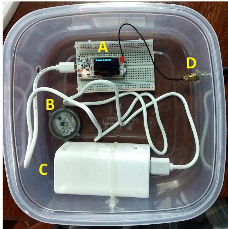
Figura 17: Estação coletora utilizada nos testes.
