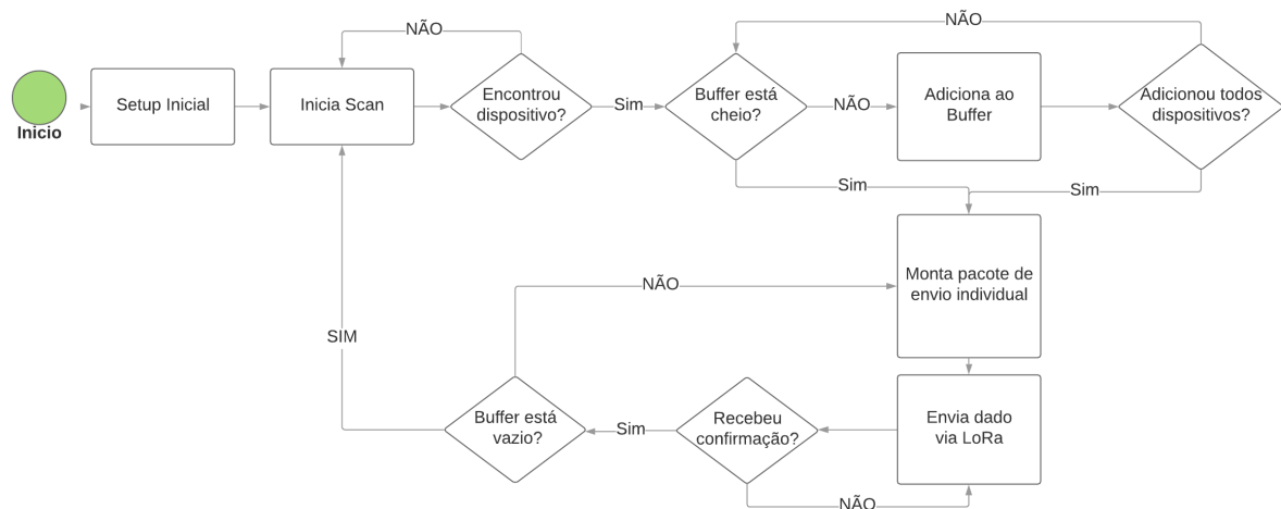
Figura 12: Fluxograma do software da estação coletora.
