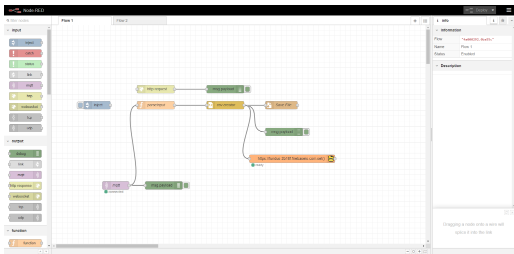
Figura 6: Página principal da ferramenta Node-RED
