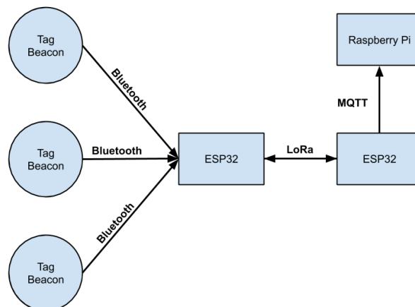
Figura 11: Diagrama do sistema
