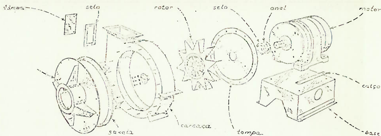
Fig.V.13 - Componentes de um ventilador.
