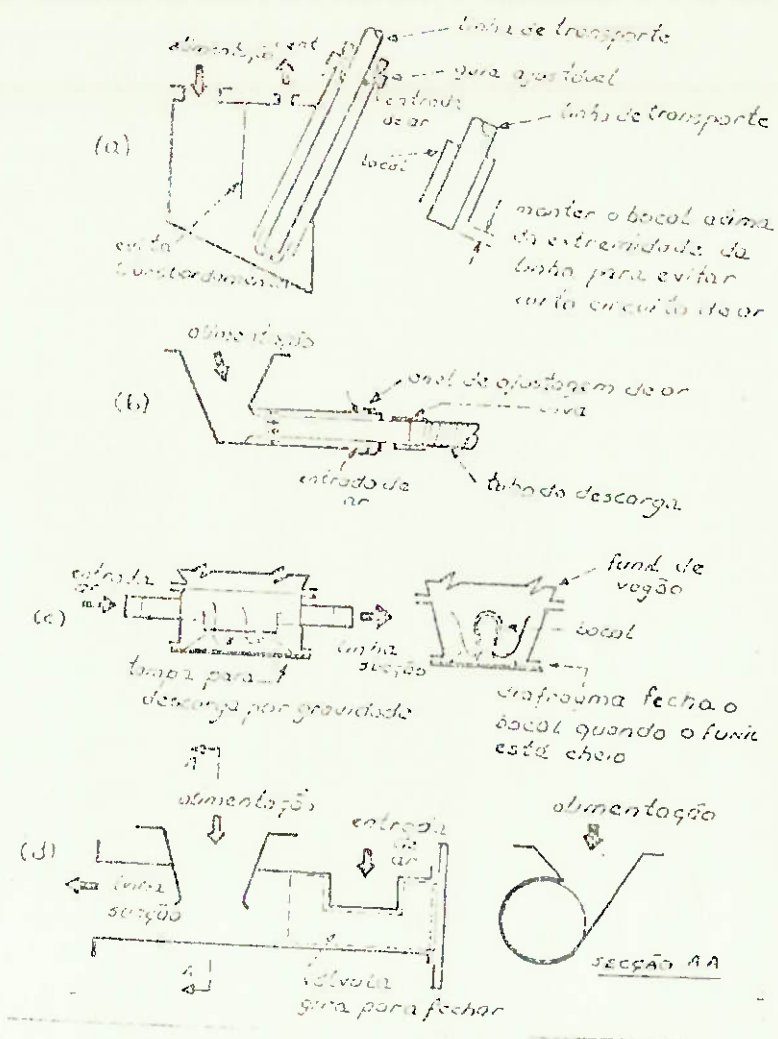
Fig.IV.1 - Vários arranjos de alimentação para sistema a vácuo.
