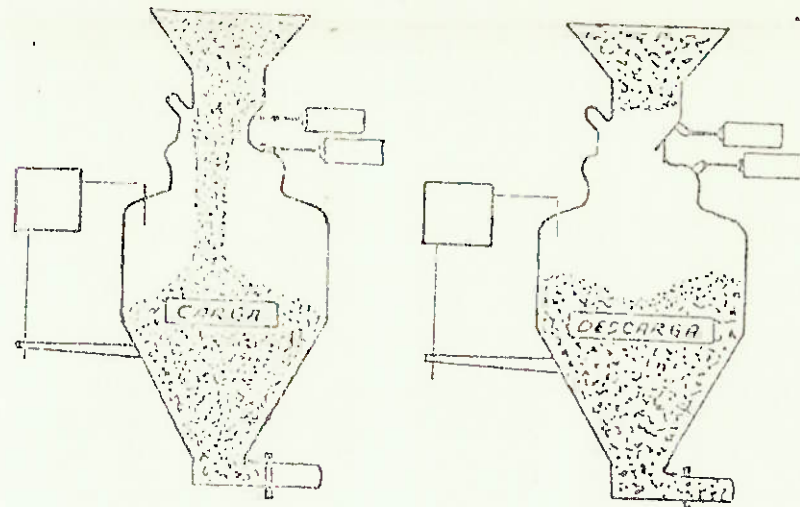
Fig. II.13 - Ilustração do ciclo de um "blow-tank".
