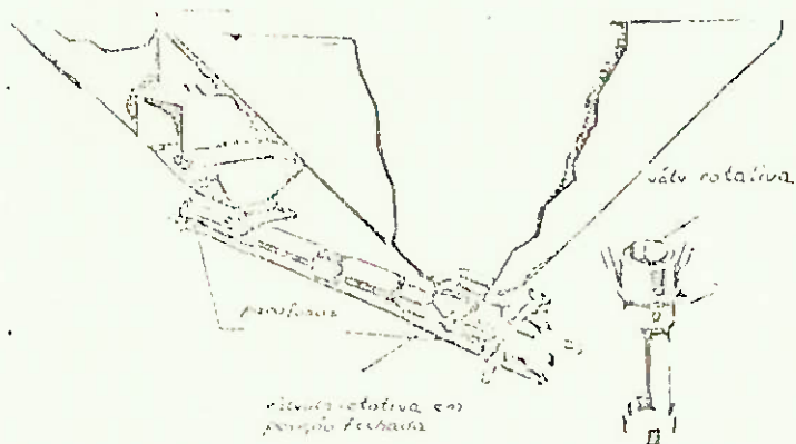
Fig.IV.30 - Válvula rotativa para descarga pneumática à vácuo.
