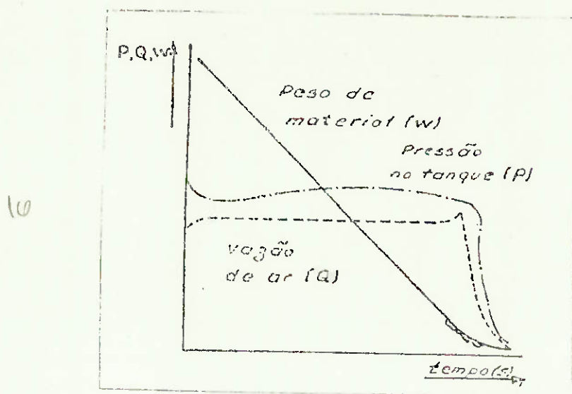
Fig. II.15 - Ciclo de um "blow-tank" c/alimentação controlada.
