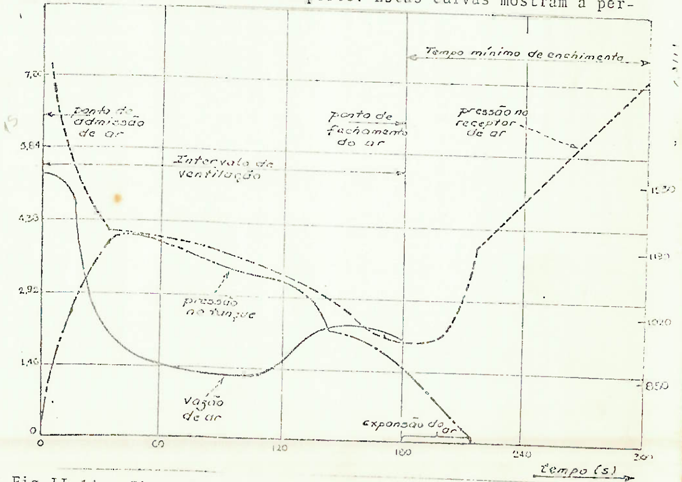
Fig.II.14 - Ciclo de operação de um "blow-tank" de alta pressão.
