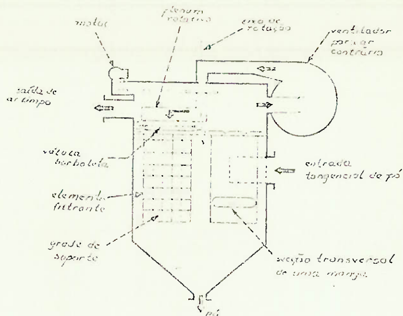
Fig.IV.22 - Filtro de pó com ar contrário a baixa pressão.
