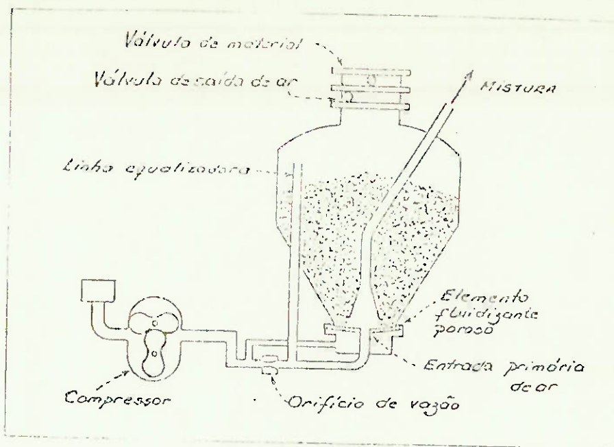
Fig. II.11 - "Blow-tank" de baixa pressão.
