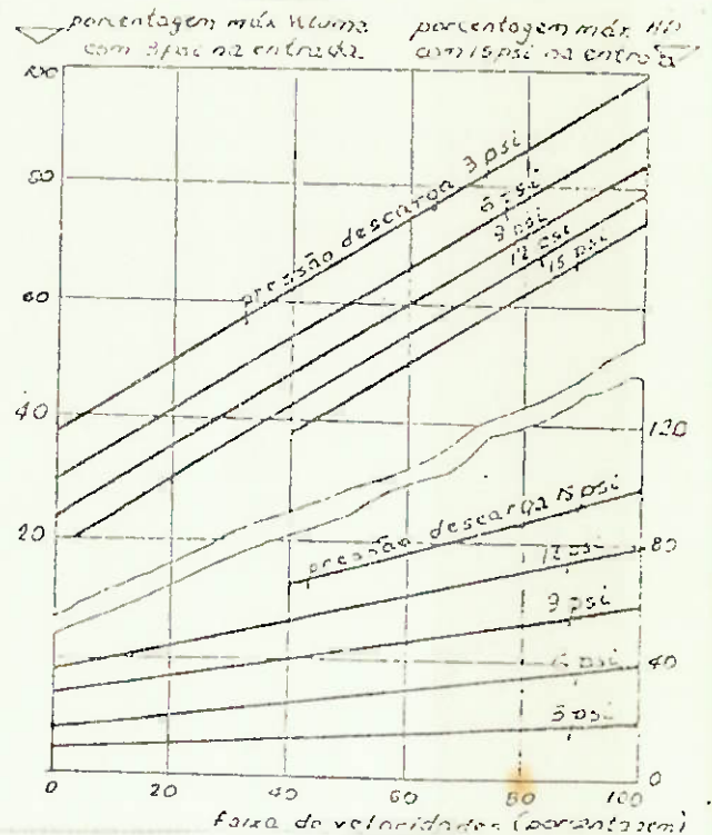
Fig.V.3 - Curva de performance de um soprador de deslocamento positivo.
