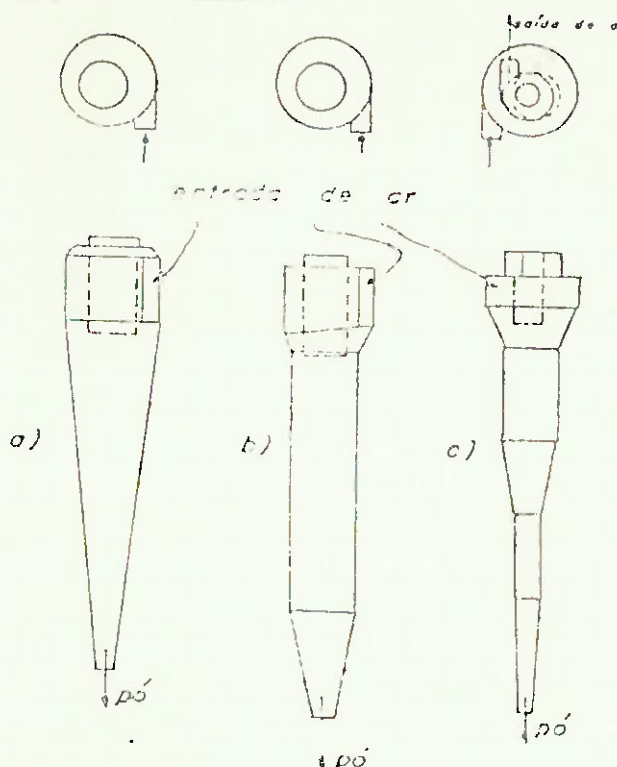
Fig.IV.15 - Ciclones de pequeno diâmetro.
