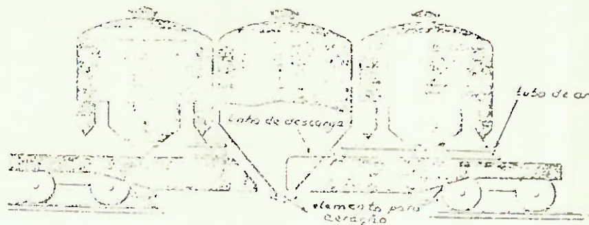
Fig.IV.27 - Carro-vagão com tanques pressurizados compartimentados.
