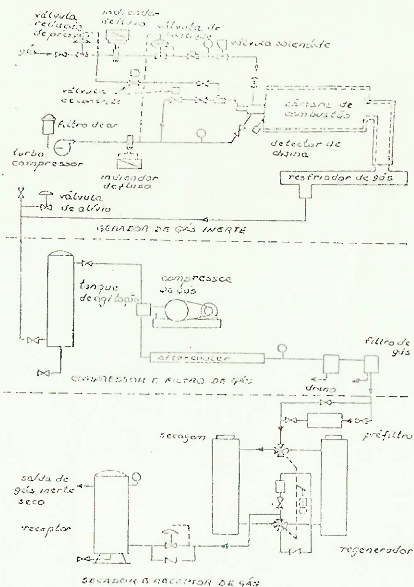
Fig.V.15 - Fluxograma de um sistema de geração de gás inerte a alta pressão.
