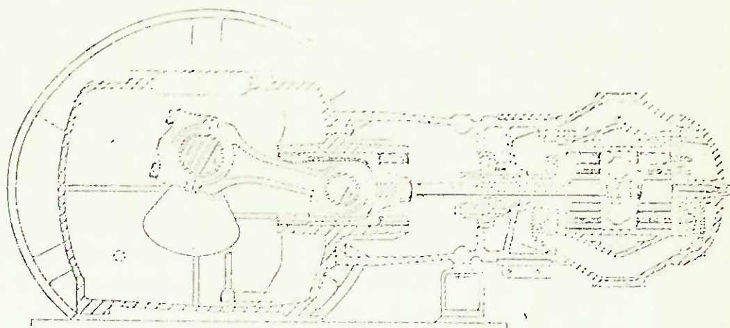
Fig.V.10 -- Compressor alternativo resfriado a água.
