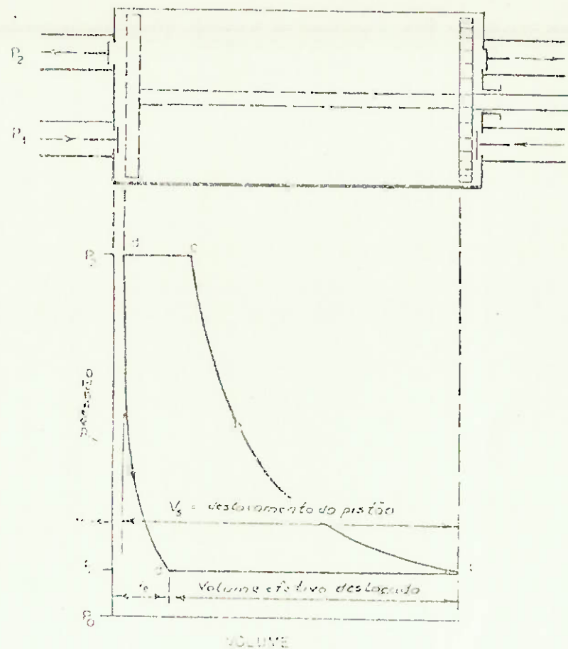
Fig.V.11 - Diagrama de um ciclo ideal de funcionamento de um compressor alternativo.
