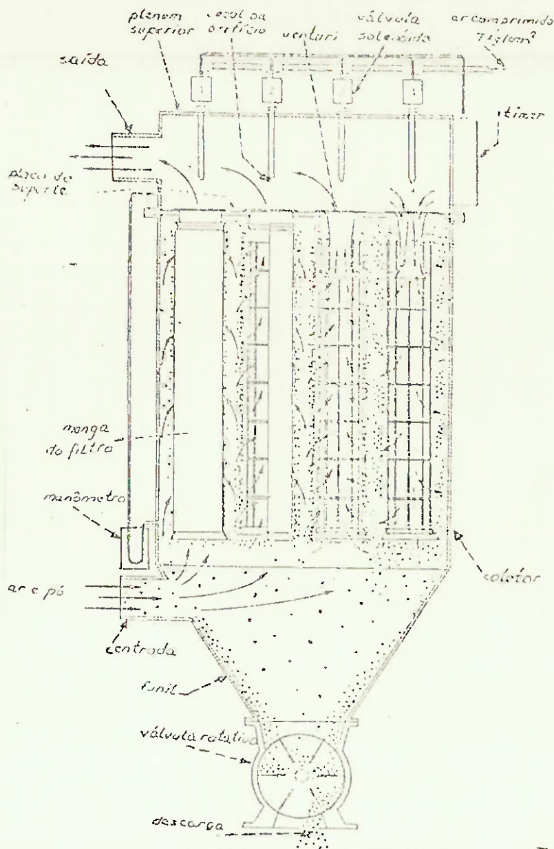
Fig.IV.21 - Filtro de pó com ar contrário a baixa pressão.
