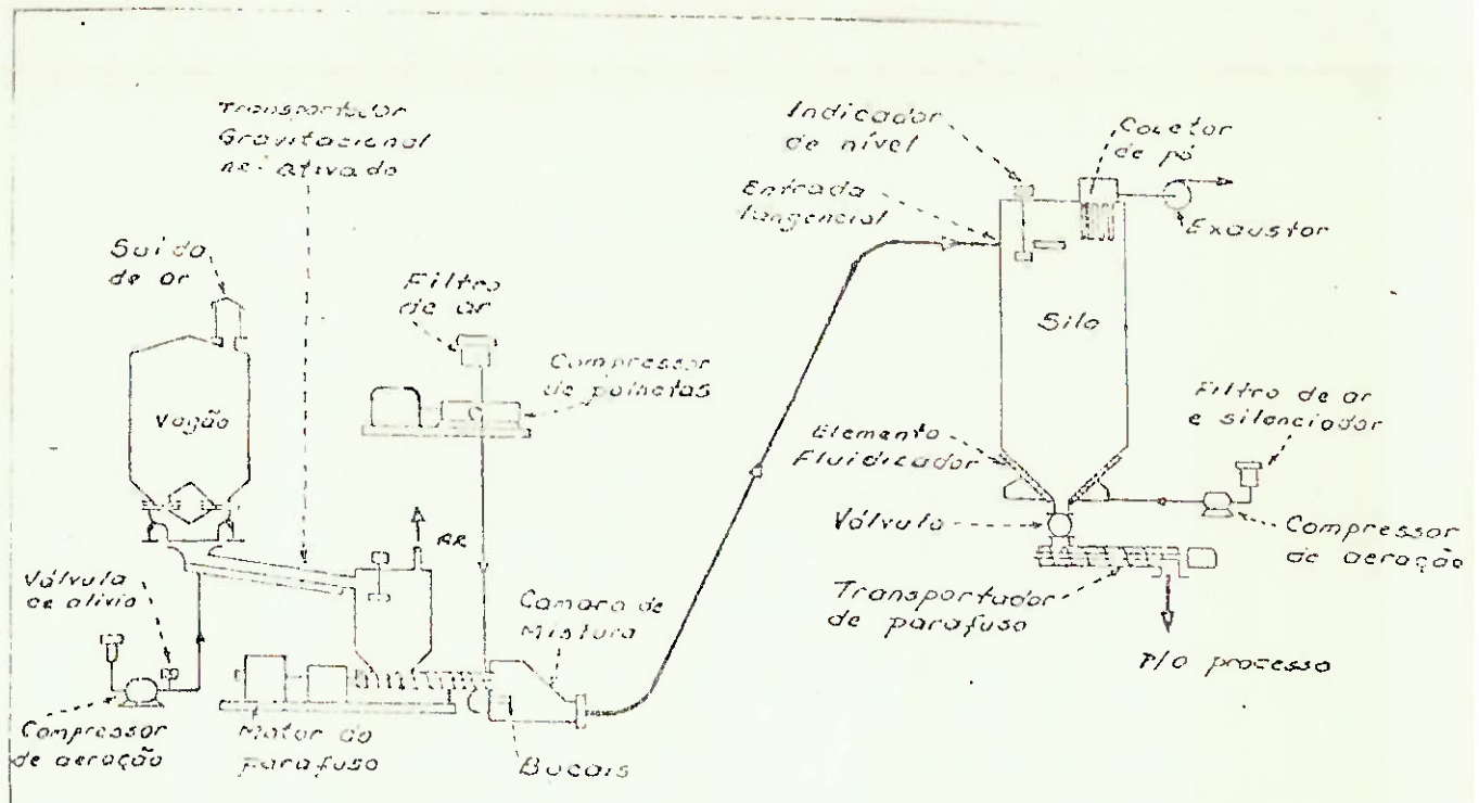
Fig.II.10 - Sistema com câmara de mistura.
