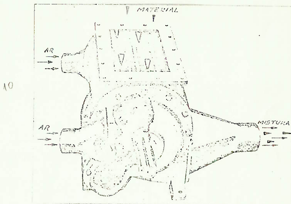
Fig.II.9 - Vista interior de um alimentador rotativo de duas entradas.
