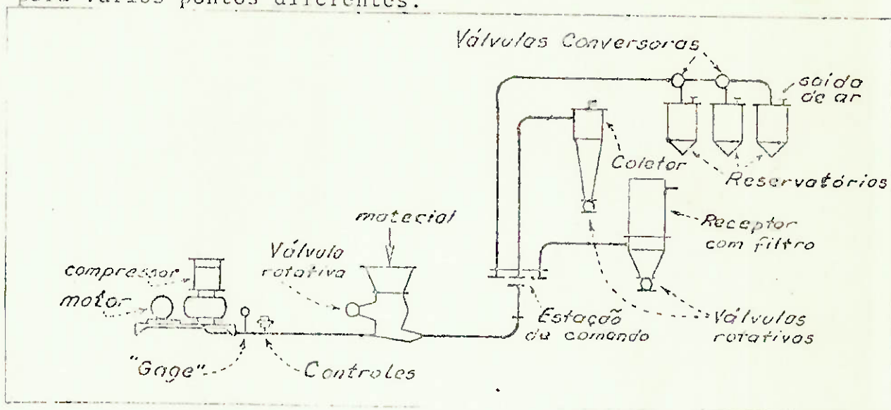
Fig.II.2 - Sistema de pressão positiva.
