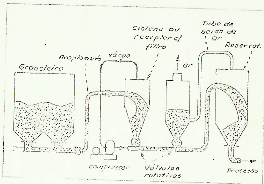
Fig.II.4 - Sistema combinado vácuo-pressão.
