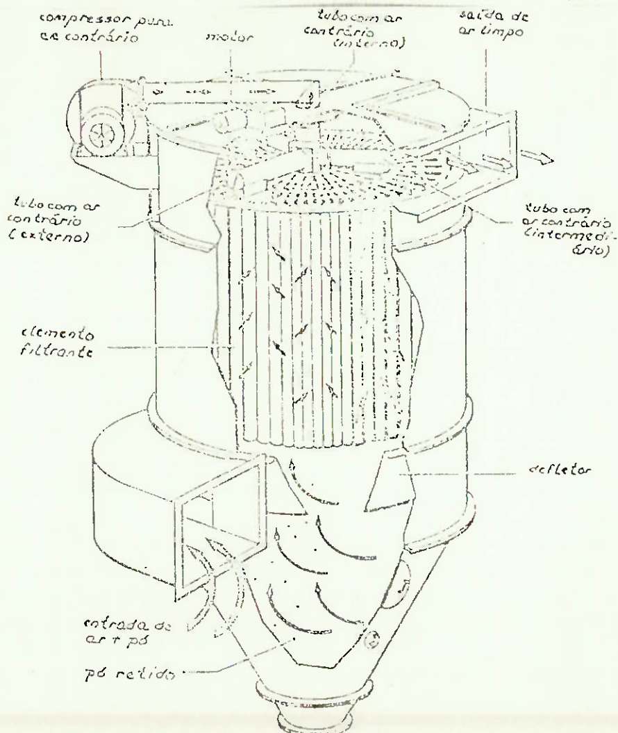
Fig.IV.23- Filtro de pó com ar contrário a baixa pressão com "plenum" rotativo.
