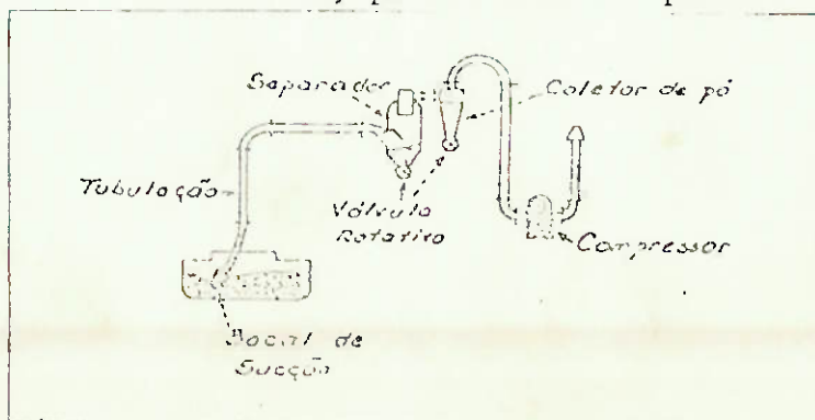
Fig.II.1.b- Sistema de vácuo c/bocal de sucção.
